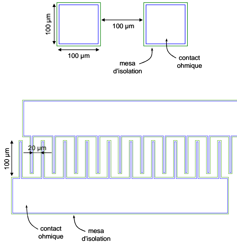
Figure A-17 : motifs d'isolation utilisés sur nos échantillons pour la mesure de la résistance des couches tampon R_{tampon}
