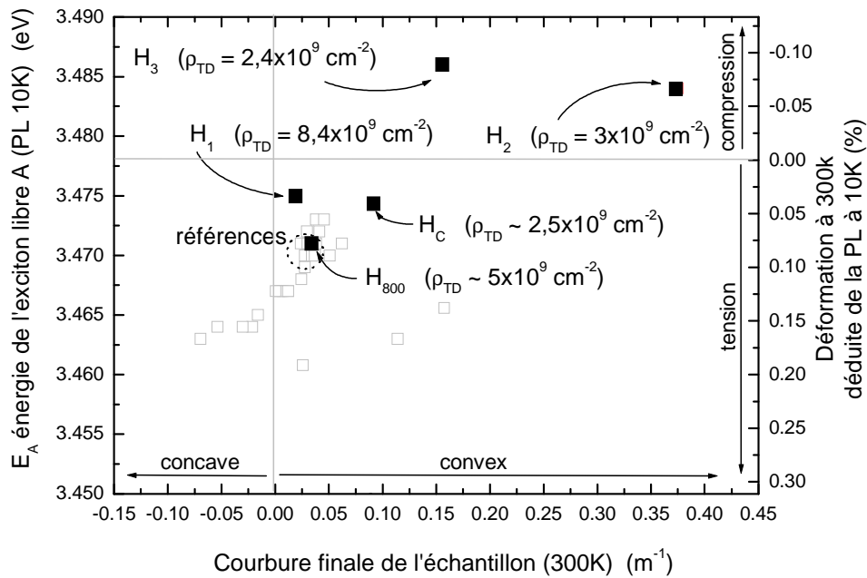
Figure III-36 : énergie de l'exciton libre A du GaN ( E_A ) mesurée par photoluminescence à basse température (PL 10K) et la déformation biaxiale ( \epsilon_{xx} ) déduite à température ambiante (300K) selon l'équation I-18 (Chapitre I), en fonction de la courbure finale de l'échantillon mesurée à température ambiante (300K). Les densités de dislocations ( \rho_{TD} ) données ont été mesurées par MFA
