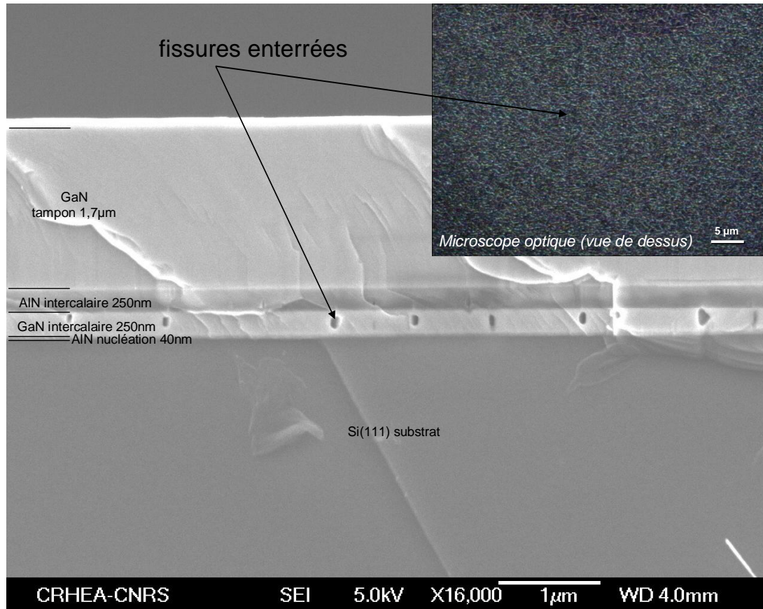
Figure III-25 : image MEB de la section d'une structure HEMT (Al,Ga)N/GaN « standard » sur substrat Si(111). En insert est présentée le réseau de fissures enterrées vue de dessus par microscopie optique (champ sombre)
