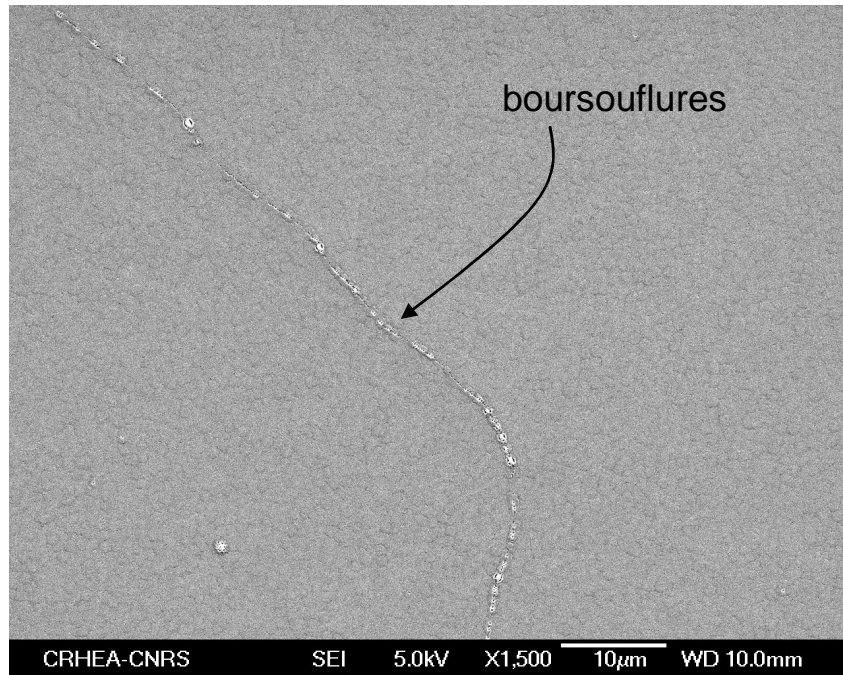
Figure III-31 : image MEB de la surface d'une couche tampon GaN épitaxiée sur un empilement \text{AlN}_{350\text{nm}}/\text{GaN}_{250\text{nm}}/\text{AlN}_{40\text{nm}} sur substrat Si(111) désoxydé thermiquement in situ
