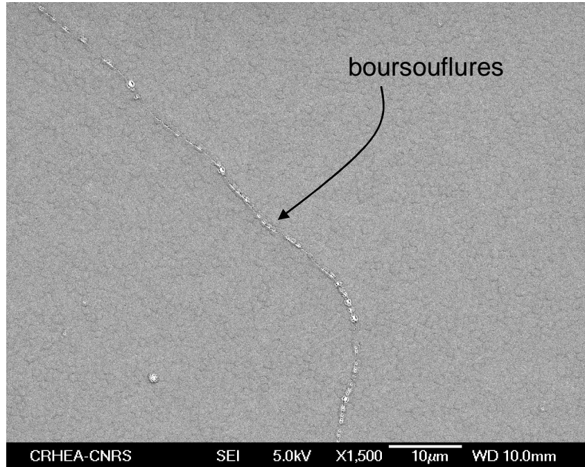
Figure III-31 : image MEB de la surface d'une couche tampon GaN épitaxiée sur un empilement \text{AlN}_{350\text{nm}}/\text{GaN}_{250\text{nm}}/\text{AlN}_{40\text{nm}} sur substrat Si(111) désoxydé thermiquement in situ
