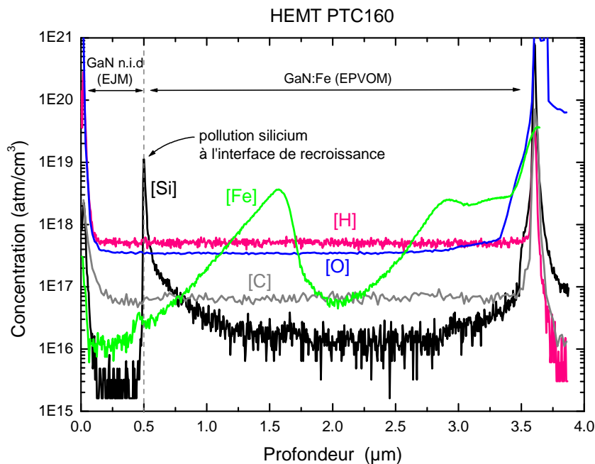
Figure IV-2 : profil SIMS montrant les contaminants et le Fer dans la structure HEMT PTC160 (reprise de croissance sur trempin GaN:Fe/Saphir classique)
