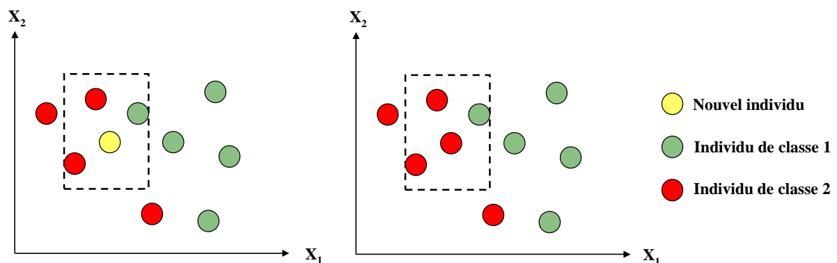
FIG. 2.1 : Principe des K plus proches voisins
