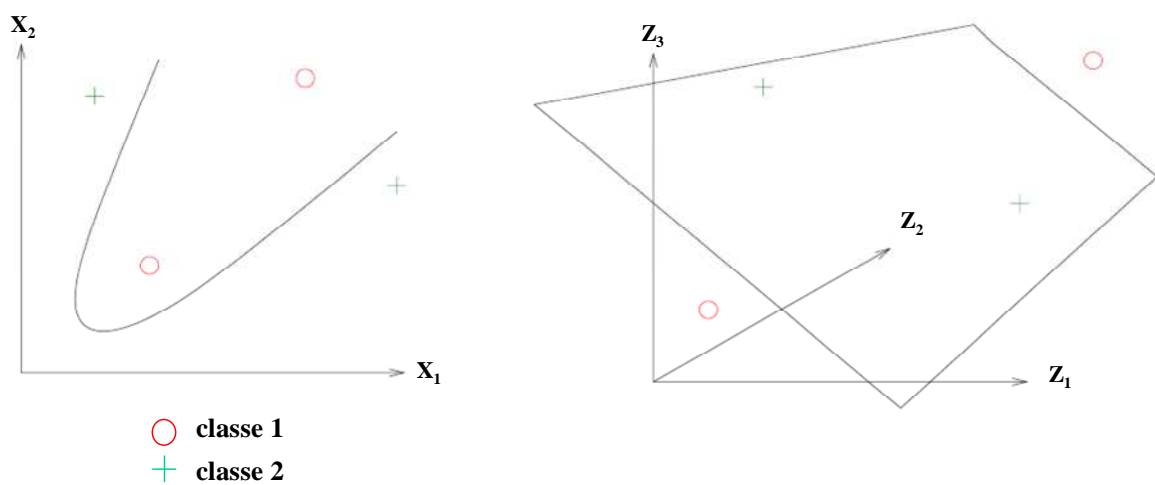
FIG. 2.6 : Exemple de SVM non linéaire [46]
