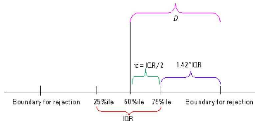
FIG. B.3 : Interquartile Range
