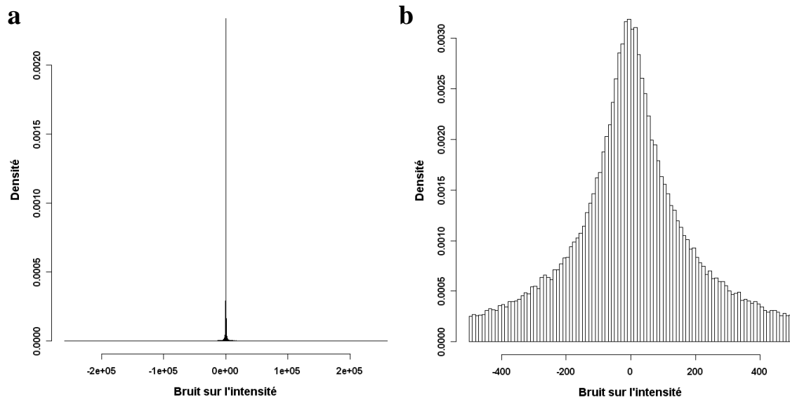
FIG. C.4 : Histogrammes du bruit sur l'intensité
