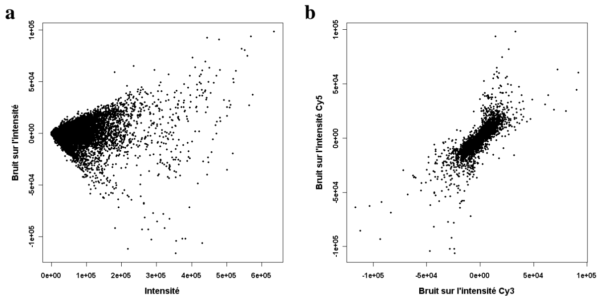
FIG. 3.7 : Propriétés du bruit sur l'intensité
