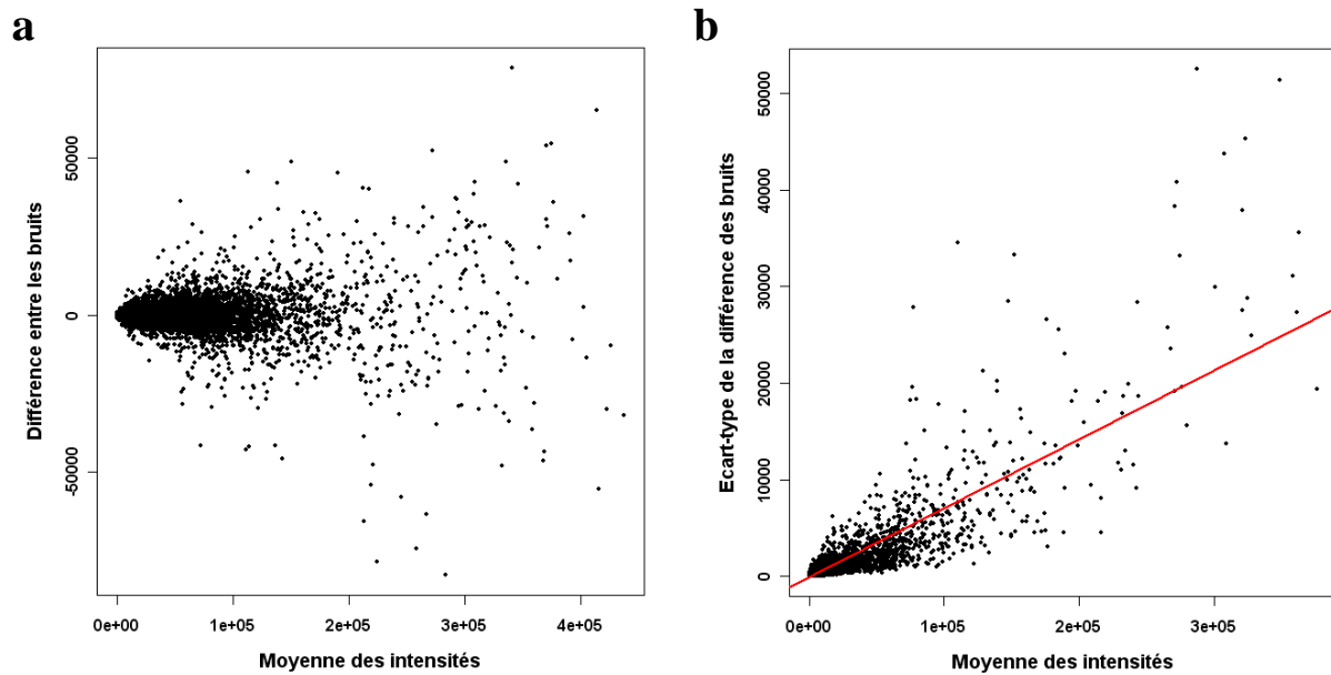
FIG. 3.12 : Étude de la différence entre bruit sur l'intensité Cy5 et bruit sur l'intensité Cy3 (a) : Différence entre les bruits sur les intensités Cy5 et Cy3 en fonction de la moyenne des intensités Cy5 et Cy3. (b) : Écart type de la différence entre les bruits sur les intensités Cy5 et Cy3 en fonction de la moyenne des intensités Cy5 et Cy3.
