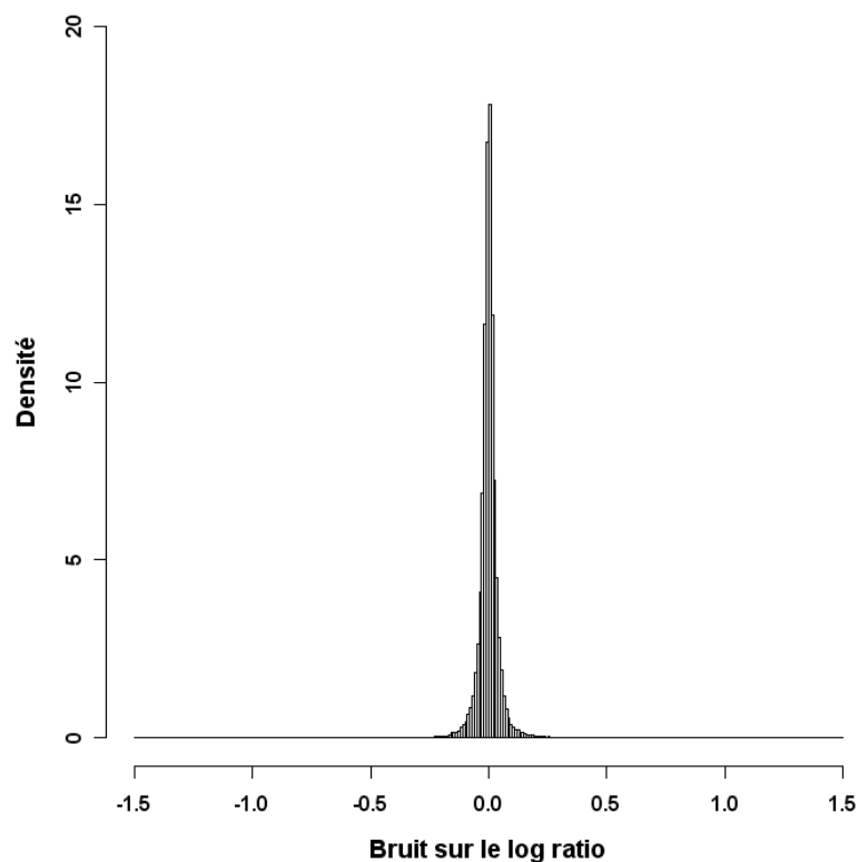
FIG. C.2 : Histogramme du bruit sur le log ratio
