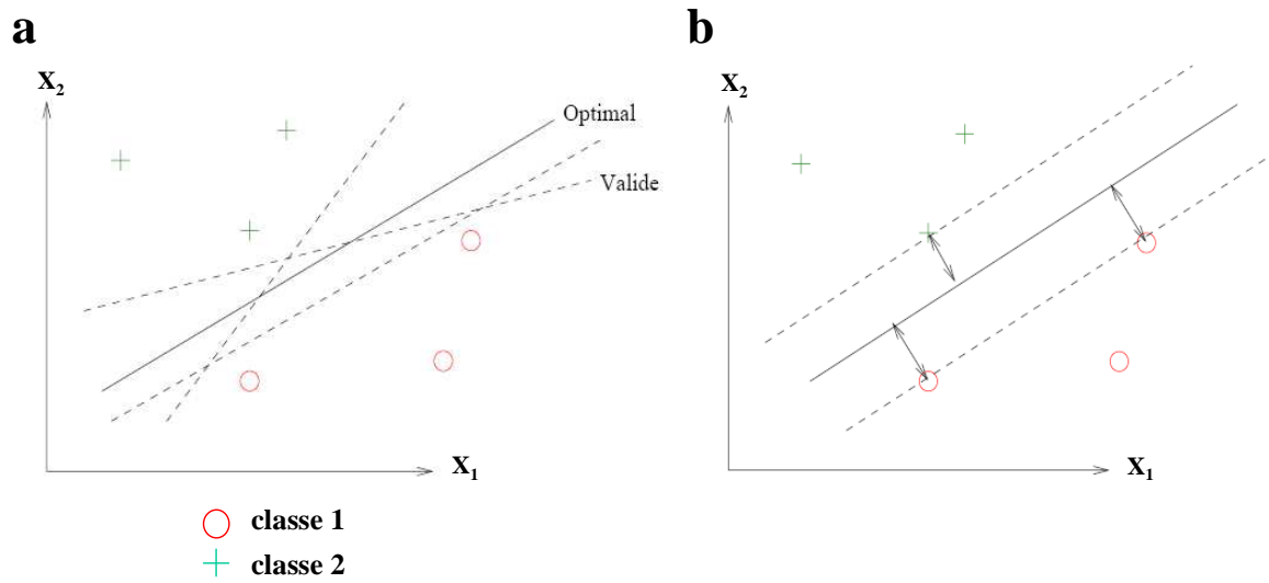
FIG. 2.5 : Principe des SVMs linéaires [46]
