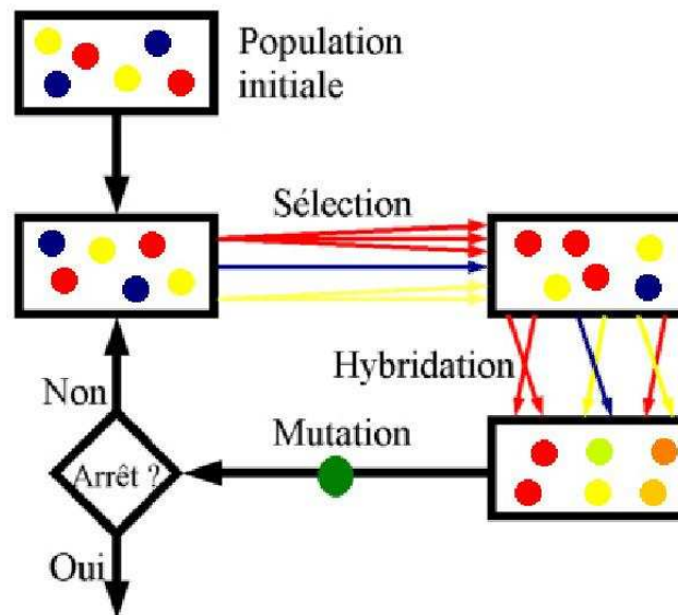
FIG. 2.9 : Principe des algorithmes génétiques [56]
