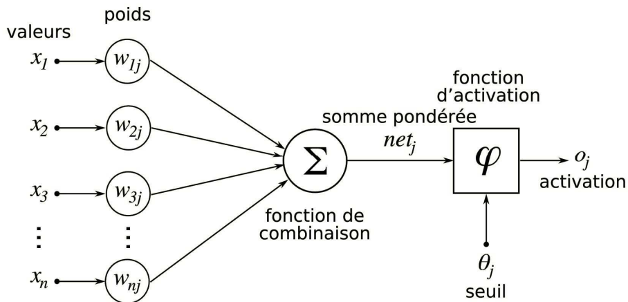
FIG. 2.3 : Unité de calcul [44]
