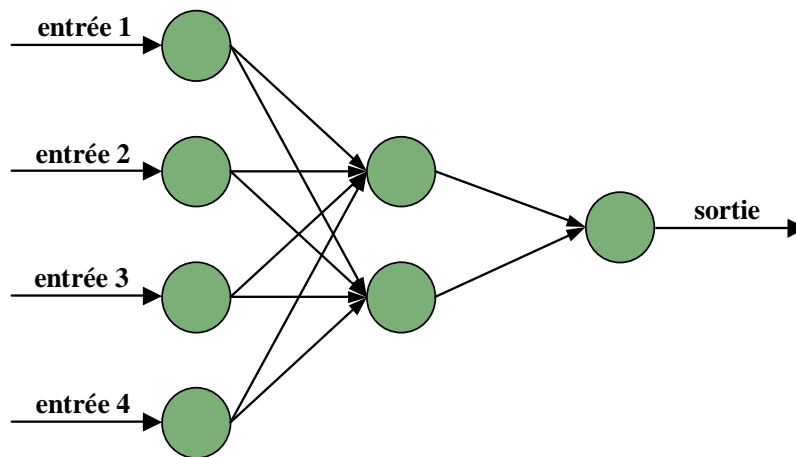
FIG. 2.4 : Perceptron multicouche
