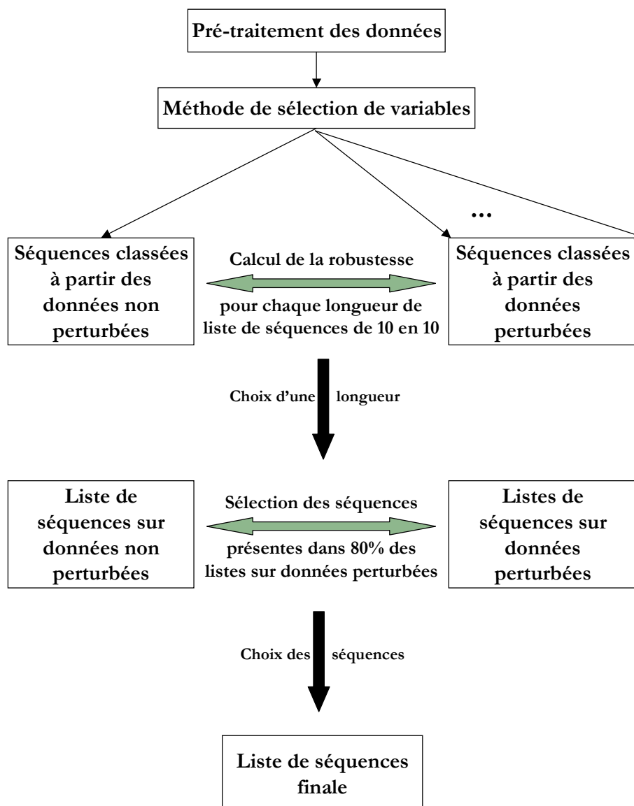
FIG. 3.2 : Principe de MetRob
