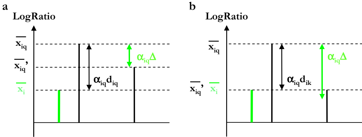
FIG. 2.7 : Principe de la méthode de Nearest Shrunken Centroids
