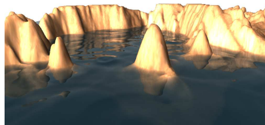
FIG. 6.4 Réflexions sur une surface d'eau.
