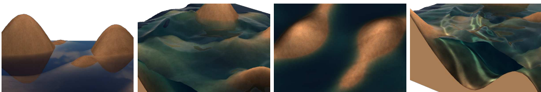
FIGURE 6.3 – Les quatre phénomènes lumineux importants à calculer dans un volume d'eau : (a) réflexion, (b) réfraction, (c) absorption, (d) caustiques.
