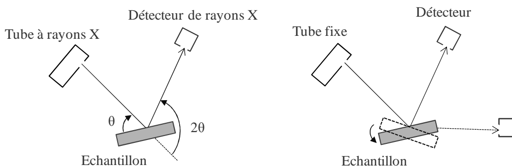
Figure 4 : Schéma de principe du montage en \theta - 2\theta .
