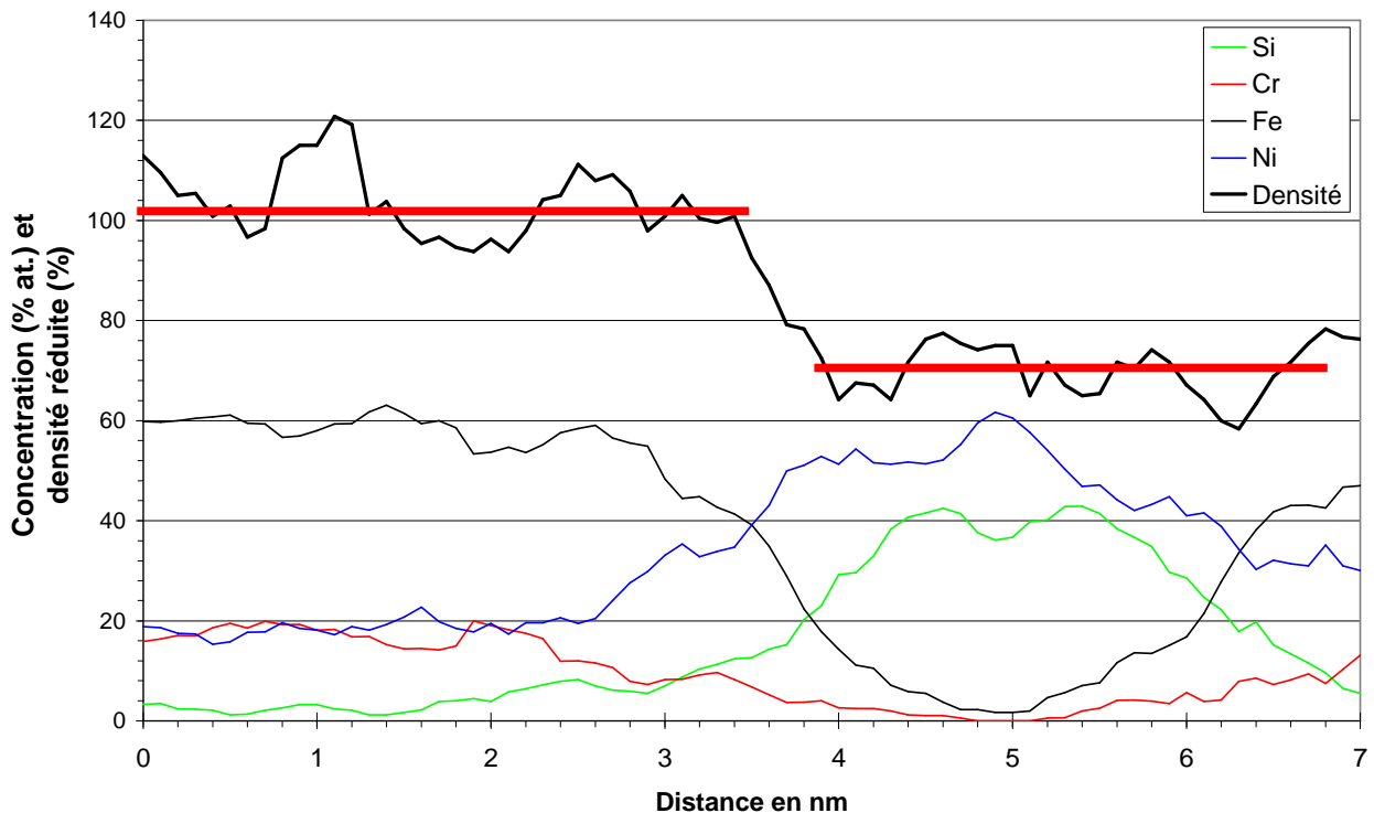
Figure 3 : Profil de concentration et profil de densité réduite au travers un amas Ni-Si.
