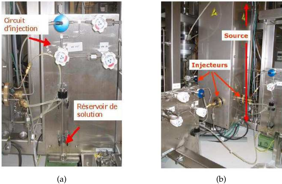
FIG. 2.11 – (a) et (b) Photos du dispositif d'injection.
