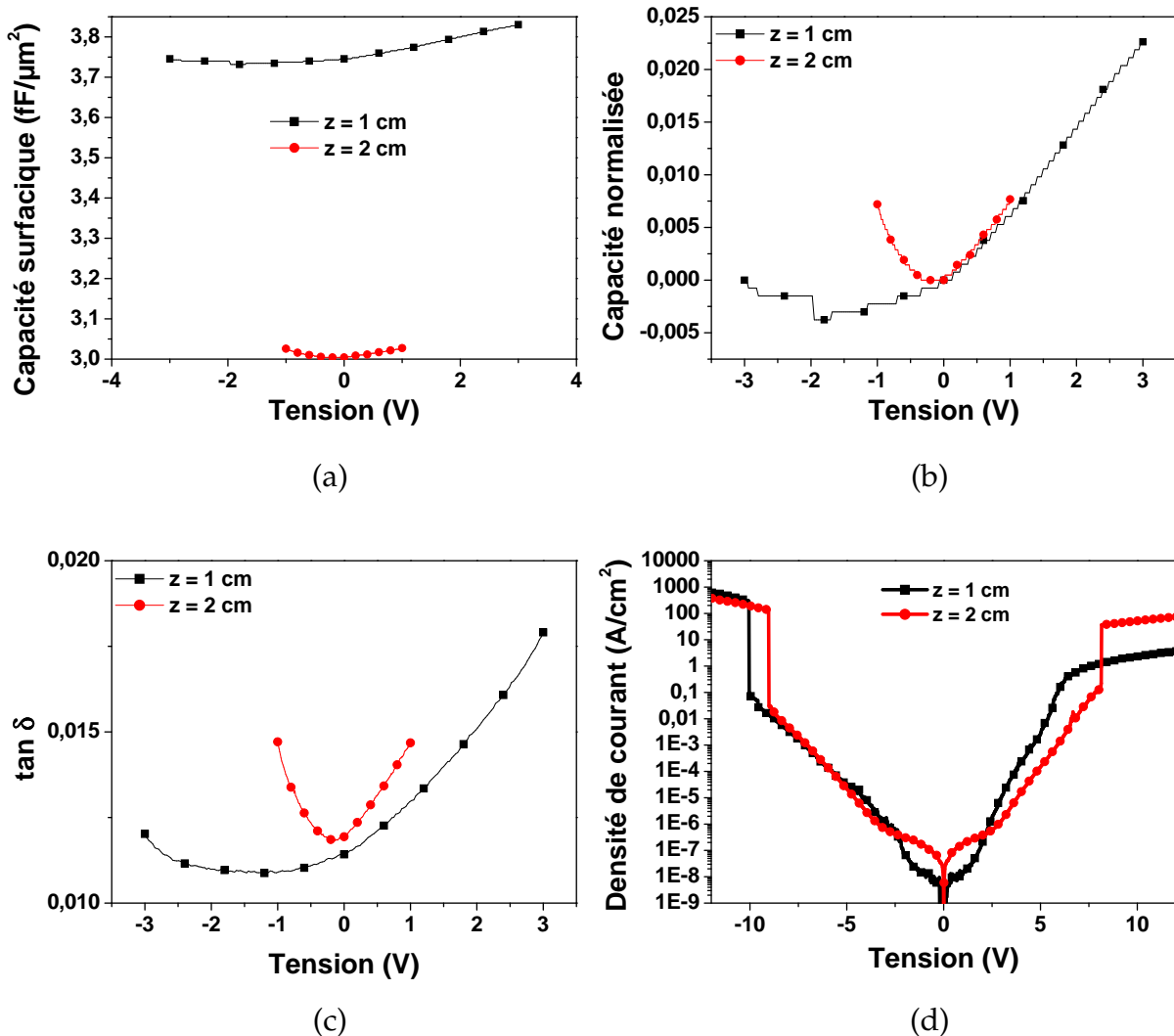
FIG. 3.21 – Caractérisations de la capacité surfacique en fonction de la tension (a), de la capacité normalisée en fonction de la tension (b), des pertes diélectrique en fonction de la tension (c) et des densités de courant en fonction de la tension (d) pour des dépôts d'oxyde d'yttrium élaborés par MOCVD avec une assistance plasma RF avec deux distances inter-électrodes 1 cm et 2 cm.
