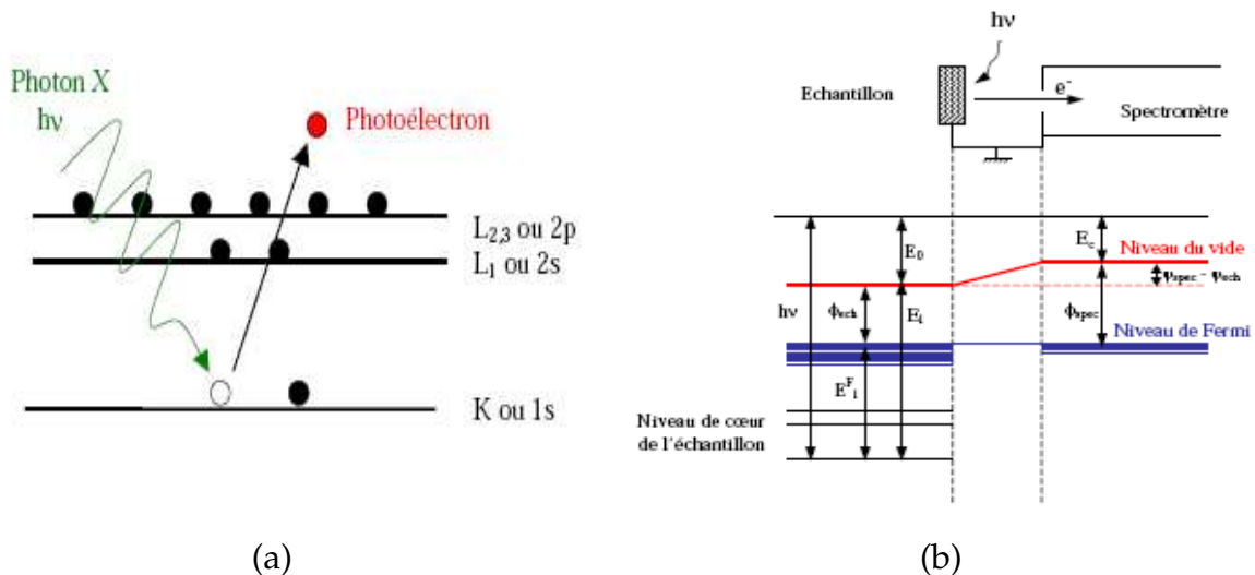
FIG. 2.19 – Phénomène de photo-émission. (a) Principe de photo-excitation sous l'effet d'un rayonnement X. (b) Diagramme énergétique du processus de photoémission pour un échantillon métallique.
