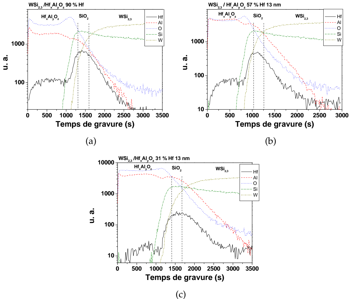
FIG. 5.20 – Spectres SIMS pour les échantillons intermixées avec 90 % (a), 57 % et 31 % de \text{HfO}_2 .
