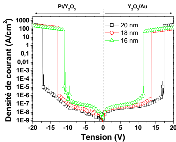
FIG. 4.18 – Courbes représentant les densités de courant en fonction de la tension concernant les dépôts de Y_2O_3 sur platine.
