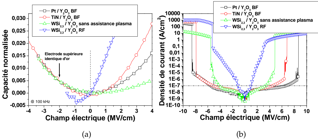
FIG. 3.28 – Comparaison de la capacité normalisée (a) et des densités de courant de fuite (b) en fonction du champ électrique pour des échantillons élaborés sur le réacteur PLANAR 200 BF sur nitrure de titane et platine, par MOCVD sans assistance plasma sur siliciure de tungstène et par MOCVD avec une assistance plasma RF sur siliciure de tungstène.
