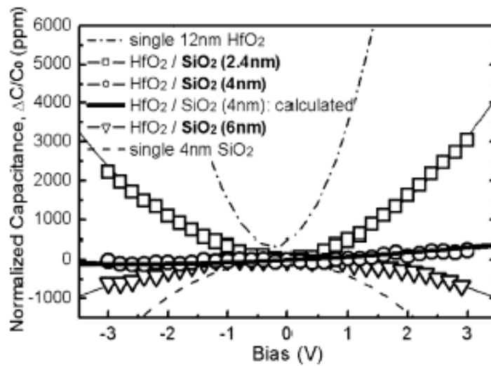
FIG. 1.14 – Amélioration de la linéarité en intercalant une couche de SiO 2 à courbure négative entre le substrat et la couche de HfO 2 .
