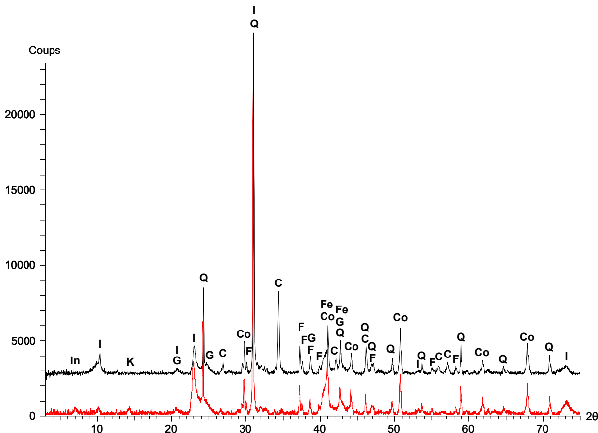
Figure 7. Diagrammes DRX de l'horizon C3 (en rouge) et du résidu de décarbonatation de l'échantillon calcaire L1 de la Terre-Plaine (en noir) au contact de l'horizon C3. Les pics principaux des différents minéraux identifiés sont annotés selon la nomenclature suivante : Q = quartz, F = (fluor)apatite, G = goéthite, Fe = ferrihydrite, B = birnessite, I = illite, K = kaolinite, In = argiles interstratifiées, C = calcite et Co = corindon (ayant servi au dopage des échantillons).
