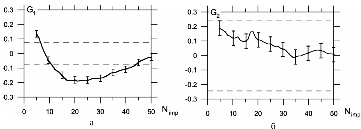
Рис. 2.4. Залежності параметрів G_1 (а) та G_2 (б) від ефективної кількості областей (імпульсів) з додатнім інкрементом. Для нормального розподілу G_1 та G_2 мають дорівнювати нулю; горизонтальні лінії показують відповідні пороги статистичної значущості відхилення.
