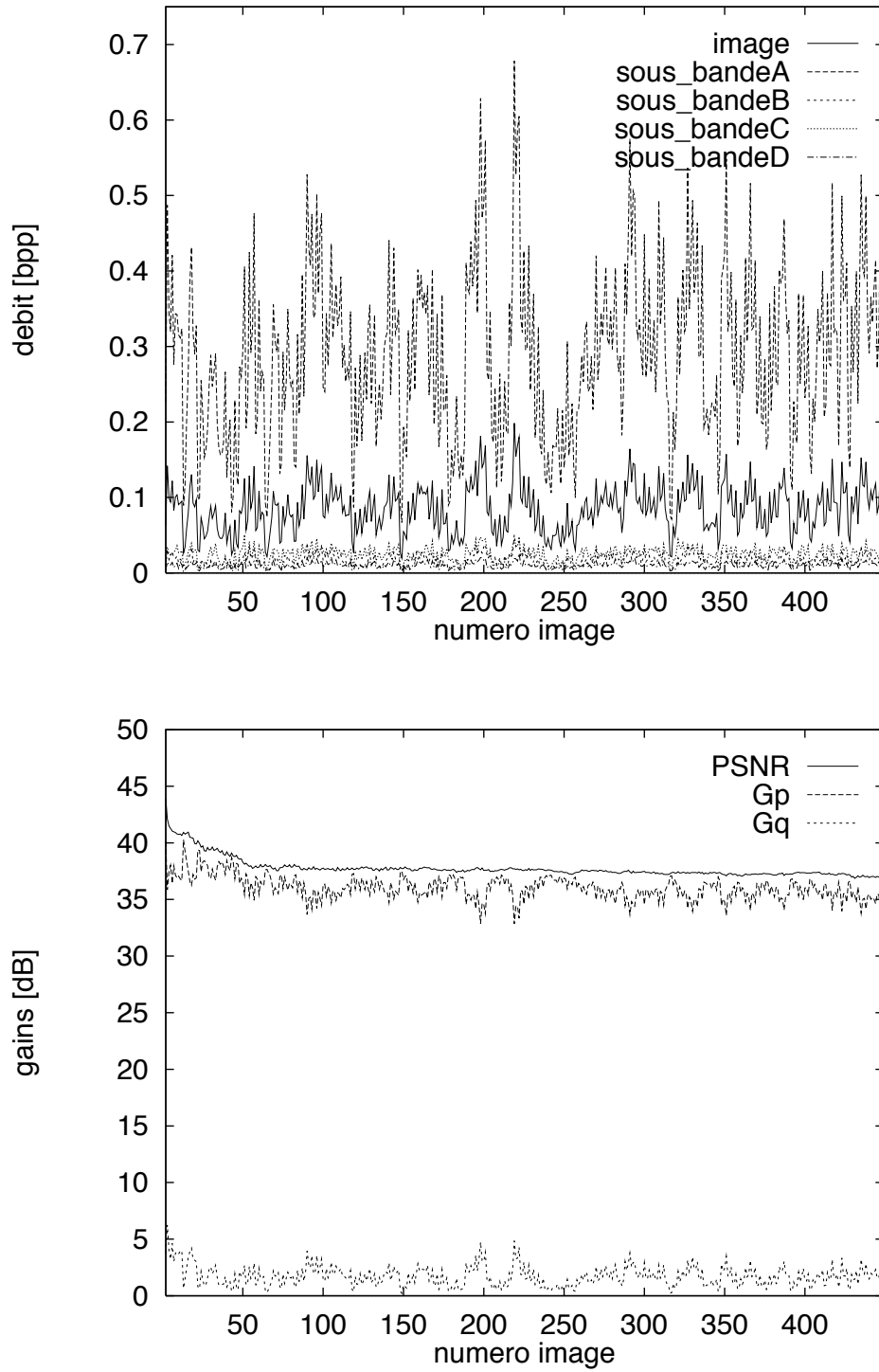
FIG. 6.11 – Codeur type MPEG, allocation à 0,2 bpp, encodage de 450 images de Claire : entropies et gains des images.
