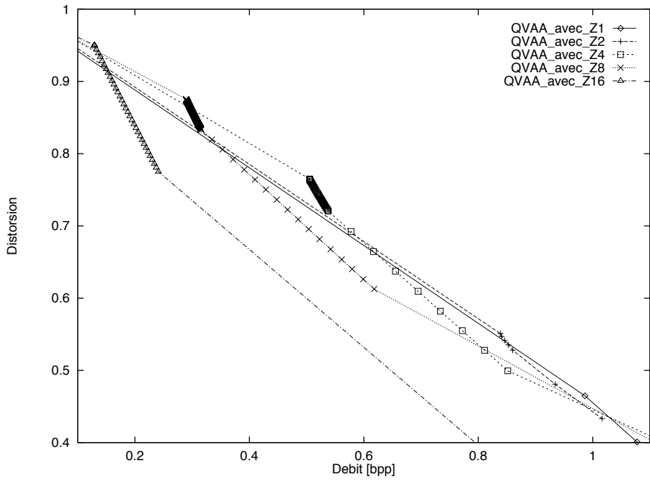
FIG. 5.15 – Courbes débit vs. distorsion (entropie du dictionnaire vs. distorsion) obtenues par découpage du dictionnaire arborescent et mettant en jeu différents réseaux. La source i.i.d obéit à une loi normale ( \sigma^2 = 1 ).
