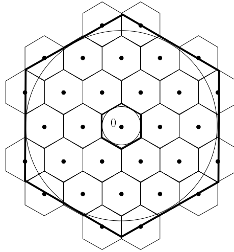
FIG. 5.6 – Un emboîtement sous-optimal avec le réseau hexagonal ( b = 5 ).
