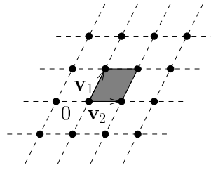
FIG. 3.1 – Un réseau bidimensionnel et son parallélotope associé.
