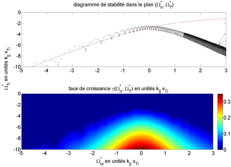
FIGURE 2.6 – Seuil de stabilité linéaire et taux de croissance d’instabilité dans le cas d’un équilibre Lorentzien, comparé au cas d’un équilibre maxwellien (trait continu). N = 100 bags, a_{100} = 10v_{Ti} , Z_i^* = 1 .
