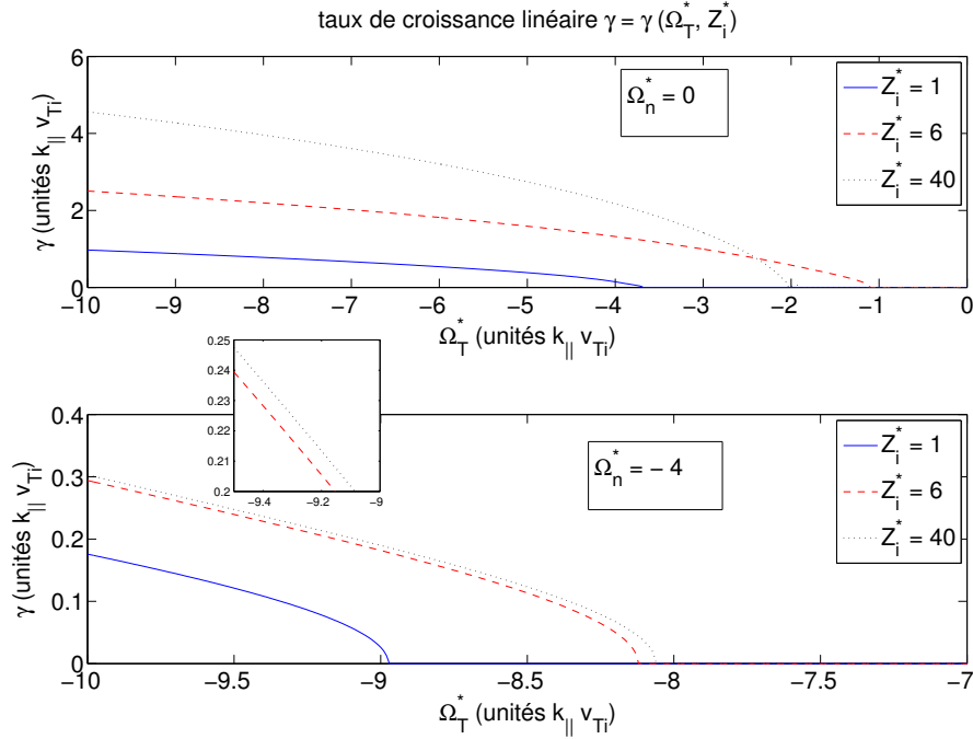
FIGURE 2.5 – Influence du paramètre Z_i^* sur les valeurs du taux de croissance d'instabilité en fonction de \Omega_T^* , pour deux valeurs du gradient de densité ( \Omega_n^* = 0k_{\parallel}v_{Ti} et -4k_{\parallel}v_{Ti} ).
