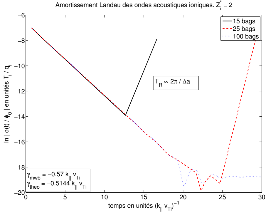
FIGURE 1.5 – Amortissement Landau linéaire : évolution temporelle du potentiel électrostatique, pour différents nombres de bags (échelle logarithmique).
