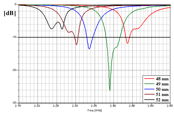
Figure 3.46: Coefficient de réflexion en fonction de la fréquence pour différentes valeurs de a_3
