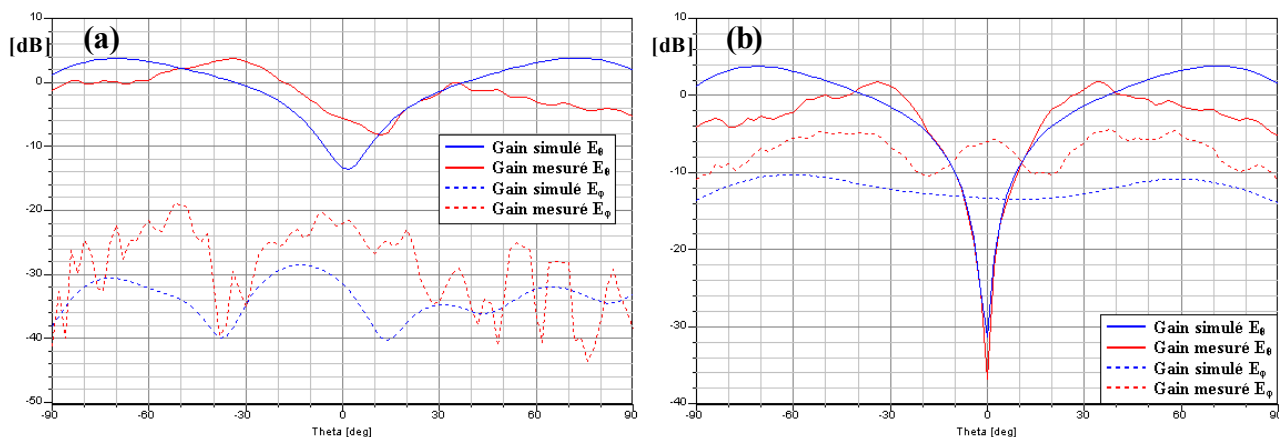
Figure I.20: Gains E_\theta et E_\phi simulé à 5,59 GHz et mesuré à 5,655 GHz (a) plan x-z (b) plan y-z
