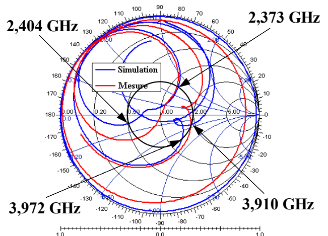
Figure 3.54: Impédance d'entrée
