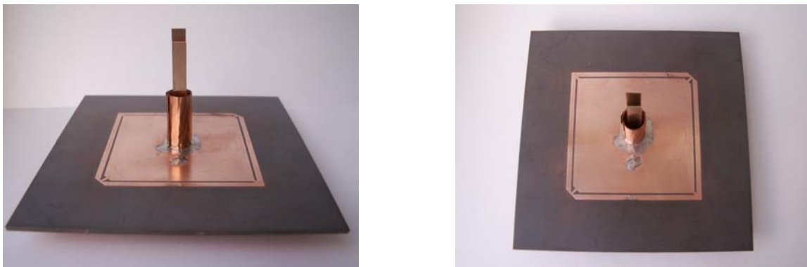
Figure 4.22: Photos de l'antenne combinée N°1
