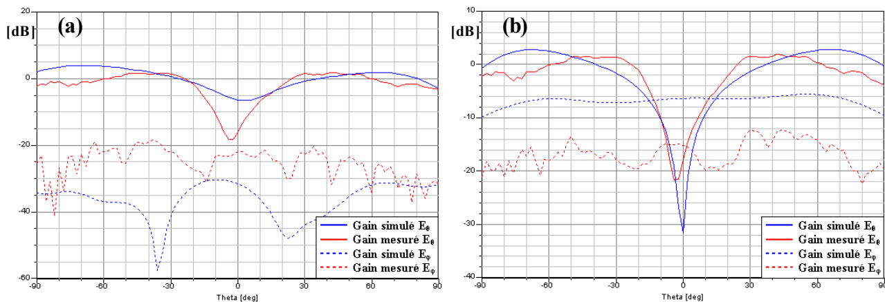
Figure I.19: Gains E_\theta et E_\phi simulé à 5,31 GHz et mesuré à 5,34 GHz (a) plan x-z (b) plan y-z
