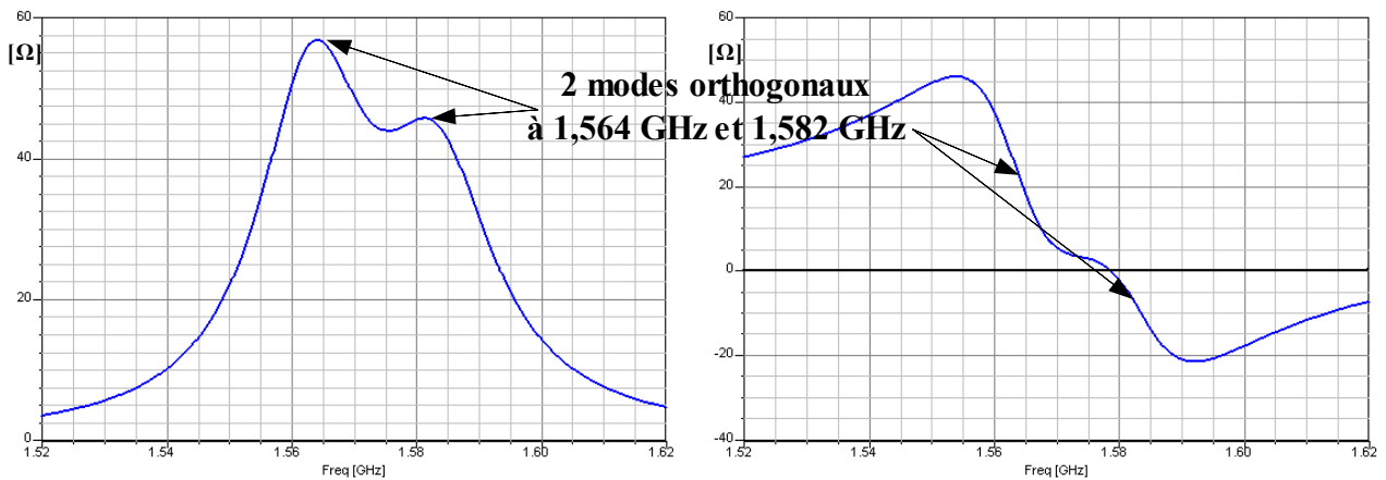
Figure 3.23: Parties réelle et imaginaire de l'impédance d'entrée
