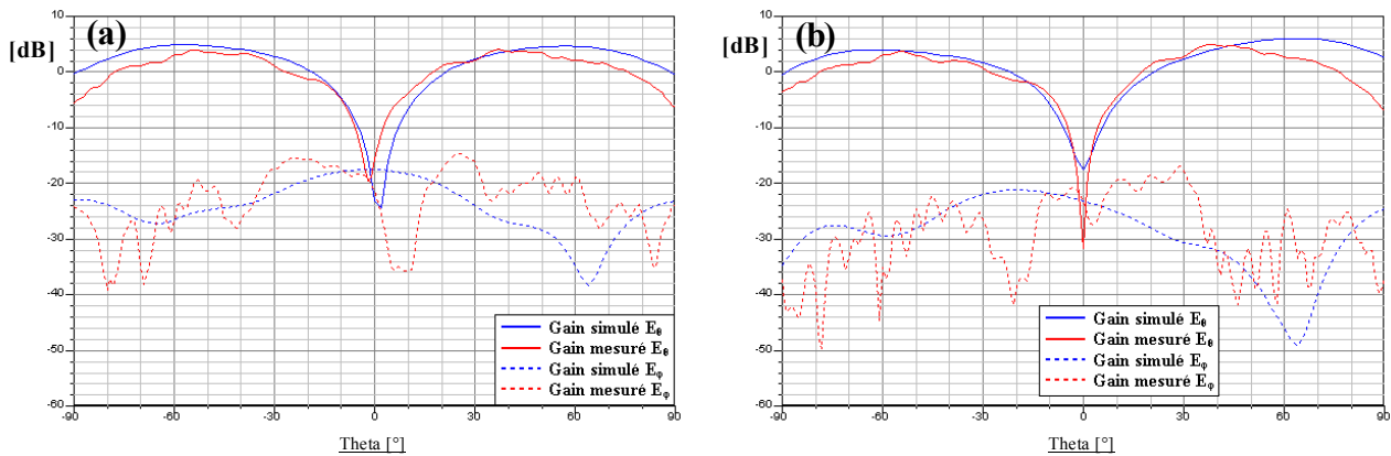
Figure 2.27: Gains E_0 et E_\phi simulé à 5,55 GHz et mesuré à 5,59 GHz
