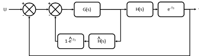
FIGURE 4.11 – Prédicteur de Smith, inspiré de Smith, 1959. Le procédé piloté est dissocié de son retard pur. Le prédicteur dispose d'un modèle interne du procédé sans retard \widehat{H}(s) ainsi que du retard pur lui-même e^{-\widehat{T}.s} . Le comportement de ce système est alors équivalent à une régulation de H(s) par G(s) en boucle fermée. La sortie de H(s) étant par la suite retardée de T .
