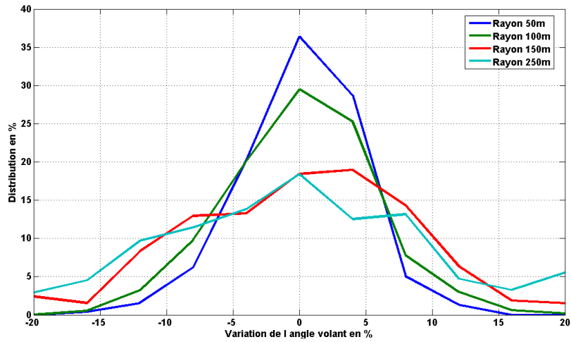
FIGURE 9.8 – Distribution de la variation relative de l'angle volant lors de conduites à la vitesse de 70\text{km/h} autour de cercles de 50, 100, 150 et 250m de rayons.
