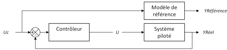
FIGURE 6.6 – Schéma block de principe d'un contrôleur par modèle de référence (MRC). L'objectif de cette technique est de proposer un paramétrage du contrôle pour que le comportement en boucle fermée de l'ensemble coïncide avec celui issu du modèle de référence et ce quelque soit le signal de consigne. Un point délicat de cette technique est la parfaite connaissance des caractéristiques du système piloté.
