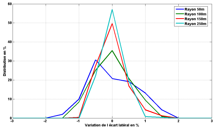
FIGURE 9.9 – Distribution de la variation relative de l'écart latéral du véhicule lors de conduites à la vitesse de 70\text{km/h} autour de cercles de 50, 100, 150 et 250m de rayons.
