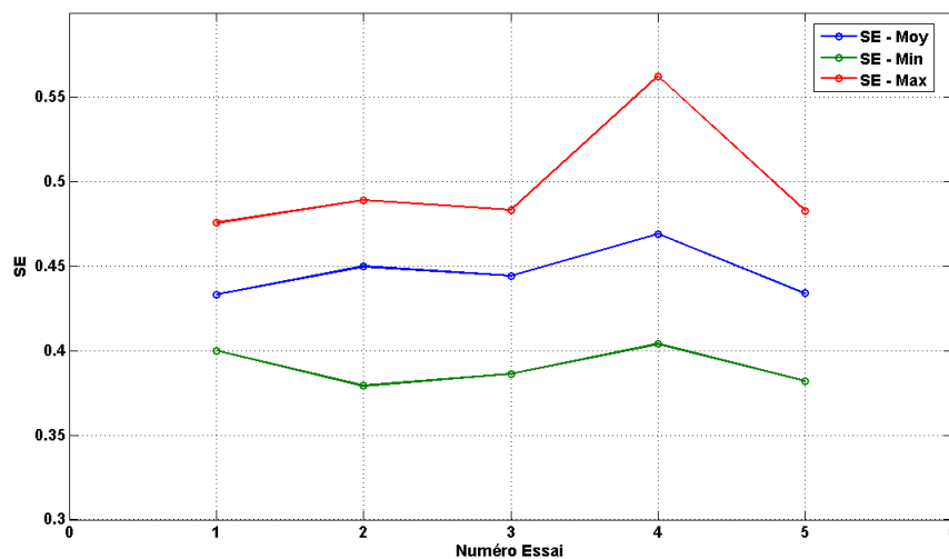
FIGURE 10.15 – Evolution du SE moyen entre les différents conducteurs. Pour près de 60% d'entre eux, l'événement volant provoque une augmentation systématique du critère alors que pour les autres celui-ci diminue.
