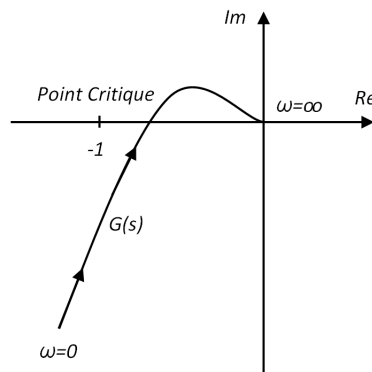
FIGURE A.2 – Illustration du critère du revers. Le système en boucle fermée est stable si en parcourant le lieu de transfert (dans le plan de Nyquist) du système en boucle ouverte dans le sens croissant des fréquences, le point critique -1 est laissé sur la gauche comme sur le schéma ci-dessus.
