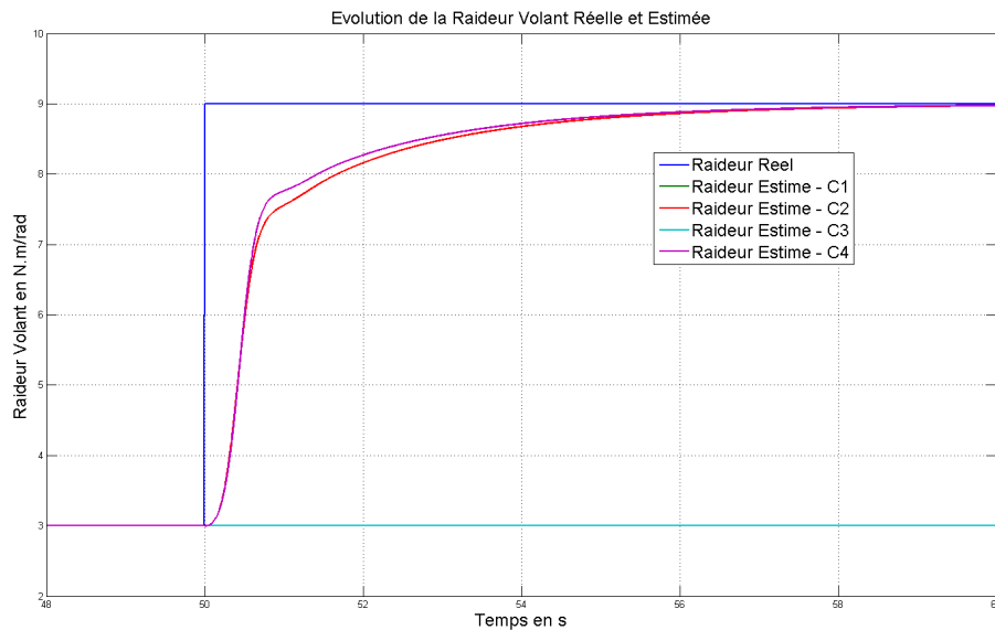
FIGURE 8.6 – Evolution de la raideur du système volant ainsi que de sa représentation interne dans le module de poursuite du modèle de conducteur. Modification du véhicule à t = 50s .
