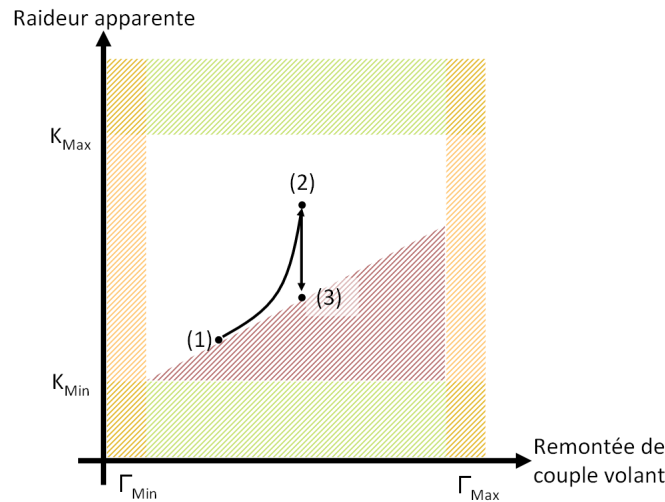
FIGURE 8.5 – Exemple de comportement de la stratégie de modulation d'impédance lors d'une élévation de couple au niveau du volant. Les différentes étapes d'évolution du niveau d'impédance sont matérialisées par les états (1), (2) et (3). Les parties hachurées en vert décrivent les zones physiologiquement impossibles à atteindre. Celles en orange représentent la gamme de couple remontée au niveau du volant et par extension, la plage de valeurs du couple de poursuite. Enfin, la zone hachurée en rouge rend compte de l'évolution de l'impédance minimale du conducteur selon le niveau de couple qu'il produit et donc le niveau d'activation de ses muscles.
