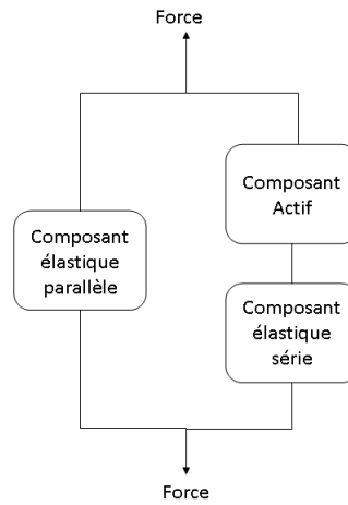
FIGURE 3.9 – Forme générale du modèle de Hill. Les composants élastiques peuvent intégrer les propriétés visqueuses des muscles.
