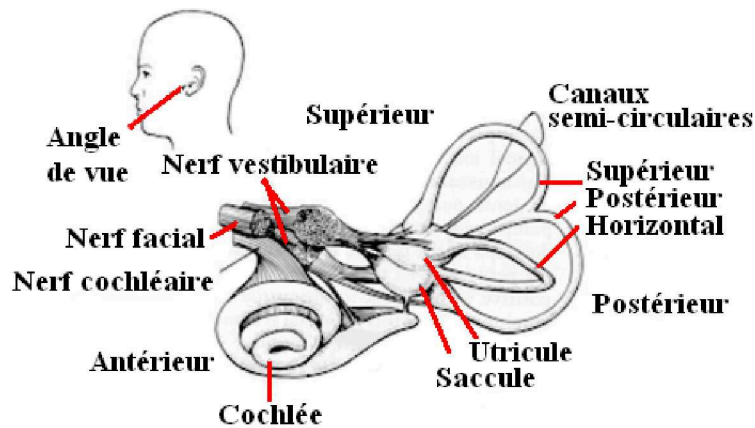
FIGURE 3.5 – D'après Blouin, 2004. L'appareil vestibulaire est permet entre autre la détection de rotations via les canaux semi-circulaires et d'accélération linéaires au niveau des otolithes.
