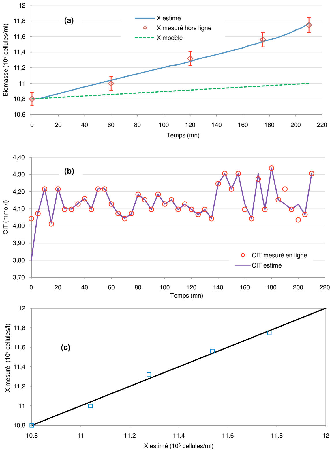
Figure 5.20 : Comparaison entre des mesures directes ( \diamond , \circ ) et les prédictions ( \text{---} ) du filtre de Kalman étendu reposant sur les mesures du CIT : (a) biomasse mesuré par granulométrie (b) concentration en carbone inorganique total, (c) validation de la relation linéaire liant X estimé et X mesuré.
