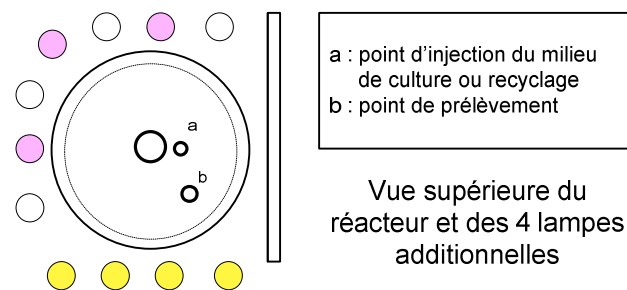
Figure 2.9 : Vue supérieure du photobioréacteur et de leur système d'illumination modifié
