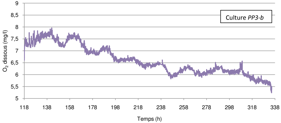
Figure C.8 : Evolution temporelle de la concentration en oxygène dissous.
