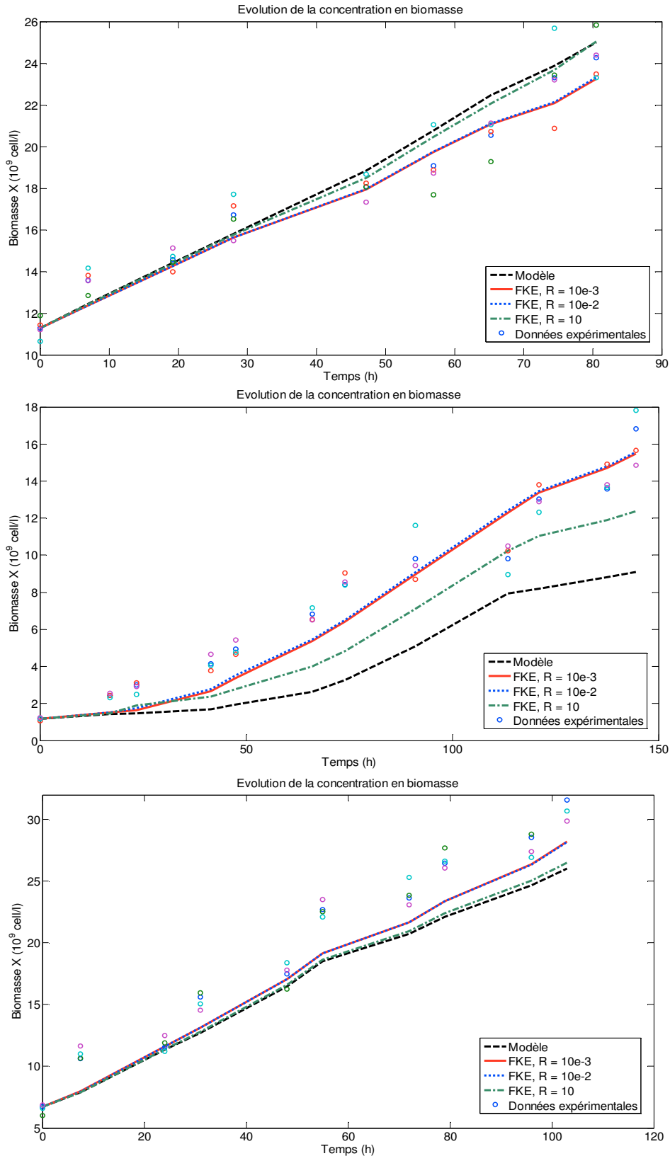
Figure 3.14 : Etude de l'effet de la matrice de covariance R sur l'estimation de la concentration en biomasse dans des cultures batch de Porphyridium purpureum à (a) 1% de \text{CO}_2 dans le gaz d'alimentation, (b) intensité lumineuse faible et (c) intensité lumineuse élevée.
