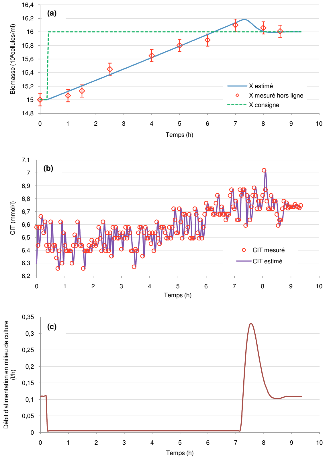
Figure 5.27 : Commande linéarisante y = X avec antiwindup ( K_s=0,5 ), comportement du système pour un échelon sur la consigne : passage de 15 à 16 \cdot 10^6 cellules/ml à t=0,25 h
