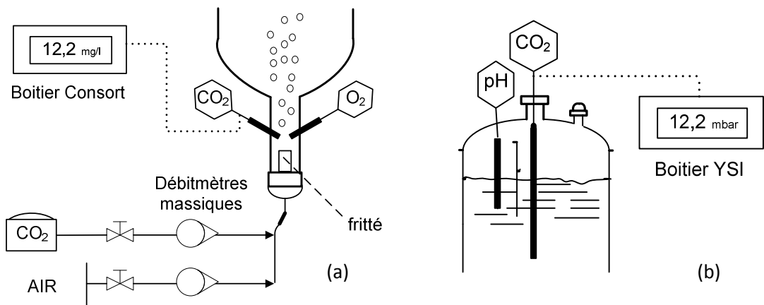
Fig. 5.14 : Configurations originale (a) et finale (b) de positionnement de la sonde à CO 2 sur le réacteur.
