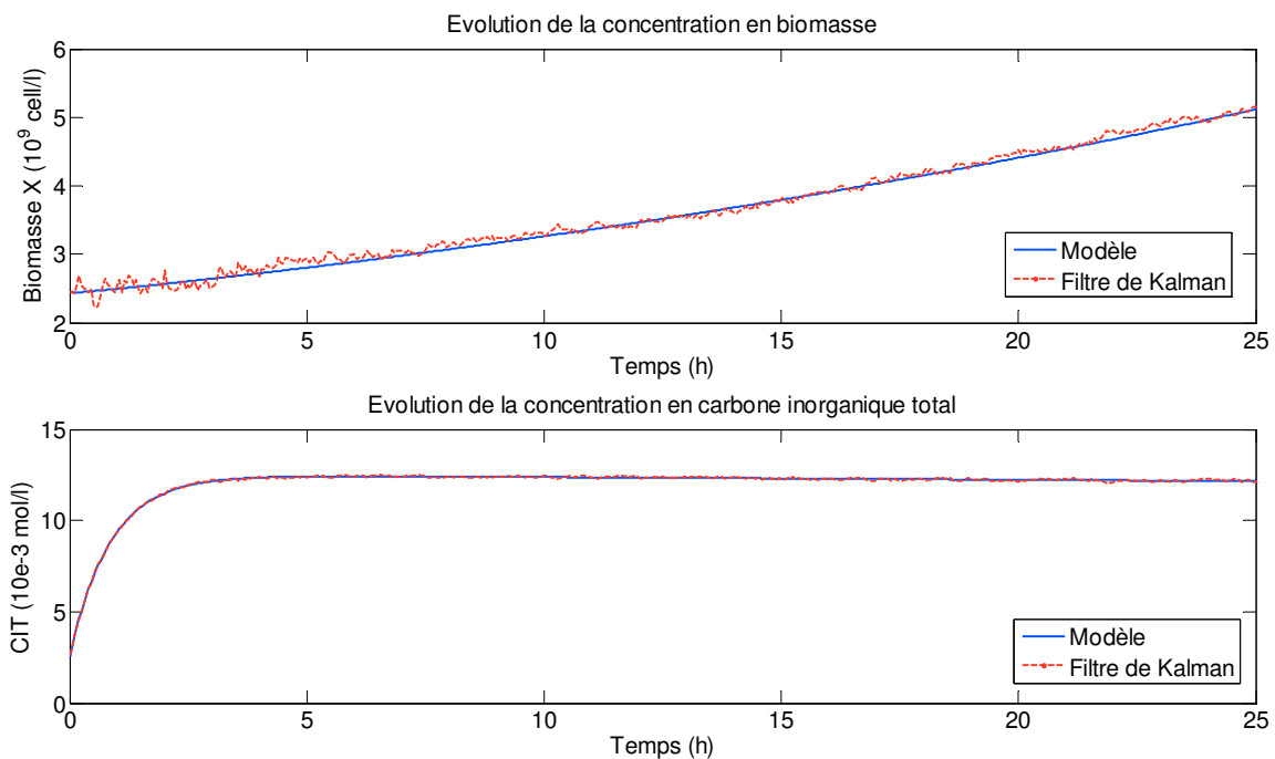
Figure 3.4 : Estimation de la concentration en biomasse et de la concentration en carbone inorganique total. Erreur de 3% sur la valeur initiale de CIT
