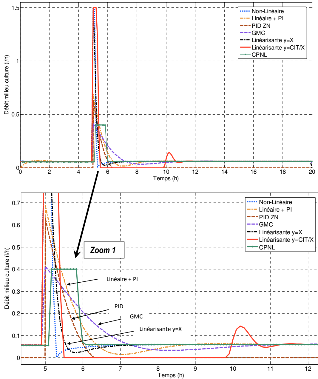
Figure 4.15 : Evolution des débits d'alimentation dans le photobioréacteur pour un échelon sur la consigne (passage de 10 à 9. 10 9 cellules/l à t = 5h).
