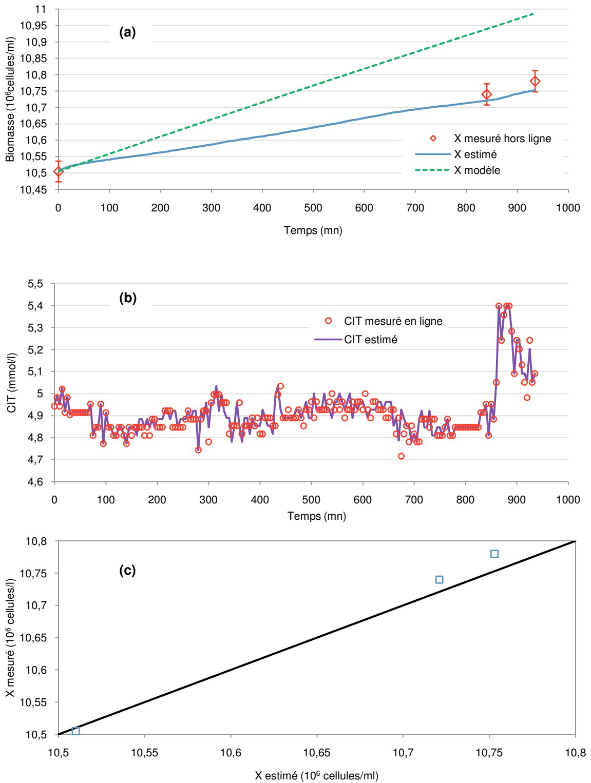
Figure 5.23: Comparaison entre des mesures directes ( \diamond , \circ ) et les prédictions ( \text{---} ) du filtre de Kalman étendu reposant sur les mesures du CIT : (a) biomasse mesuré par granulométrie (b) concentration en carbone inorganique total, (c) validation de la relation linéaire liant X estimé et X mesuré.
