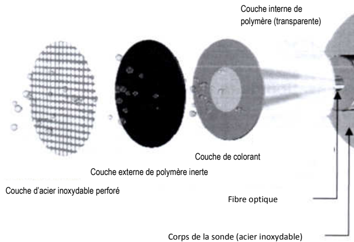
Figure 5.3 : Capsule du capteur YSI 8500 (documents YSI®).
