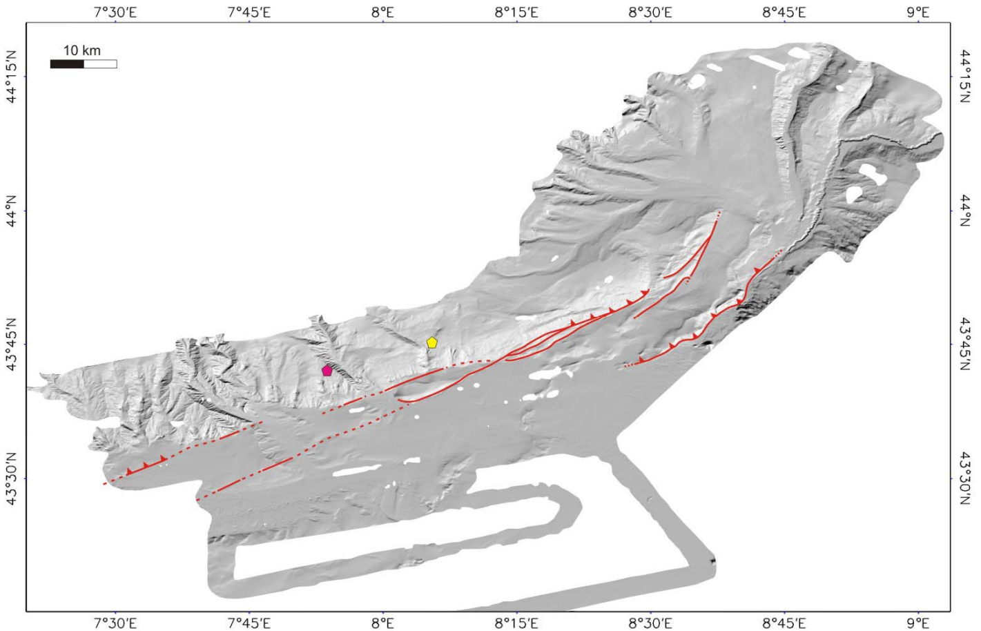
Figure II-54 : Bathymétrie EM 300 de la campagne MALISAR 1. Le faisceau de failles obliques à la marge est surligné en rouge. Les symboles rose et jaune correspondent aux épacentres possibles du séisme de 1887 déterminés par Charlier (2007), à partir des données françaises et italiennes respectivement.
