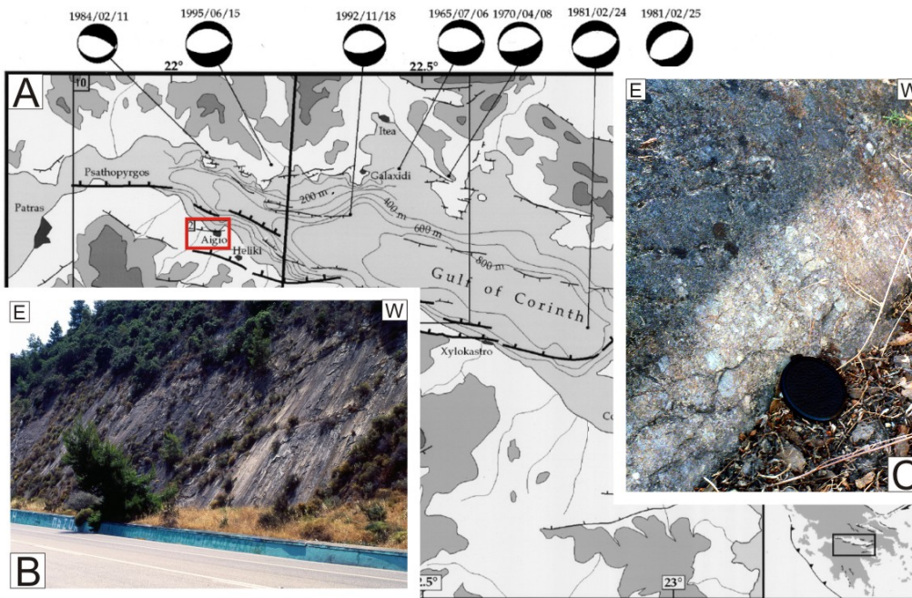
Figure II-22 : Observations de terrain après le séisme d'Aigion (Grèce, M_s=6,2 - 15/06/1995 ). A, Localisation des principales failles normales bordant le Golfe de Corinthe (d'après Bernard et al., 1997). B, L'escarpement cumulé de la faille d'Aigion (environ 80 m de hauteur) démontre que sur le long terme le glissement tectonique est plus rapide que le décapage par l'érosion. C, Décalage de surface récent au pied de l'escarpement de faille correspondant peut-être à l'événement de 1995 ou à un événement plus ancien.
