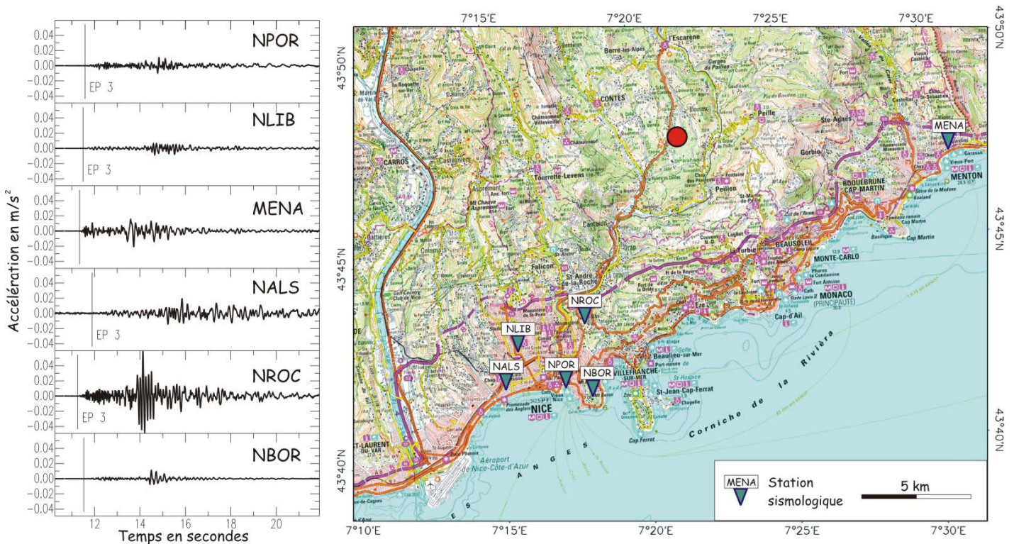
Figure I-8 : Enregistrements du séisme de Peille ( M_w=3,4 , 1/11/1999) par les stations du réseau RAP de Menton et Nice (d'après Courboux et al., 2001). L'épicentre est figuré par le rond rouge. Les accélérographes représentent la composante N-S du mouvement du sol. On observe une différence d'amplitude importante entre les sites : les enregistrements sur la station NROC ont une amplitude trois fois plus grande que ceux de la station MENA pourtant située à la même distance épicentrale, et dix fois plus grande que sur la station NLIB située à seulement 2,5 km de NROC. On note également une augmentation de la durée du signal sur les stations NROC et NALS. Les différences entre ces mouvements sont dues aux effets de site.
