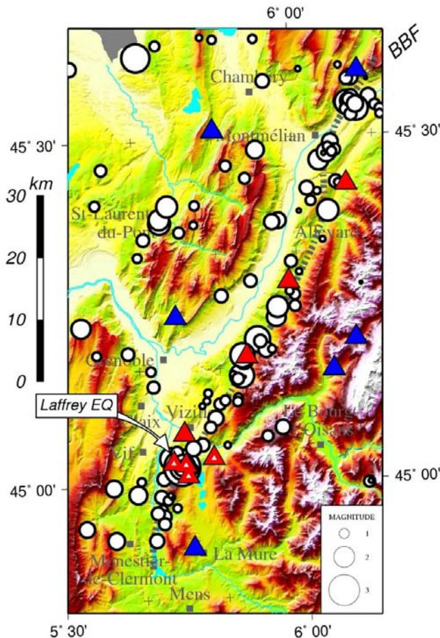
Figure II-9 : Sismicité instrumentale de la zone ouest de Belledonne pour la période 1989-2000 (d'après Thouvenot et al., 2003). Les epicentres sont les ronds blancs et le tracé de la faille bordière de Belledonne correspond aux pointillés gris. Les triangles bleus sont les stations permanentes du réseau sismalp et les triangles rouges sont les stations de la campagne de microsismicité « Belledonne Border Fault » (Décembre 1998-Mai 1999). L'épicentre du séisme de Laffrey (11/01/1999 ; Mw=3,5) est indiqué, avec les stations d'enregistrement post-sismiques (triangles rouges à points).
