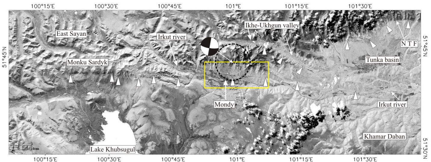
Figure III-9 : Mosaïque d'images landsat-TM (résolution 30 m) de la zone Khubsugul-Tunka. Les triangles blancs soulignent les failles actives majeures. Le cercle pointillé indique la zone épiscopentrale du séisme de Mondy et le mécanisme au foyer est tiré de Delouis et al. (2002). NTF, faille nord-Tunka. Le rectangle jaune correspond à la figure III-12 (modifié d'après Arjannikova et al., 2004).
