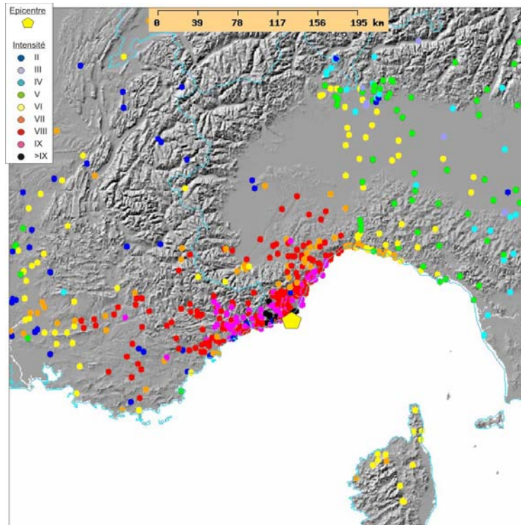
Figure II-51 : Carte des intensités épiscopentrals pour l'événement de 1887 (d'après la base de données SISFRANCE, http://www.sisfrance.net ).
