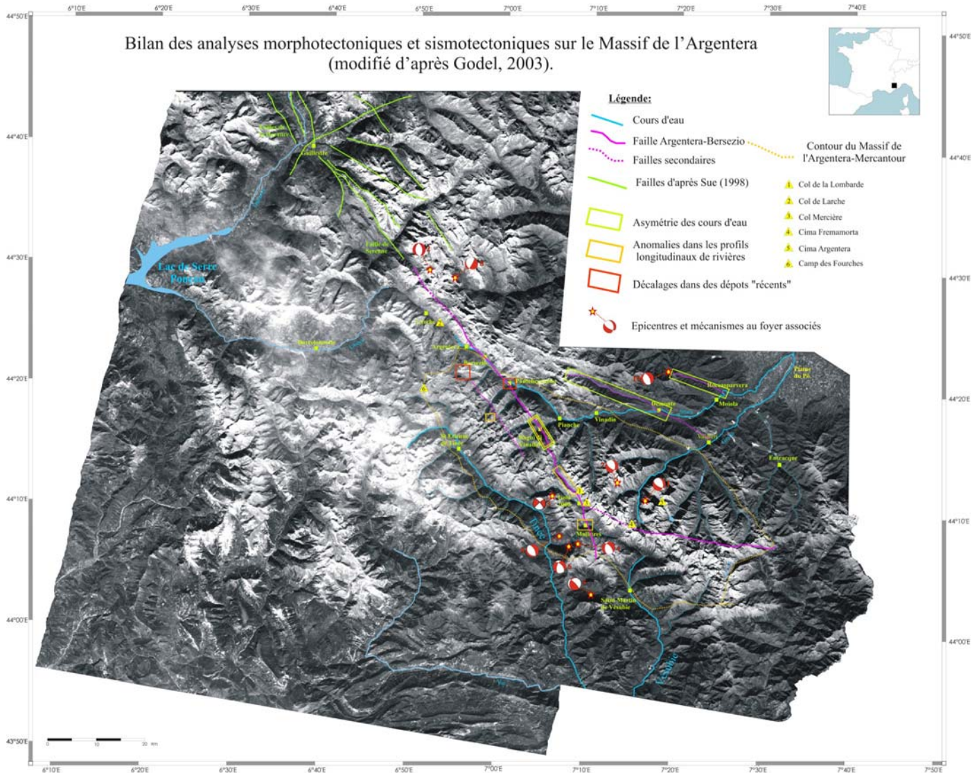
Figure II-35 : Bilan de l'analyse morphotectonique et sismotectonique sur le Massif de l'Argentera (modifié d'après Godel, 2003). Les images sont des SPOT 3 panchromatiques orthorectifiées (K52-J260, K52-J261 et K54-J261). La trace de la faille Argentera-Bersezio et de la faille Fremamorta-colle del Sabbione a été reportée sur les images SPOT à partir de l'analyse des photos aériennes. Les mécanismes au foyer correspondent aux événements suivants : 1 (07/03/1999, M_l=2,6 ), 2 (13/10/1995, M_l=3,9 ), 3 (17/10/1999, M_l=2,9 ), 4 (19/03/1997, M_l=2,5 ), 5 (23/09/2000, M_l=2,5 ), 6 (23/09/1999, M_l=2,6 ), 7 (24/11/2002, M_l=2,7 ), 8 (26/06/2000, M_l=3,3 ), 9 (30/05/2001, M_l=2,5 ) et 10 (24/10/2008, M_w=4,1 ). Toutes les données sur les mécanismes sont décrites dans Godel (2003) sauf pour l'événement de 2008 (n°10, B. Delouis, com. pers.).
