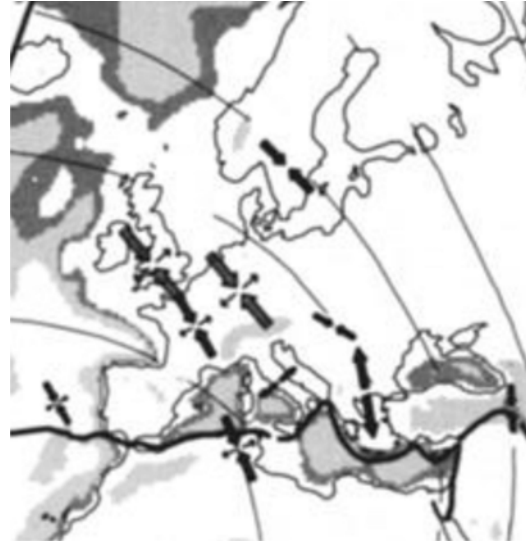
Figure I-18 : Schéma généralisé des directions de contrainte dans le domaine intraplaque ouest européen (extrait de la figure 4 de Zoback, 1992). La frontière entre la plaque Afrique et la plaque Eurasie est indiquée par le trait gras noir et les fines lignes noires représentent la direction du mouvement absolu des plaques. Les grosses et les petites flèches donnent l'orientation de SHmax et Shmin respectivement.
