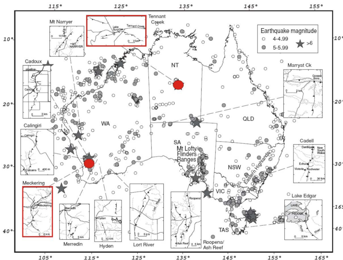
Figure I-13 : Sismicité de 1900 à 2002 en Australie (les événements de la marge nord qui ont été enlevés pour plus de clarté). Les localisations des séismes de Meckering et de Tennant Creek sont en rouges, les cartouches présentent la cartographie des ruptures de surface lorsqu'elles existent (d'après Clark et McCue, 2003).
