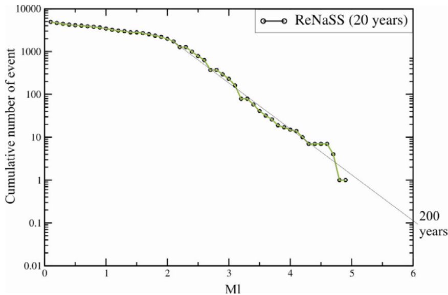
Figure II-56 : Distribution fréquence-magnitude pour les événements enregistrés par le réseau ReNaSS de 1985 à 2005 sur la zone 43°N-45°N et 6,5°E-8,5°E (d'après Courboulex et al., 2007). La courbe de Gutenberg-Richter est de la forme : \log N = a - bM ( N est le nombre de séismes de magnitude >M ; a et b sont des constantes et b , la pente de la courbe, représente la proportion de petits séismes par rapport aux grands).
