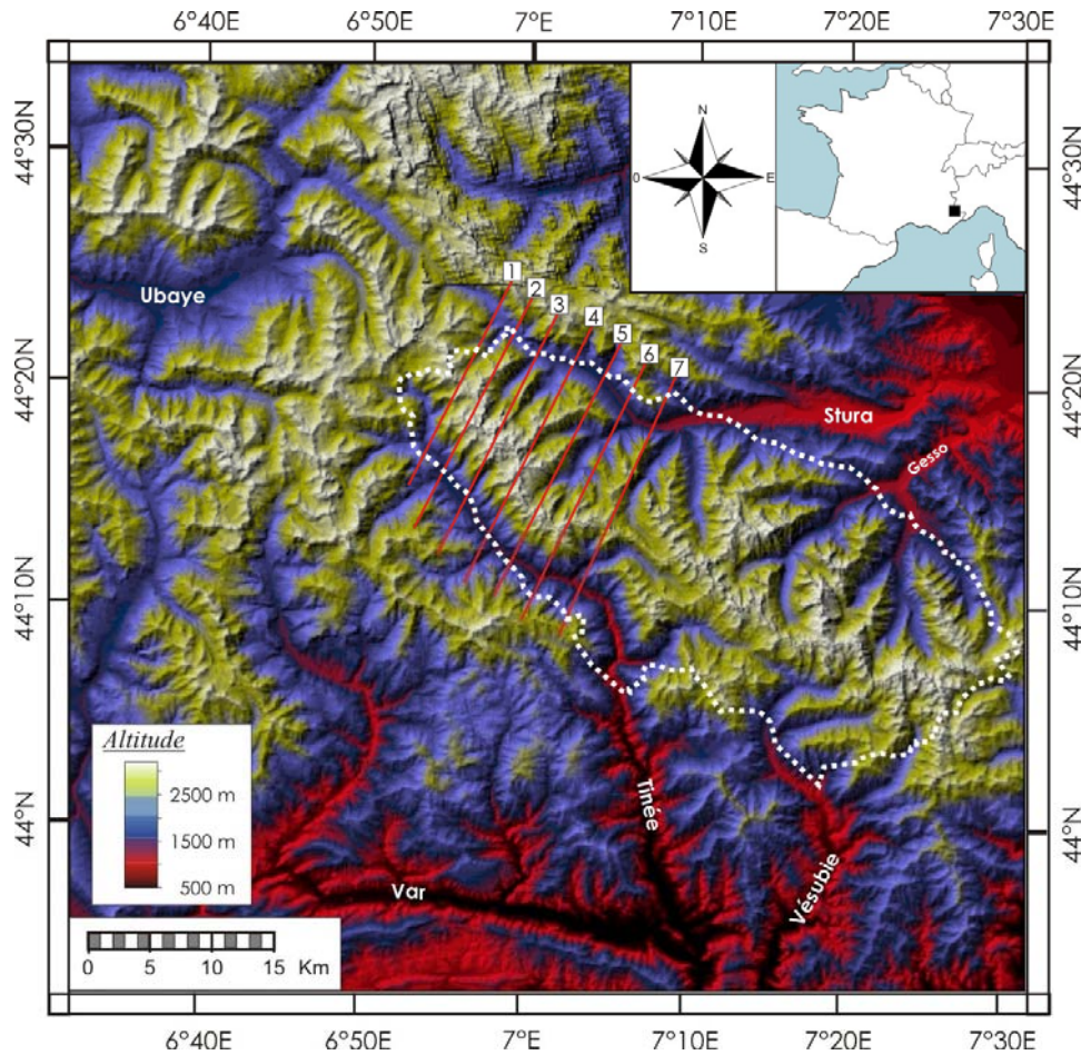
Figure II-36 : Modèle Numérique de Terrain du Massif de l'Argentera (source I.G.N et Région Ligurie). Le contour du massif est en pointillés blancs et les traits rouges correspondent aux profils topographiques de la figure II-35 (modifié d'après Godel, 2003).
