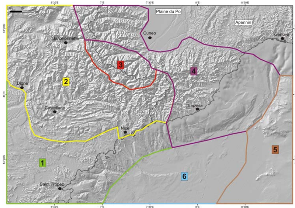
Figure II-57 : Limite des grands ensembles géologiques de la jonction Alpes – Bassin Ligure. 1, avant-pays provençale ; 2, chaînes subalpines ; 3, Massif de l'Argentera ; 4, zones internes alpines ; 5, marge sud ligure ; 6, croûte transitionnelle et croûte océanique ligure.
