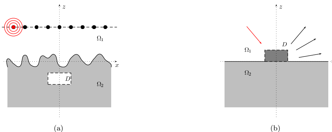
FIG. 5.11 – Configuration stratifiée (a) dans le cas d'un objet enfoui sous une interface rugueuse avec une ligne de mesure proche de la surface (b) dans le cas d'un objet posé sur une interface plane et éclairée par une onde plane incidente, par exemple dans le cas des applications en tomographie optique.
