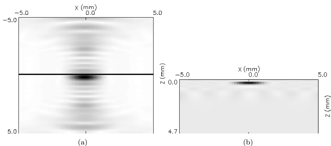
FIG. 6.6 – L’objet est dans le demi-espace inférieur. Les antennes émettrices et réceptrices se trouvent au-dessus de la surface et effectuent un balayage le long d’une ligne à plusieurs fréquences (basse fréquence). (a) Le domaine de recherche n’est pas restreint et un algorithme de tomographie classique est appliqué, (b) le domaine de recherche est limité au demi-espace inférieur et les inconnues sont projetées sur la base des fonctions Z_B . Seul le problème linéarisé est considéré dans cette configuration issue du contrôle non-destructif par courants de Foucault.
