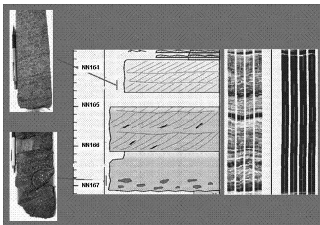
Fig. 5—Fluvial channel.
