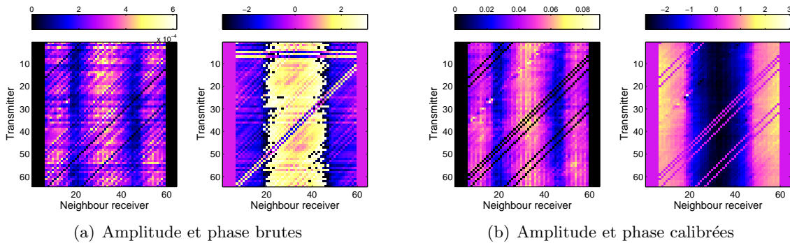
FIG. 5.8 – (a) Matrice de diffraction brute, (b) Matrice de diffraction après calibration et détection/élimination des antennes défectueuses (ce qui correspond aux lignes en noir sur la matrice de diffraction). L’objet mesuré correspond à un cylindre centré métallique de diamètre 60cm.
