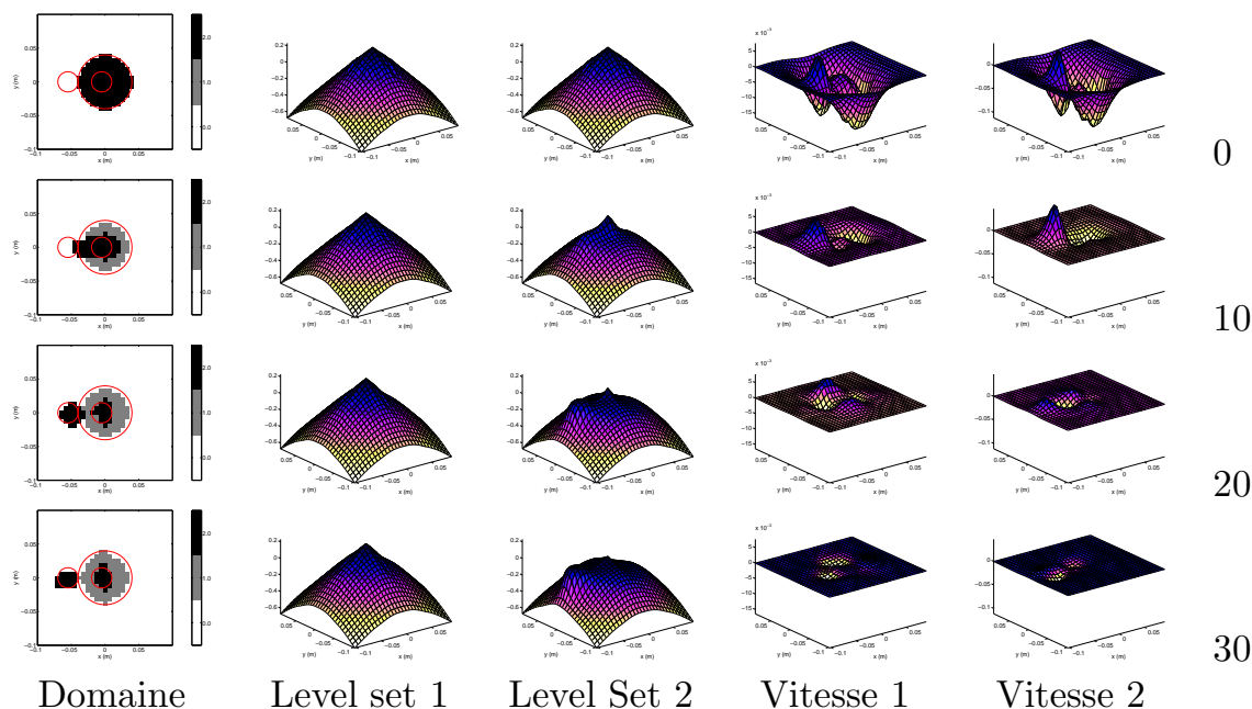
FIG. 6.13 – Evolution des fonctions de niveaux et des vitesses associés dans le cas de la reconstruction d’un objet homogène par morceau. Les champs ont été mesurés dans la chambre anéchoïque de l’Institut Fresnel et cet objet, appelé FoamTwinDiel, fait partie de la seconde base de données publiée dans la revue Inverse Problems .
