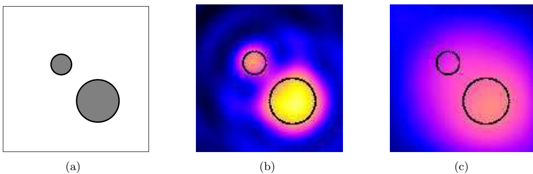
FIG. 5.5 – (a) Image exacte, (b) Image obtenue par dérivées topologiques en utilisant le module et la phase, (c) Image obtenue par dérivées topologiques en n'utilisant que le module.
