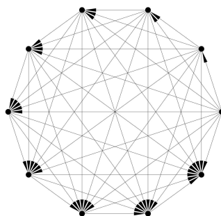
FIG. 7.17: Réseau complet unidirectionnel de 10 neurones. Dans un tel réseau, le neurone i reçoit des signaux des neurones 1, \dots, i - 1 . Ainsi, le degré entrant des neurones est compris entre 0 et 9.
