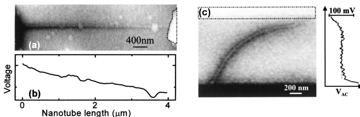
FIG. 1.20 – (a) Nanotube de carbone multiparois d'un diamètre de 9 nm imagé par ac-EFM. Une tension AC de 150 mV est appliquée sur l'électrode de gauche. (b) Signal ac-EFM le long du nanotube. (c) Signal ac-EFM d'un fagot de nanotubes monoparois. La tension AC de 100 mV est appliquée sur l'électrode du haut. La valeur du potentiel le long du nanotube est tracée à droite. (Figure adaptée de [32]).
