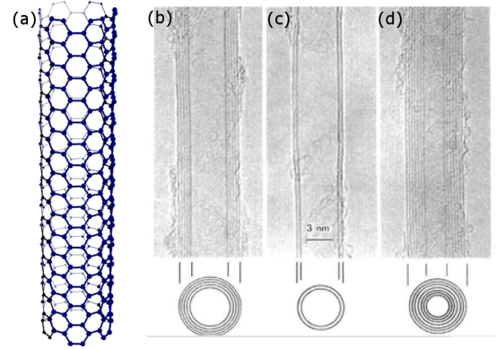
FIG. 1.2 – (a) Image d'art d'un nanotube mono-paroi. (b-d) Image TEM de nanotubes multiparois à (b) 5 parois (c) 2 parois et (d) 7 parois.
