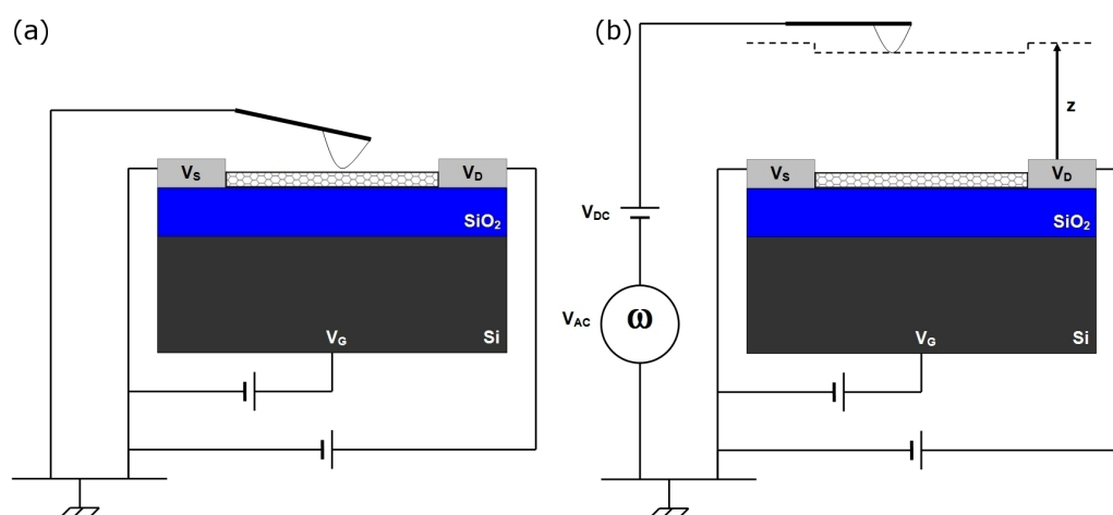
FIG. 3.4 – Imagerie KFM d'un CNTFET (a) Image de topographie AFM lors du premier aller-retour de la pointe AFM en mode tapping. (b) Imagerie KFM lors du second aller-retour de la pointe en mode lift à z constant.
