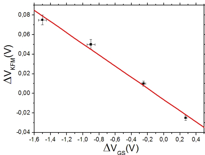
FIG. 3.19 – Réponse électrostatique du nanotube de carbone aux injections de charges en fonction de la réponse électrique.
