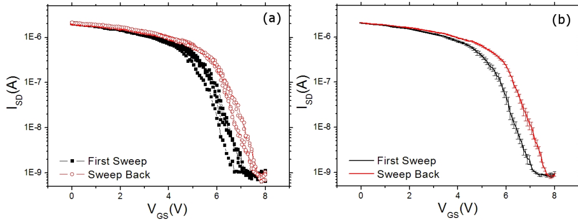
FIG. 3.3 – (a) Caractéristiques de transfert allers-retours successives d'un CNTFET, le balayage aller est représenté par les carrés noirs, le balayage retour est représenté par les cercles rouges. (b) Caractéristique de transfert moyenne avec les marges d'erreur standard. Le tracé en noir (à gauche) est le balayage aller et le tracé en rouge (à droite) est le balayage retour.
