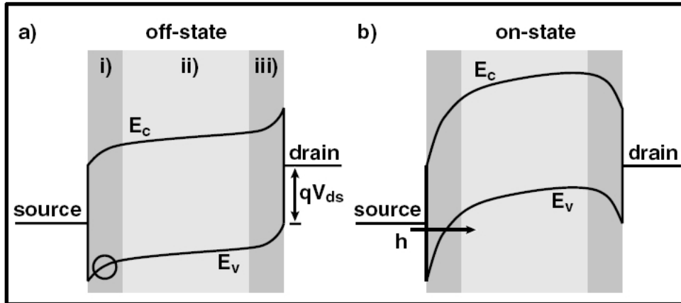
FIG. 1.15 – Réponse qualitative des bandes de conduction et de valence d'un nanotube de carbone pour une tension négative V_{DS} fixée négative. (a) Le potentiel de grille est en dessous de la tension seuil et décrit l'état OFF. (c) Courbure de bandes décrivant l'état ON où la tension de grille est supérieure à la tension seuil. (Figure adaptée [20])
