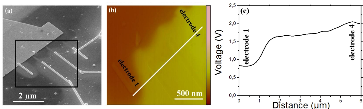
FIG. 2.10 – (a) Image SEM d'un nanotube de carbone multiparois d'un diamètre de 16 nm connecté en 4 points par du platine déposé par IBID. (b) Image KFM de la zone délimitée par le rectangle noir indiqué en (a), l'échelle correspond de bas en haut à 0 à 6V. (c) Potentiel de surface le long de la ligne blanche tracée en (b).
