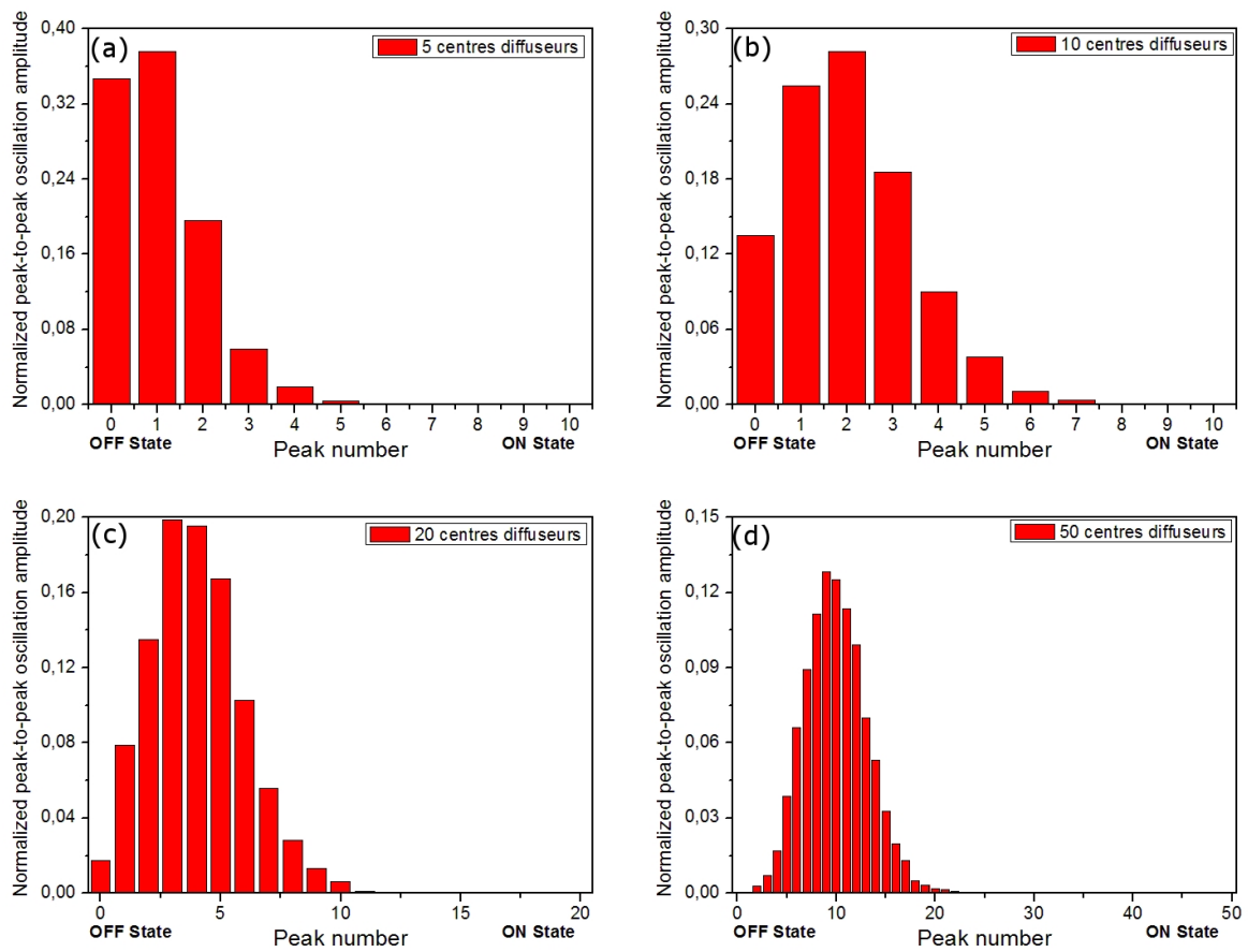
FIG. 4.11 – Distributions de phonons par des probabilités totales d'avoir émis N phonons sur les N_{\text{diff}} sites possibles. On choisit g = 0.2 , et (a) N_{\text{diff}} = 5 sites, (b) 10 sites, (c) 20 sites et (d) 50 sites.
