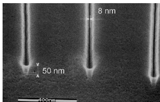
FIG. 2.4 – Gravure ultime par FIB
