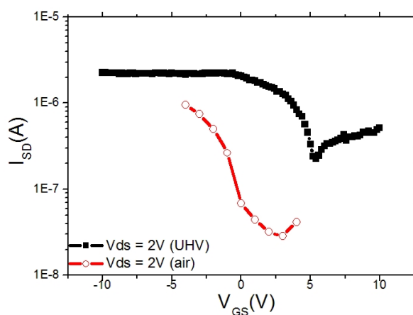
FIG. 3.22 – Caractéristiques de transfert du transistor de la figure 3.23 pour V_{DS} = +2V sous ultra-vide et à l'air ambiant.
