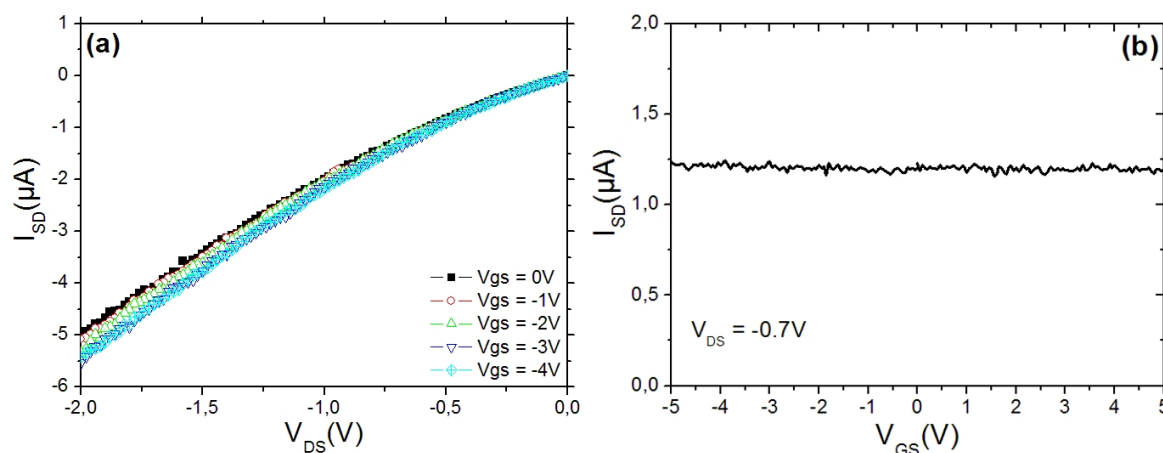
FIG. 2.20 – (a) Caractéristique de transfert I_{SD}(V_{GS}) d'un nanotube de carbone métallique; (b) Caractéristique I_{DS}(V_{DS}) d'un nanotube de carbone métallique.
