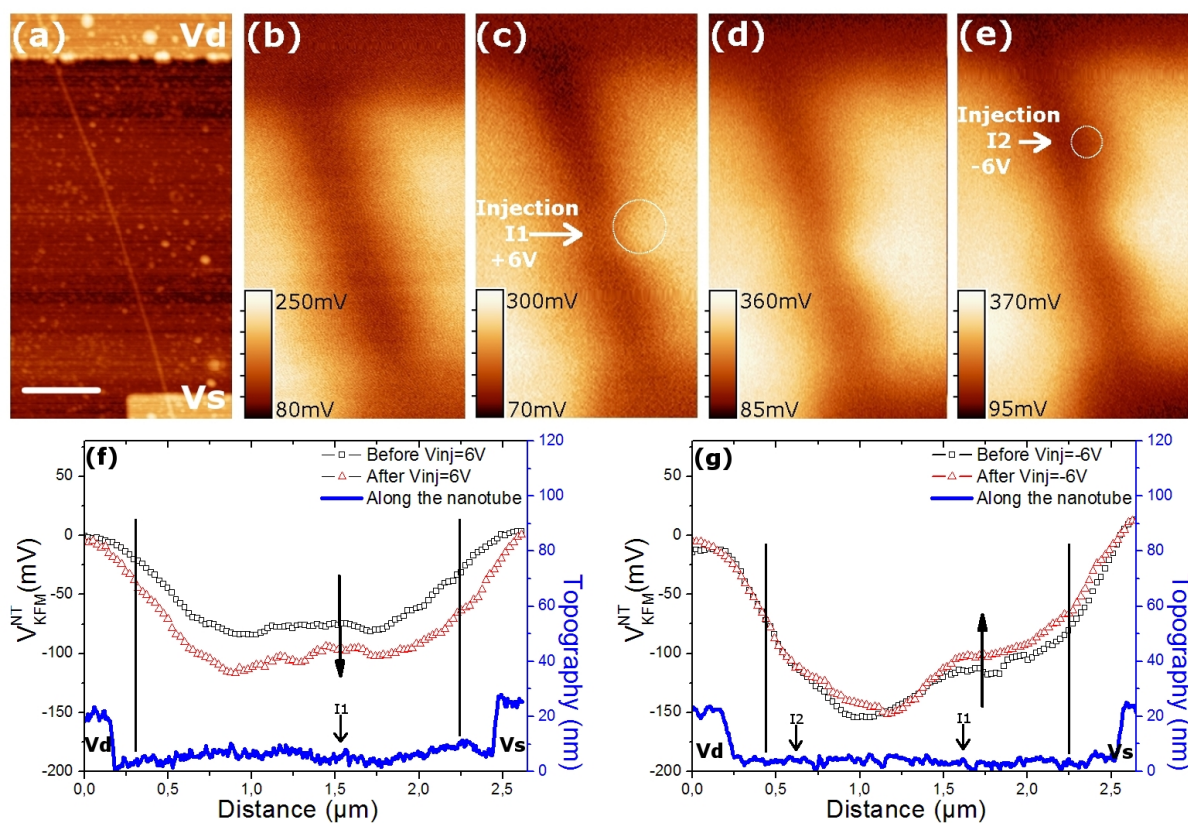
FIG. 3.17 – (a) Image AFM du transistor SC1, la barre d'échelle correspond à 500 nm (b-e) Images KFM des injections de charges (b) Avant I1 à V_{inj} = +6V (c) après I1, le cercle blanc indique la zone chargée. (d) Avant I2 à V_{inj} = -6V (e) Après I2, le cercle blanc indique la zone chargée. (f-g) Potentiels V_{KFM}^{NT} le long du nanotube (en soustrayant le signal équivalent loin du nanotube) (f) avant et après l'injection I1 (indiquée sur le graphe) (g) puis avant et après l'injection I2 (indiquée sur le graphe ainsi que l'injection précédente I1). Les barres verticales délimitent la région relative au nanotube seul et les deux régions relatives aux électrodes, les flèches noires verticales indiquent le décalage global du potentiel de surface le long du nanotube.
