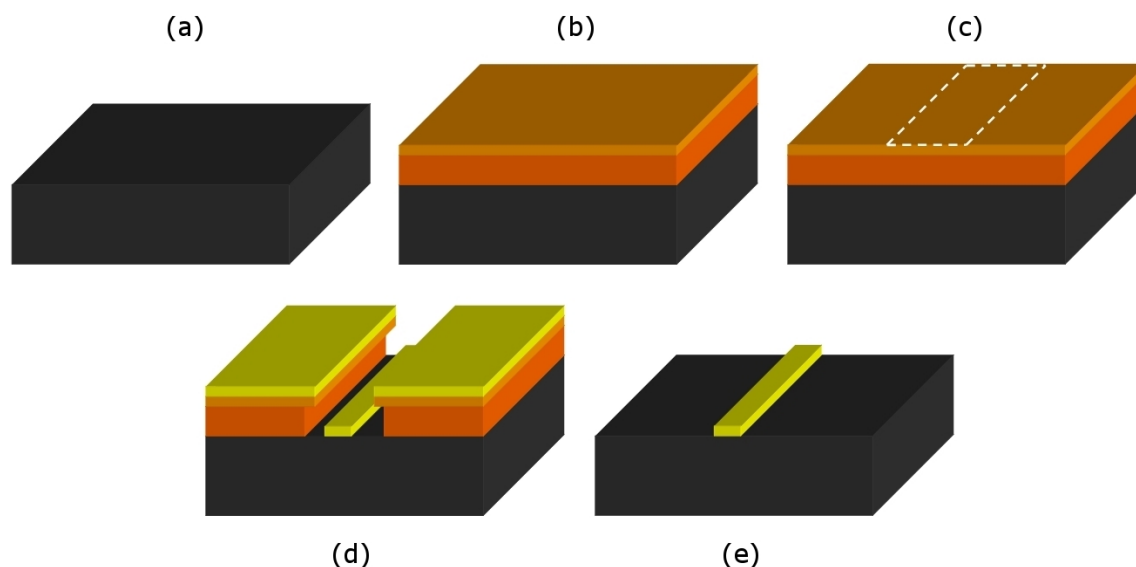
FIG. 2.14 – Schéma de fabrication d'électrodes sur une surface de Si/SiO 2 par lithographie électronique. (a) Substrat initial, (b) Dépôt d'un bicouche de résines électroniques pour l'obtention d'un profil en 'casquette', (c) Insolation par le faisceau d'électrons de la zone délimitée par les pointillés, (d) Révélation de la zone insolée, (e) Evaporation des métaux. (f) Lift off.
