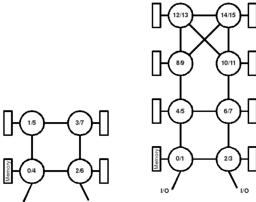
(a) Nœud du cluster Borderline à base de 4 OPTERONS dual-core, Grid5000.
