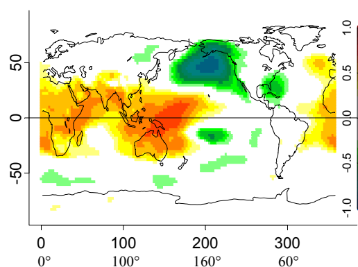
(c) Cor ( Indice DA, PNM.JFM) 1950-2001
