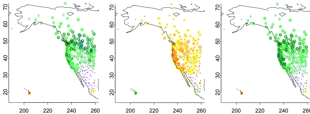
(a) Cor(Indice D, Tmin10)
