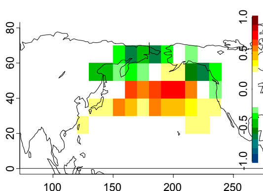
(d) Cor (Indice CP1-FD.CNRM-CM3, Freq.D)
