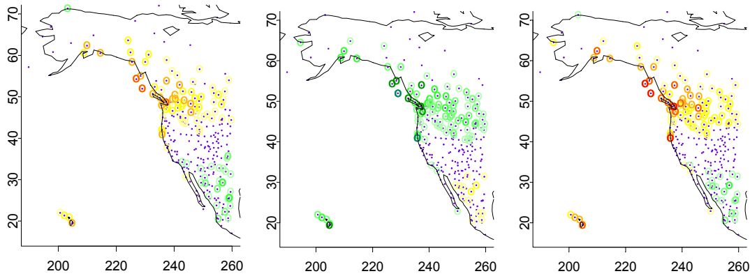
Figure 5.15. Coefficients de corrélations linéaires entre la fréquence des nuits extrêmement chaudes (Tmin90) et les indices D, A et DA (a, b, c) en JFM 1950-2001. Même chose pour la fréquence des journées extrêmement chaudes (Tmax90) (d, e, f). (couleurs = sig. > 95%, t-test bilatéral).
