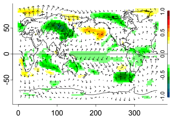
Figure 7.10. Première composante principale de l'intensité des anticyclones (CP1-IA.NCEP-NCAR : intensité = pression centrale pour les anticyclones), indices CP1-IA (a, b), carte des coefficients de corrélation linéaire entre les indices précédents et l'intensité des anticyclones (c, d), les pressions au niveau de la mer (e, f), les températures de l'air à 2 m et le vent à 10m (g, h). Les couleurs = corrélations sig.> 95%. A gauche d'après les Réanalyses et à droite d'après la simulation XX1 du modèle CNRM-CM3.
