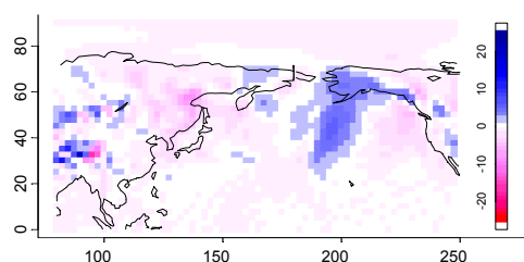
(a) Variation PNM ouest – est (hPa)
