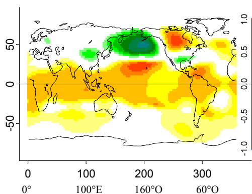
(c) Cor ( Indice DA, G200.JFM) 1950-2001
