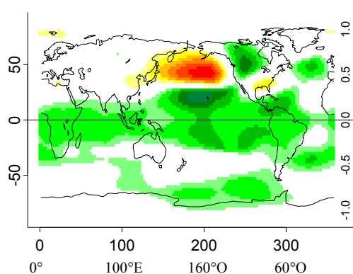
(b) Cor ( Indice A, G200.JFM) 1950-2001
