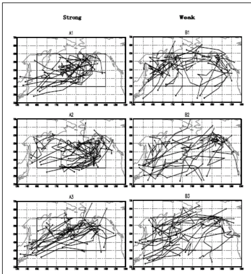
Figure 3.1. Trajectoires des dépressions ayant atteint la zone 40^{\circ}\text{N}-60^{\circ}\text{N} / 150^{\circ}\text{E}-140^{\circ}\text{O} , au cours des mois de décembre – janvier – février (DJF), 1976-77 (A1), 1982-1983 (A2), 1986-1987 (A3), 1968-1969 (B1), 1970-1971 (B2), 1971-1972 (B3). A gauche, (A) correspondent les hivers durant lesquels la dépression des Aléoutiennes est intensifiée et à droite, (B) anormalement affaiblie. Xioje et al. (2006).
