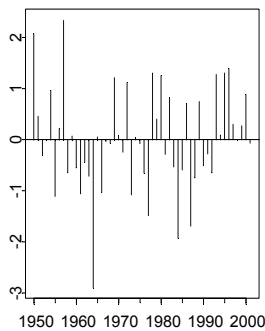
(g) CP2Tmin (15%)
