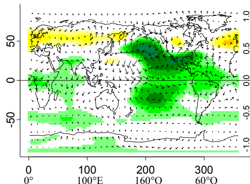
(b) Cor ( Indice A, Ta200&V200.JFM) 1950-2001
