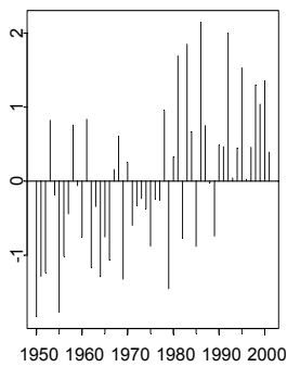
(g) CP2Tmin (15%)
