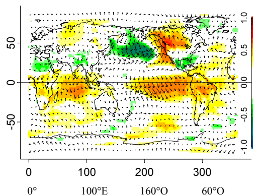
(c) Cor ( Indice DA, Ta2m&V10.JFM) 1950-2001
