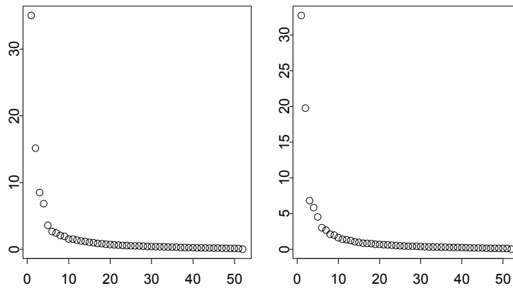
(d) Corrélations
