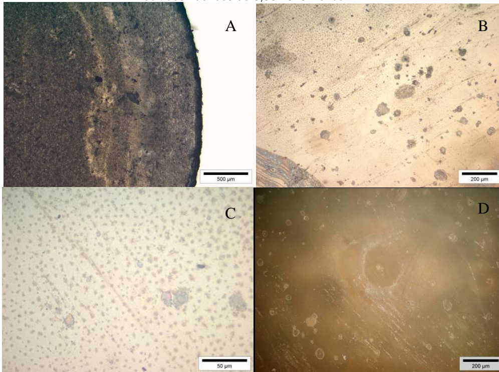
Figure VI. 20 Photographie en microscopie optique de la face d'entrée (A, échelle : 500 µm BF) et de la face de sortie (B, échelle : 50 µm, DF) (C, échelle : 200 µm, BF ; D, échelle : 200 µm, DF) de lame de verre \text{II-L}_{20}\text{Y}_5\text{C}_0\text{AS} irradié par un faisceau de 100 nA pendant 1 heure soit une fluence de 3,96 \cdot 10^{15} \text{ He}^{2+}/\text{cm}^2 .
