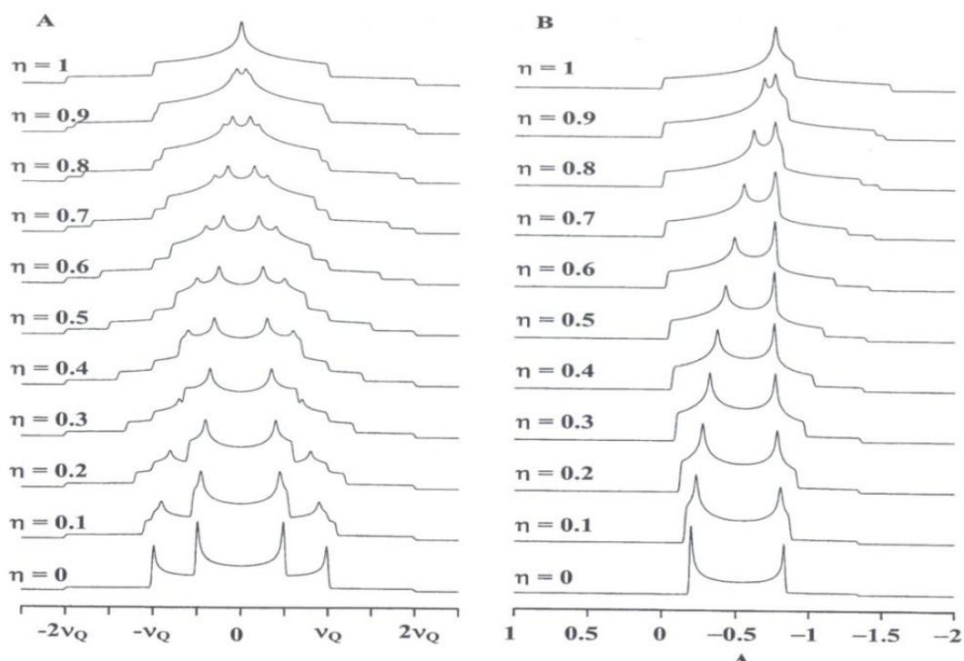
Figure III. 11. Forme théorique des transitions satellites statiques élargies au premier ordre (A) et de la transition centrale MAS élargie au second ordre (B) [45].
