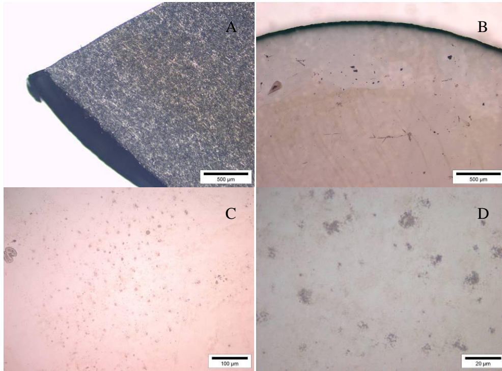
Figure VI. 19 Photo en microscopie optique de la face de sortie (B, échelle : 500 µm, BF ; C, échelle : 100 µm, BF ; D, échelle : 20 µm, BF) de lame de verre \text{II-L}_5\text{Y}_{20}\text{C}_5\text{AS} irradié par un faisceau de 100 nA pendant 1 heure soit des fluences de 3,96 \cdot 10^{15} \text{ He}^{2+}/\text{cm}^2 .
