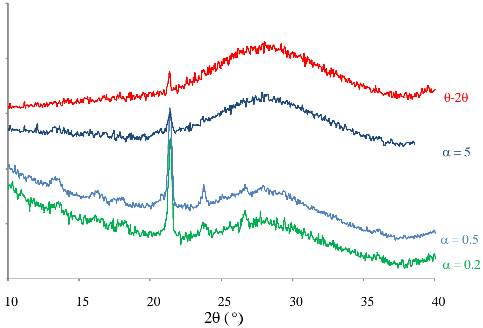
Figure VI. 24 Diffractogrammes de la face d'entrée de la lame de verre II-L 20 Y 5 C 0 AS irradié par un faisceau de 100 nA soit 10^{12} \alpha/cm^2.s pour différente valeur de l'angle \alpha incident.
