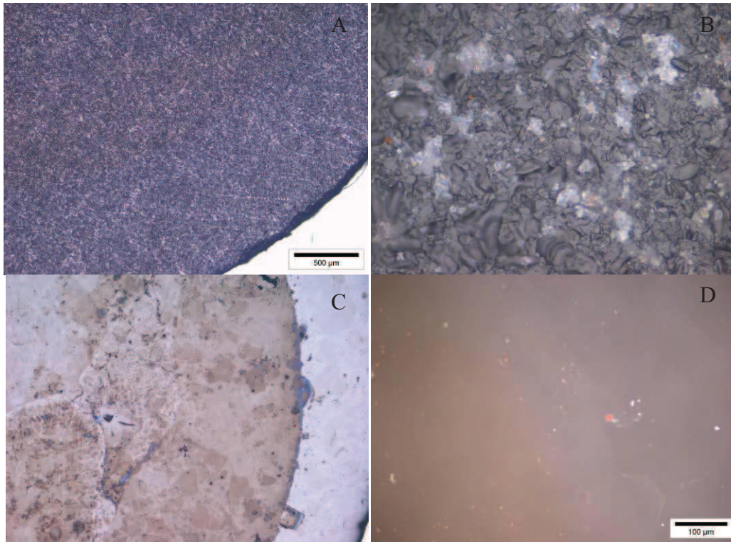
Figure VI. 18 Photographie en microscopie optique de la face d'entrée (A, échelle : 500 µm, BF ; B échelle : 20 µm BF) et de la face de sortie (C, échelle : 500 µm, BF ; D, échelle : 100 µm, DF) de lame de verre II-L 5 Y 20 C 5 AS irradiée par un faisceau de 1 nA pendant 1 heure soit une fluence de 3,96 10 13 He 2+ /cm 2 .
