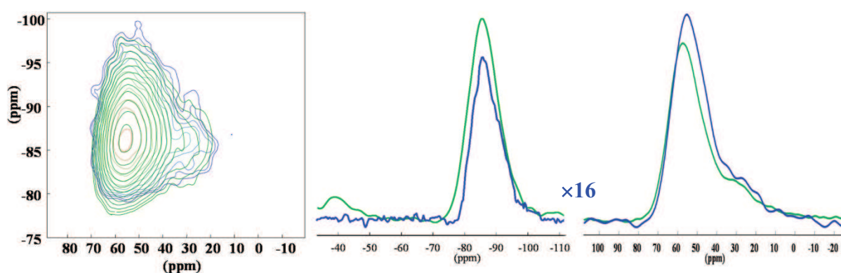
Figure IV. 20 Comparaison des spectres ^{27}\text{Al}/^{29}\text{Si} MAS HMQC, et des projections ^{29}\text{Si} et ^{27}\text{Al} des échantillons II- \text{L}_5\text{Y}_{20}\text{C}_5\text{AS} en abondance naturel (4096 scans – 3 jours - bleu) et IV- \text{C}_5\text{L}_5\text{Y}_{20}\text{AS} enrichi (256 scans – 4 h - vert)
