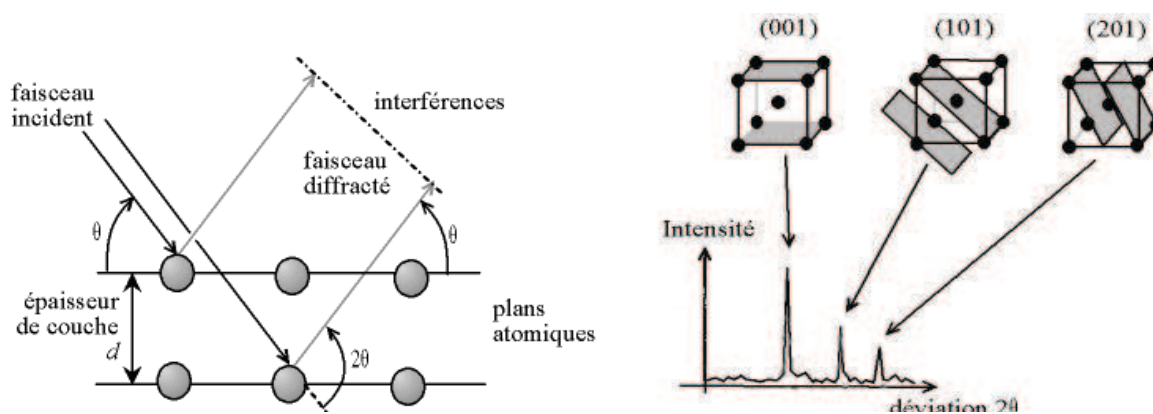
Figure IV. 9. Schématisation du phénomène de diffraction des rayons X
