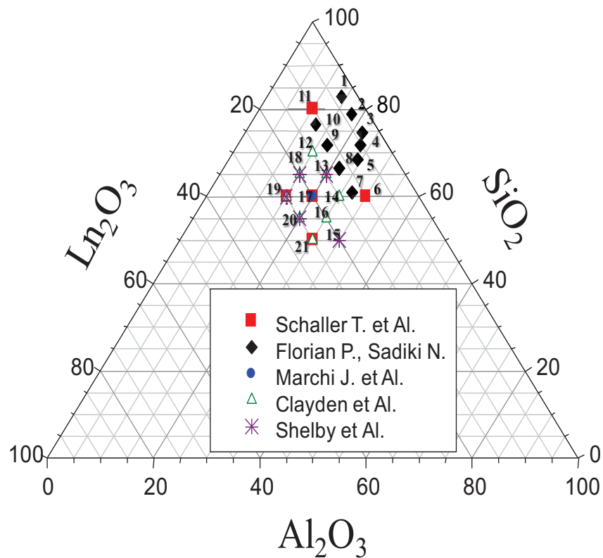
Figure II. 15. Synthèse des études en RMN 27 Al et 29 Si. Chaque point est annoté puis répertorié dans le tableau. On précisera la terre rare introduite dans le réseau dans la première colonne, puis les espèces aluminium et silicium présentes (×) et éventuellement leur teneur approximative si une étude quantitative a été réalisée.
