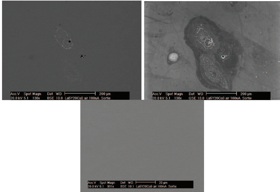
Figure VI. 23 Photo de microscopie électronique à balayage de la face de sortie de la lame de verre \text{II-L}_5\text{Y}_{20}\text{C}_0\text{AS} irradié par un faisceau de 100 nA pendant 1 heure soit une fluence de 3,96 \cdot 10^{15} \text{ He}^{2+}/\text{cm}^2 .
