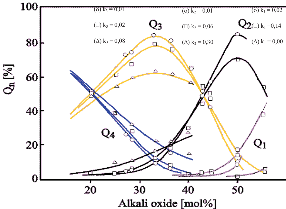
Figure II. 11. Distribution des entités Q^n au sein des verres SiO_2-M_2O en fonction de la teneur en oxyde d'alcalin M_2O avec M = K ( \circ ), Na ( \square ), Li ( \Delta ) et k_n les constantes de dissociation [42].
