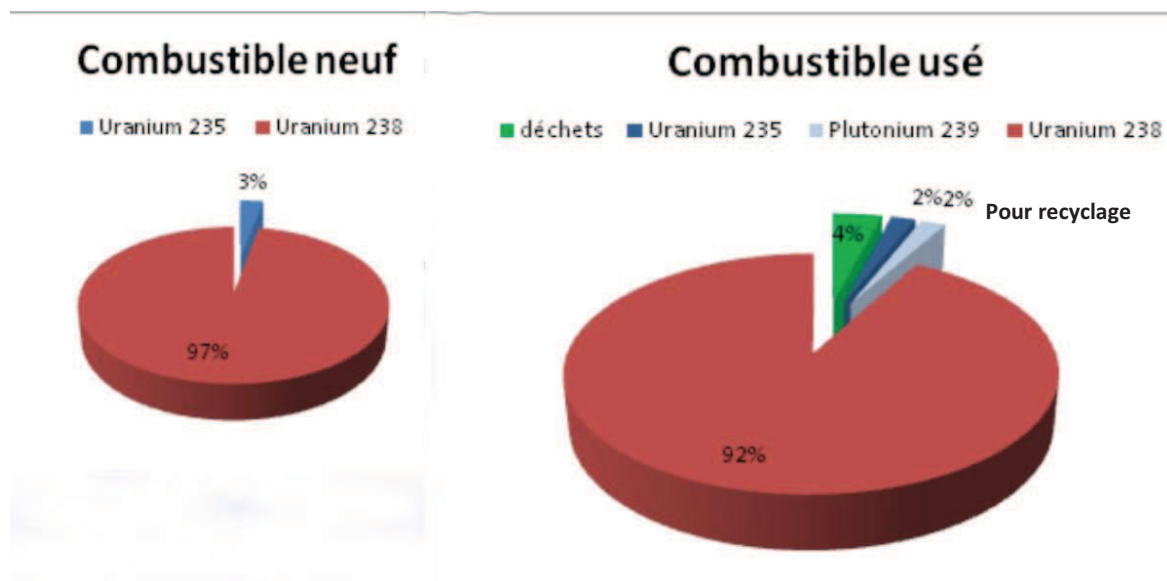
Figure I. 3. Composition des combustibles neuf et usé
