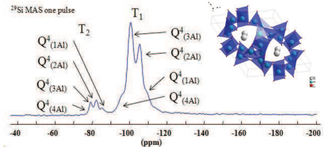
Figure III. 20 Spectre MAS RMN ^{29}\text{Si} de la cordiérite hexagonale ( \text{Mg}_2\text{Al}_4\text{Si}_5\text{O}_{18} : groupe d'espace P6/mcc) dont la représentation 3D montre l'existence d'un site T_1 , formant un hexagone composé de six tétraèdres ou « ring », et d'un site T_2 reliant les hexagones empilés parallèlement les uns par rapport aux autres. Dans la maille, composée potentiellement de 9 tétraèdres Al/Si, on doit retrouver 3 sites T_1 et 6 sites T_2 . Les Si seront préférentiellement sur les sites T_2 et les Al sur les sites T_1 . Dans la cordiérite naturelle, les taux d'occupation sont les suivants : T_1 : 0,72 Al/0,29Si et T_2 : 0,30Al/0,70Si [104]. Le calcul du rapport Si/Al dans la maille, montre qu'il est fort probable que des liaisons Al-O-Al existent (1,5 104).
