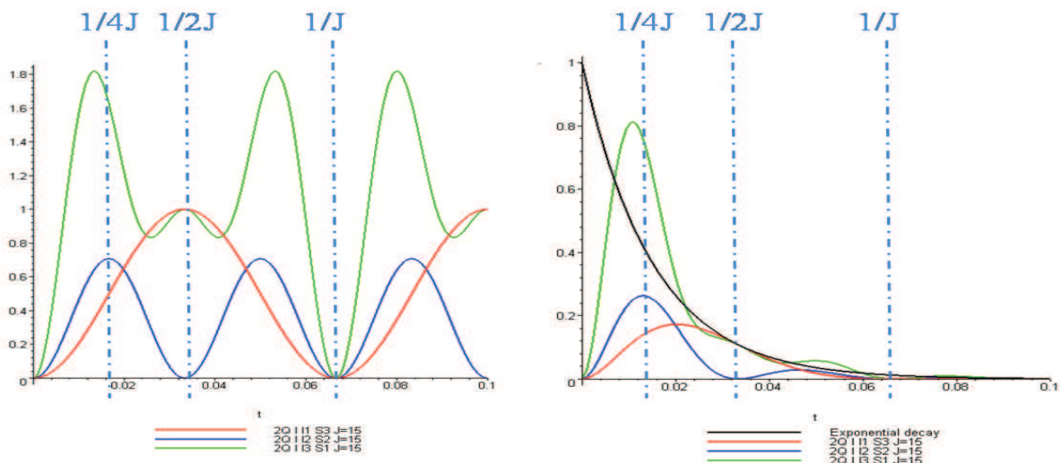
Figure III. 24 Build up théoriques et normés des signaux 2Q des unités I(I_3S_1) en bleu, I(I_2S_2) en vert et I(I_1S_3) en rouge pour une valeur de couplage scalaire J = 15 Hz.
