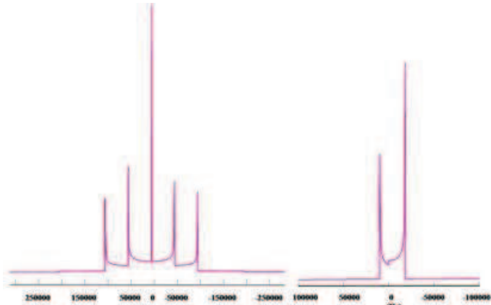
Figure III. 12. Spectre de poudres théorique statique pour un noyau de spin I = 5/2 pour l'ensemble des transitions ( CT \pm 1/2 ; ST \pm 1/2 \leftrightarrow \pm 3/2 ; ST \pm 3/2 \leftrightarrow \pm 5/2 – à gauche) et pour la transition centrale (à droite) élargie au second ordre.
