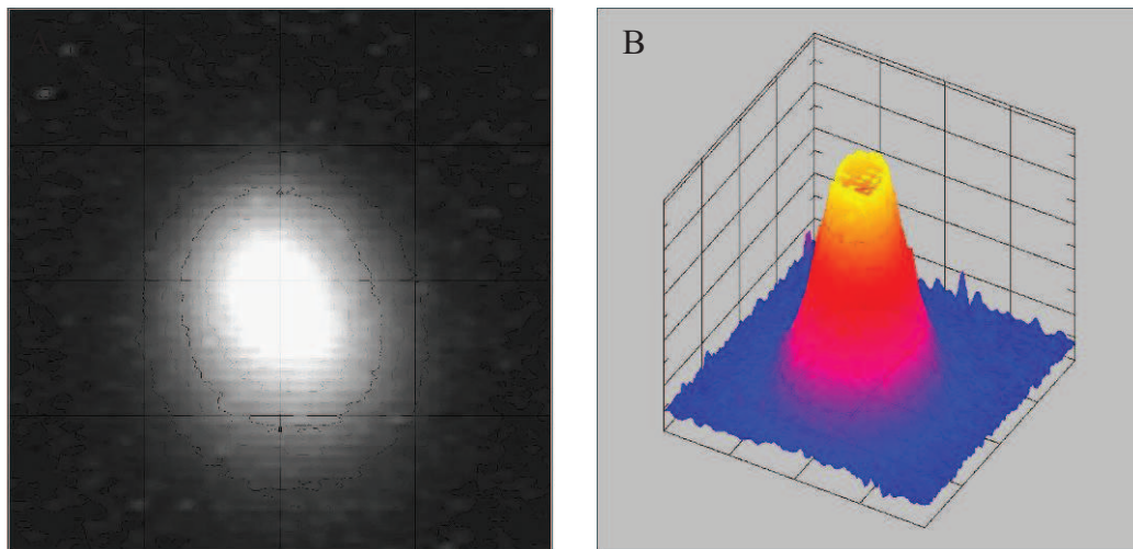
Figure VI. 15 Visualisation 2D d'un faisceau homogène, rond, capté par une alumine placé sur son trajet (A) lors de l'irradiation du verre II-La 5 Y 20 Ca 5 AS, puis reprocessé en 3D pour présenter le front du faisceau, de forme gaussienne quand le faisceau est homogène (B).
