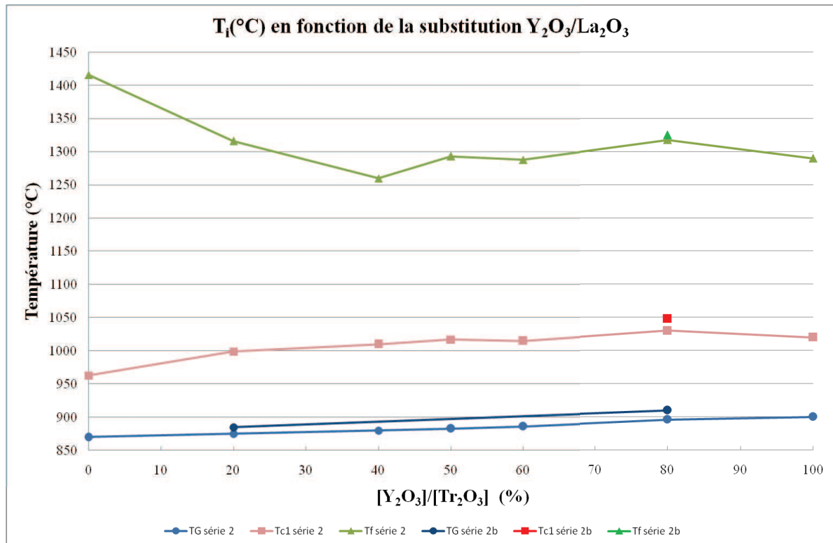
Figure V. 3 Evolution de T_g , T_c et T_f en fonction du rapport R_2 = [Y_2O_3]/[Tr_2O_3] pour la série II- L_xY_5C_5AS et II- L_xY_5C_0AS (b).
