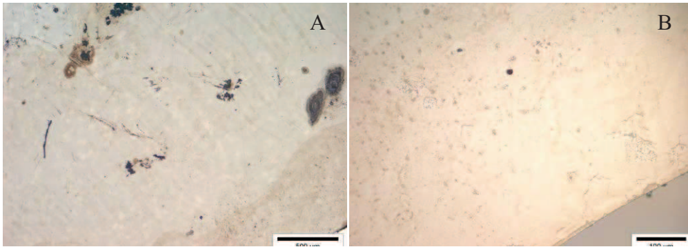
Figure VI. 21 Photo en microscopie optique de la face de sortie (A, échelle : 500 \mu\text{m} BF ; B, échelle : 100 \mu\text{m} BF) de lame de verre II-L 5 Y 20 C 0 AS irradié par un faisceau de 100 nA pendant 1 heure soit une fluence 3,96 10 15 He 2+ /cm 2 .
