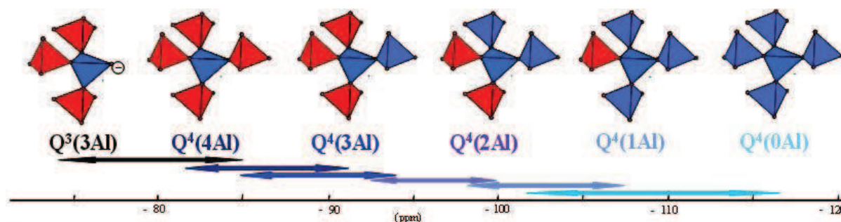
Figure III. 3. Influence de l'environnement du noyau sur le déplacement chimique. Exemple du silicium et des unités Q^n(mAl) dans les aluminosilicates, des espèces Q^4(0Al) les plus écrantées (faible ppm) aux espèces Q^4(3Al) les moins écrantées (haut ppm) – Si en bleu / Al en rouge.
