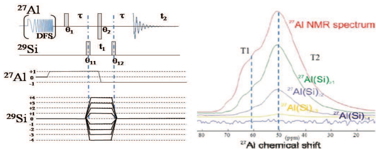
Figure III. 27 Description théorique de la séquence HMQC filtrée Multi-Quanta avec p l'ordre des cohérences. La forme de cette séquence est identique à celle présentée dans le paragraphe 2.5. Seul le cyclage de phase diffère. En l'occurrence la phase \phi_{22} est décalée de 90^\circ par rapport \phi_{11} . Les pulses sont cyclé sur \pi/8 .
