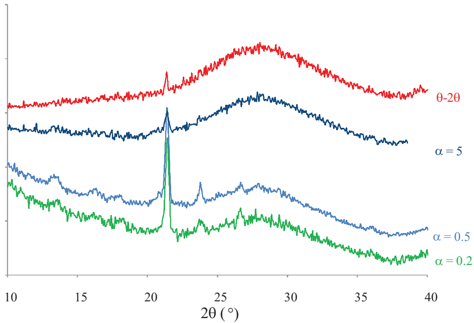
Figure VI. 24 Diffractogrammes de la face d'entrée de la lame de verre II-L 20 Y 5 C 0 AS irradié par un faisceau de 100 nA soit 10^{12} \alpha/cm^2 \cdot s pour différente valeur de l'angle \alpha incident.
