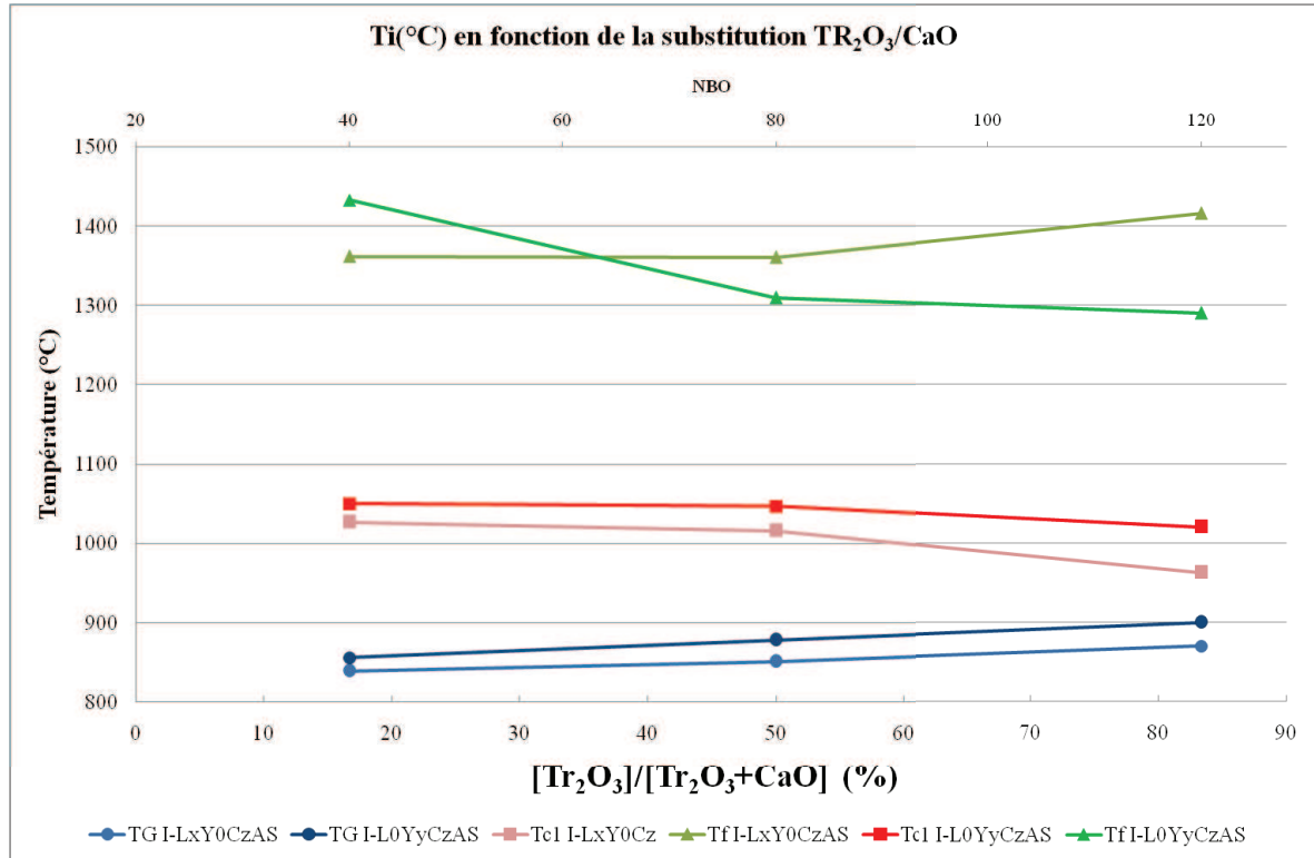
Figure V. 1. Evolution de T g , T c et T f en fonction du nombre d'oxygènes non-pontants (NBO) et de R 1 = [Tr 2 O 3 ]/{[Tr 2 O 3 ]+[CaO]} (%).
