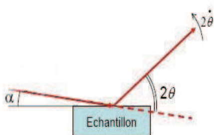
Figure IV. 22. Photographie du diffractomètre Phillips et principe du montage en incidence rasante utilisé dans cet appareillage.
