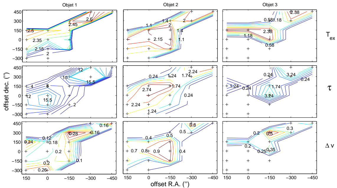
FIGURE 6.14 – Carte des valeurs de T ex , τ et Δv pour les trois composantes en vitesse observées dans TMC-1, déduites des observations. Les croix symbolisent les points d’observation.
