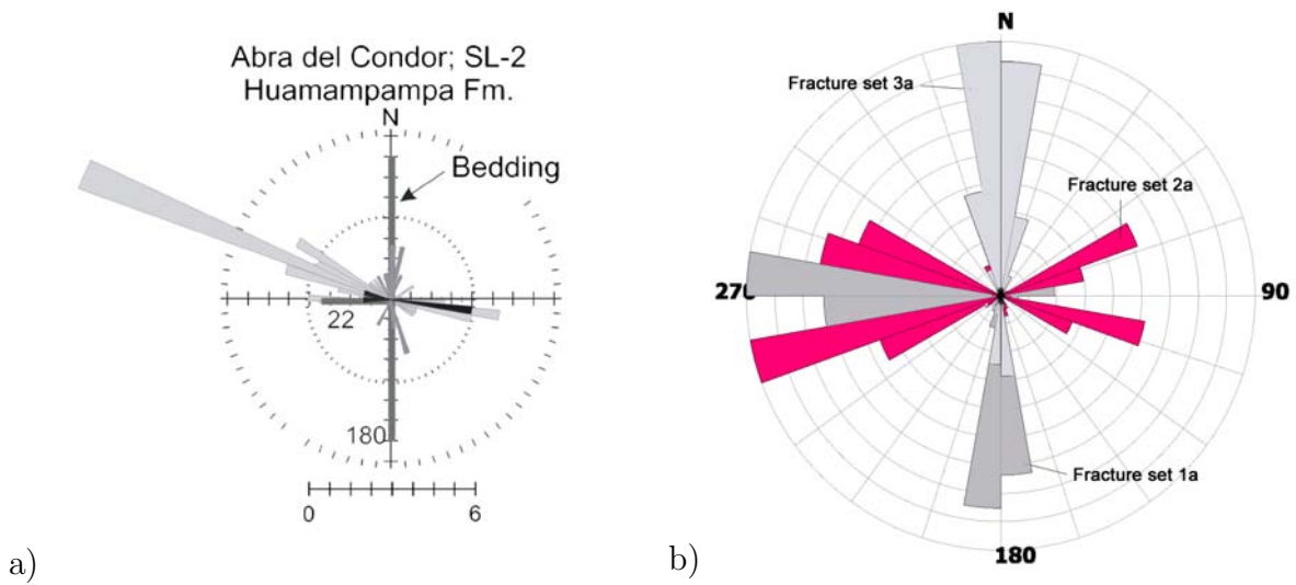
Figure 4.27 – Azimuts des fractures pour le modèle Final. Figure a) : azimuts des fractures mesurées sur l'anticlinal Abra del Condor [Florez-Niño et al. , 2005]. Figure b) : azimuts des fractures générées (famille a), pour le modèle Final, à l'aide du facteur de forme \overline{R^*} , choisi avec QC(R^*) \geq 0.9 et du critère de Coulomb. La nomenclature utilisée est celle introduite à la figure 4.10.
