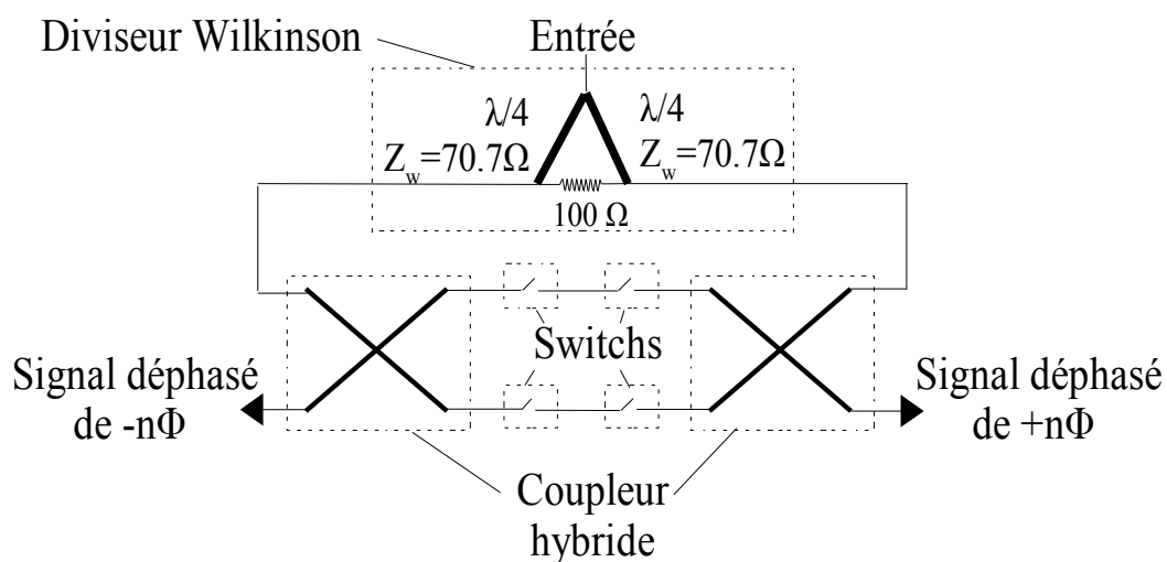
Figure V.2: Topologie du circuit d'alimentation de l'antenne à 2 patchs
