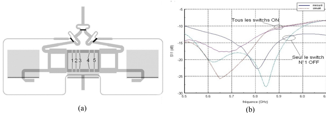
Figure V.9: (a) Vue de dessus : coupleurs hybrides en gris foncé, fentes en noir, patchs en gris clair (b) S_{11} pour 2 lois de phase
