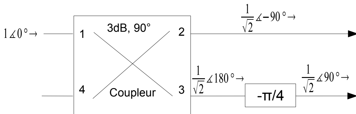
Figure V.14: Hybride 180° à partir d'un hybride 90°
