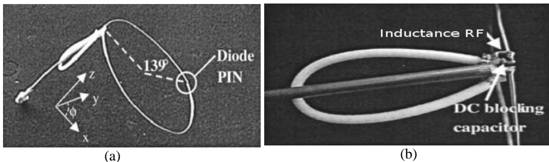
Figure II.51: (a) Antenne spire commutable (b) Vue du contact d'alimentation
