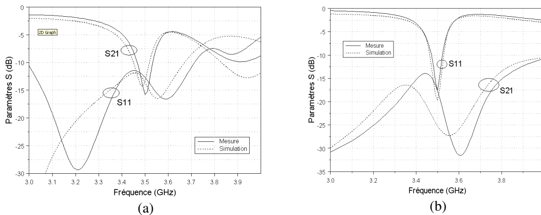
Figure IV.40: Adaptation et pertes de l'antenne pour une tension de 0,96V (a) et 15V (b)
