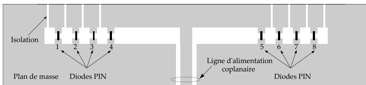
Figure I.19: Antenne à 5 fréquences commutables
