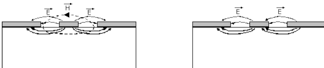
(a) mode quasi TEM
