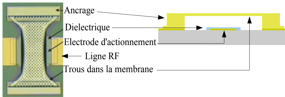
Figure II.19: (a) Photographie du switch de RATHEON SYSTEMS et (b) vue en coupe
