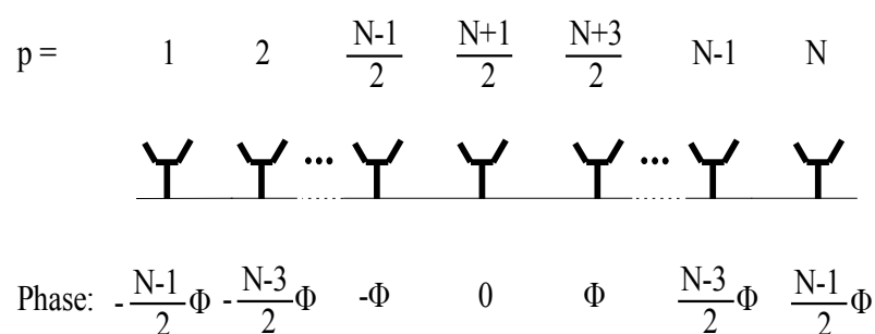
Figure V.1: Distribution de phase pour un réseau de N antennes
