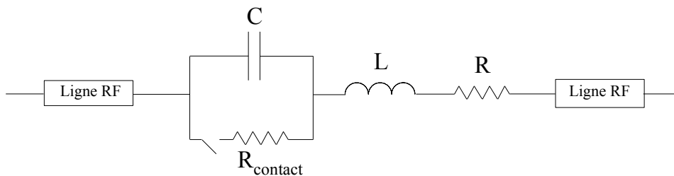
Figure II.5: Modèle représentatif d'un microcommutateur ohmique série
