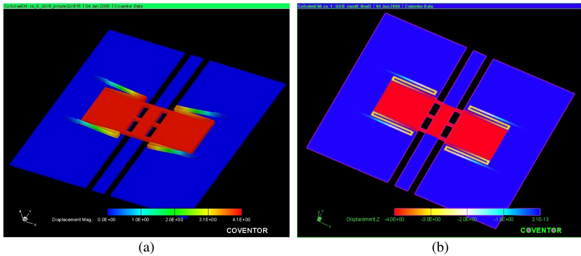
Figure III.12: (a) Membrane MEMS avec 1 serpentins (b) Membrane MEMS avec 1.5 serpentins
