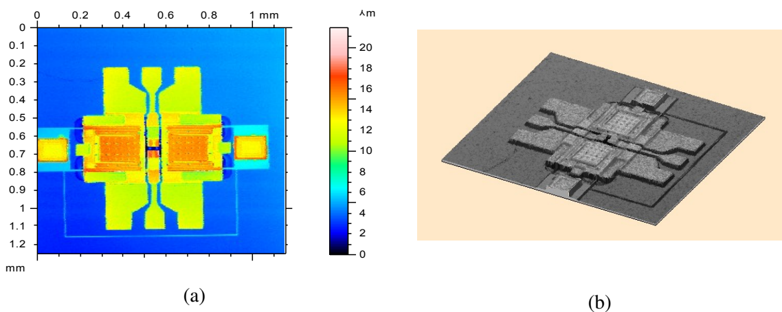
Figure III.25: (a) Microtopographie du MEMS série et (b) vue 3D
