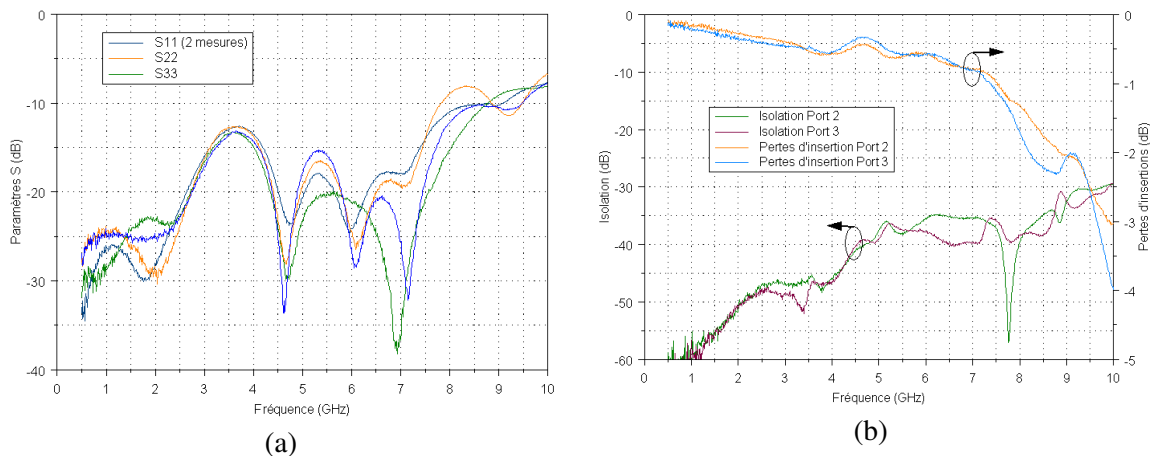
Figure III.4: (a) Adaptation (b) Pertes d'insertion en fonction de la fréquence
