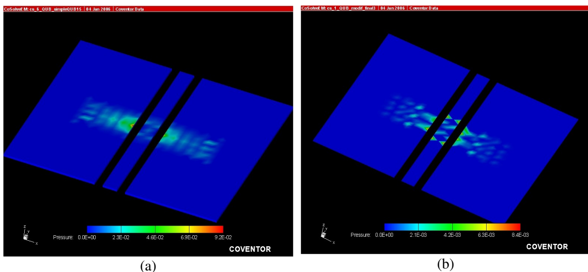
Figure III.13: Empreinte après commutation de la membrane pour la structure (a) 1 serpentins et (b) 1.5 serpentins
