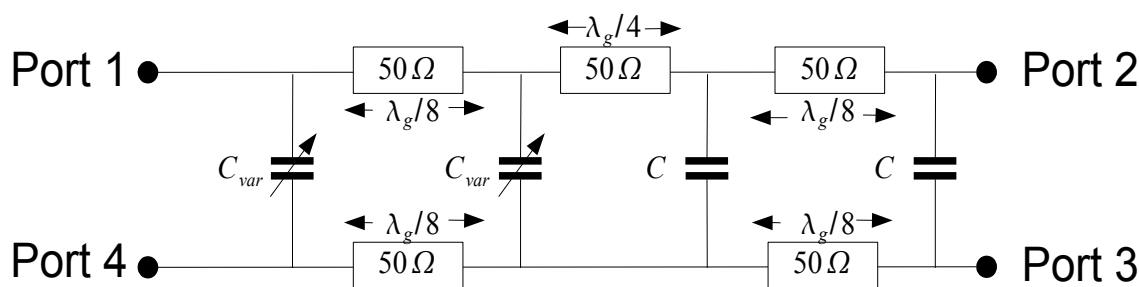
Figure V.15: Schéma final du déphaseur
