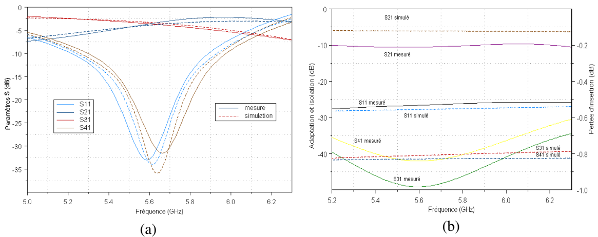
Figure IV.20: Paramètres Sij pour le coupleur avec capacités (a) et sans capacités(b)
