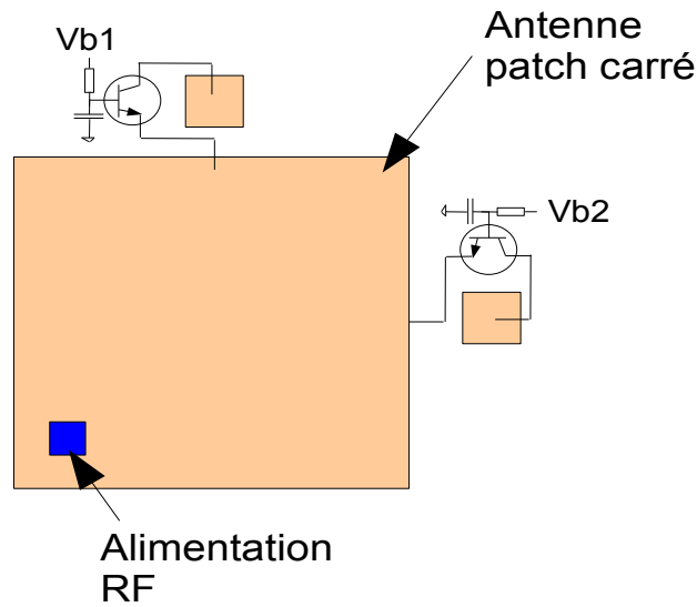
Figure II.48: Antenne chargée par des transistors bipolaires
