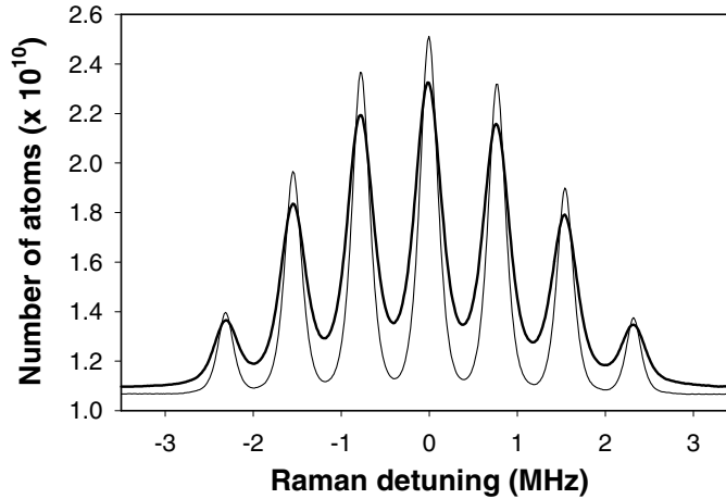
FIG. 3.8 : Flux d'atomes transférés en fonction du désaccord Raman pour une transition \pi contre-propagante. Les deux courbes correspondent aux deux jets.
