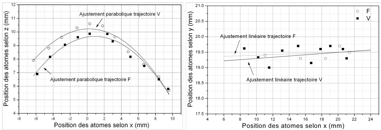
FIG. 3.15 : Trajectoires des deux nuages d'atomes au niveau de la zone interférométrique pour les deux nuages issus des sources F et V : à gauche dans le plan vertical ( OXZ ) et à droite dans le plan horizontal ( OXY ).
