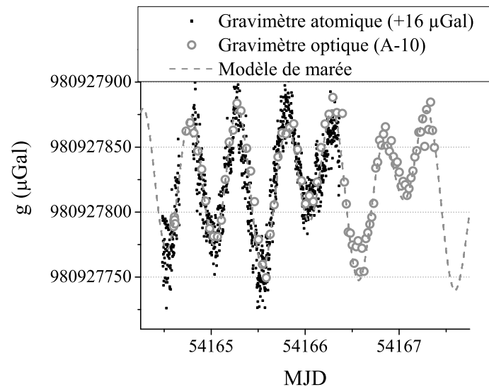
FIG. 4.12 : Marées luni-solaires de la gravité mesurées par le A10 de l'IPGP et le gravimètre du SYRTE (mesures décalées de 16 \mu\text{Gal} )
