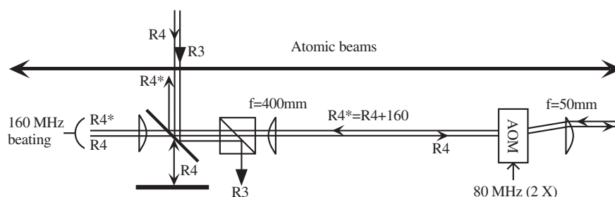
FIG. 3.7 : Schéma de principe de l'optique de rétro-réflexion de chaque paire de faisceaux lasers Raman.
