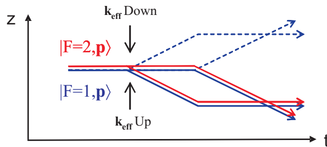
FIG. 4.10 : Trajectoires atomiques dans le référentiel en chute libre en fonction du temps. Renverser la direction de k_{\text{eff}} change la trajectoire moyenne des atomes. Par contre en changeant au préalable l'état interne, les trajectoires des deux interféromètres à \pm k_{\text{eff}} sont identiques, garantissant la réjection du gradient de champ magnétique.
