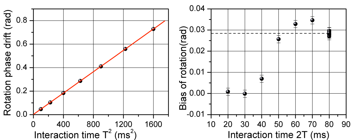
FIG. 3.23 : Variation du facteur d'échelle (gauche) et du biais (droite) en fonction de la durée T entre deux impulsions successives.
