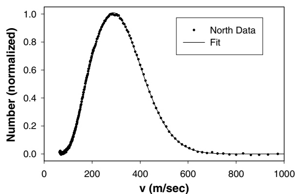
FIG. 3.4 : Distribution de la vitesse longitudinale de l'un des deux jets atomiques, mesurée par temps de vol.
