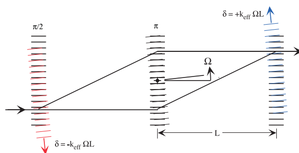
FIG. 3.9 : Dans un référentiel inertiel, la rotation apparaît comme un décalage de fréquence de signes opposés pour les deux impulsions \pi/2
