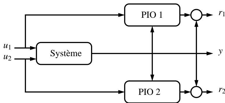
Figure 5.7 – Schéma de détection de défauts d'actionneurs
