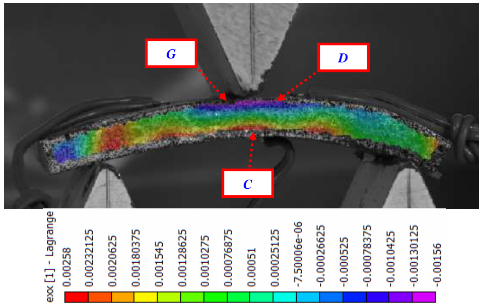
Figure 87: 69_08 EP 02 – V_o = 825,46 mm/min - Déformations longitudinales maximales Stéréocorrélation d'images
