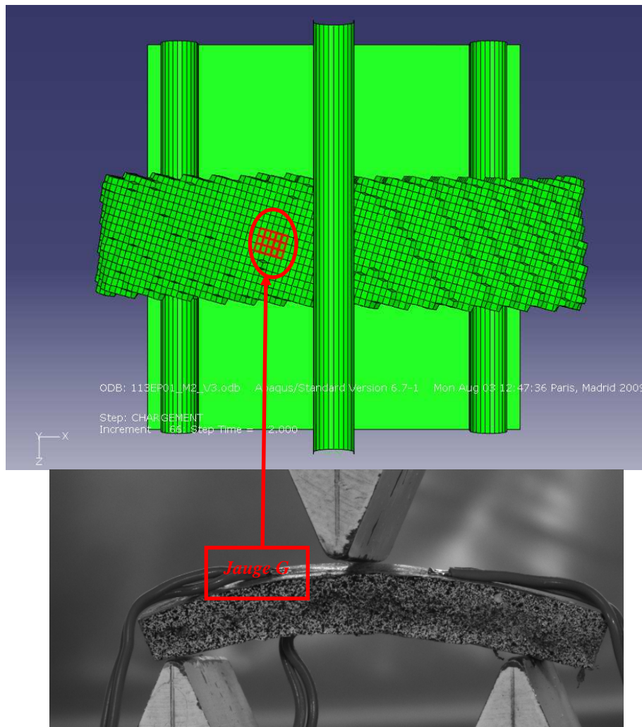
Figure 124: Eléments choisis pour le calcul des déformations – Epreuve 113_07 EP 01 - Jauge G
