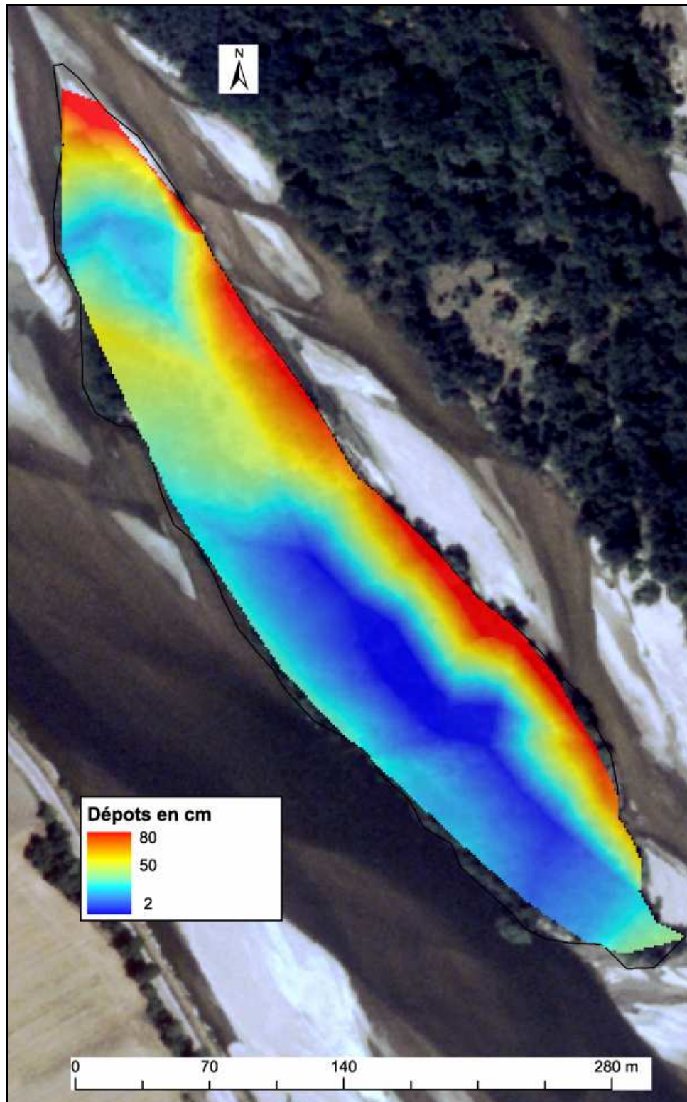
Figure 173 – Evaluation de la sédimentation sur une île jeune après la crue 5 (décembre 2003). Secteur des Loges, à l'aide de la méthode krigeage des points mesurés in situ.
