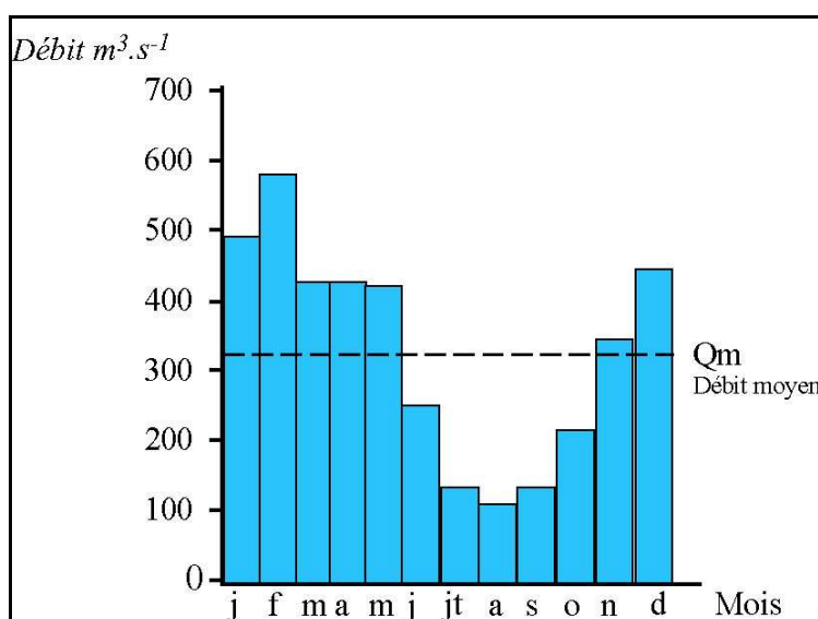
Figure 31 – Régime hydrologique de la Loire à la station de Givry (Cher).
