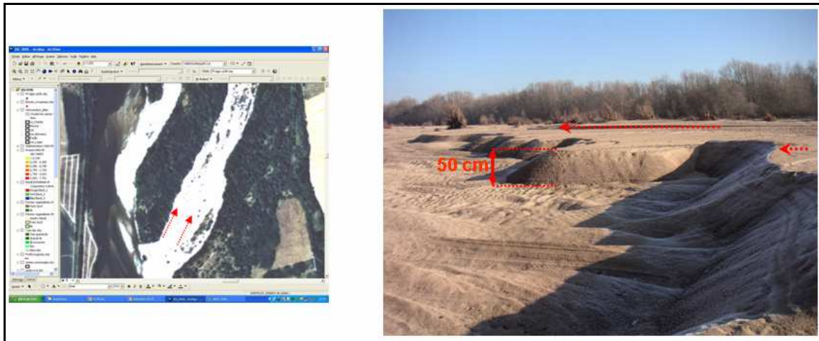
Photographie 33 – Sédimentation active dans les bras secondaires les plus longs.
