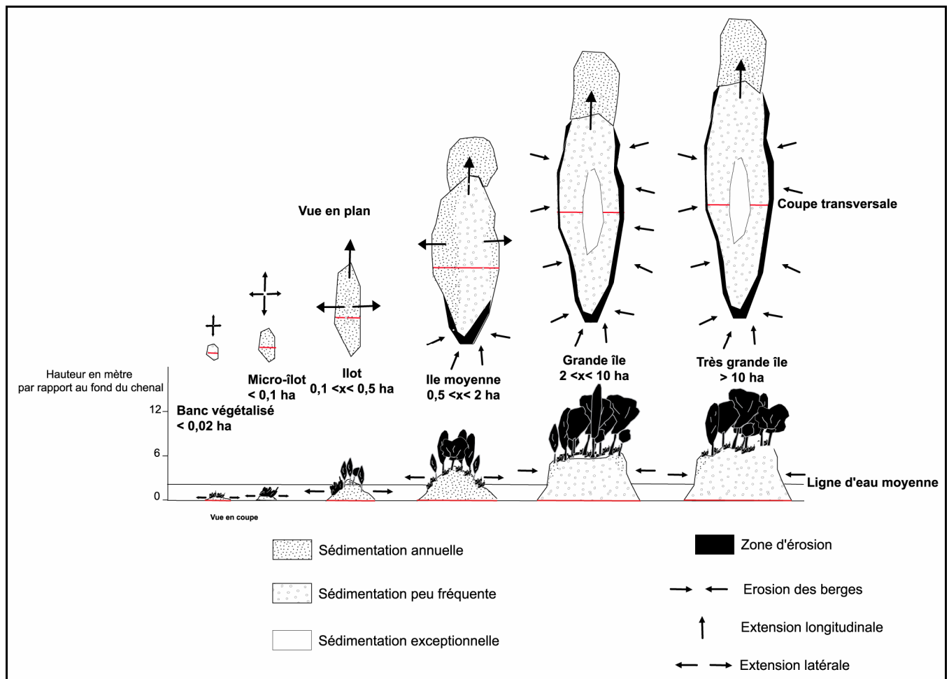
Figure 118 – Processus de sédimentation et d'érosion suivant les types d'îles et leur modèle d'évolution.
