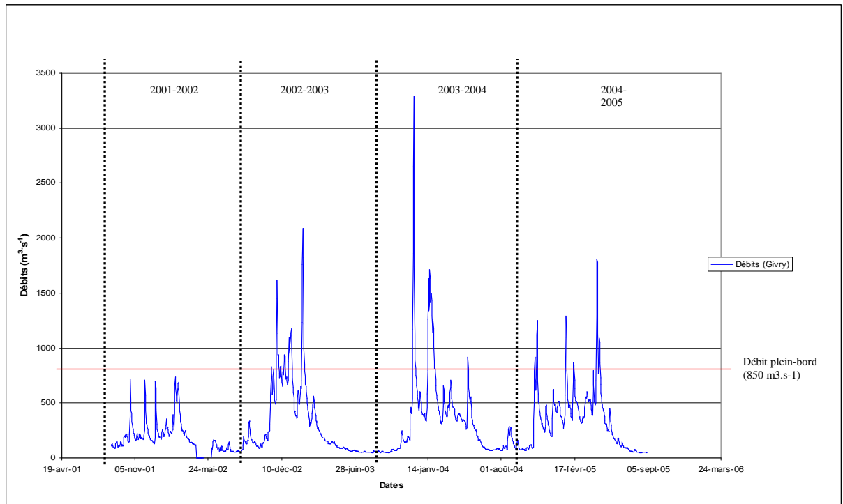
Figure 61 - Evolution des débits entre 2002 et 2005.
