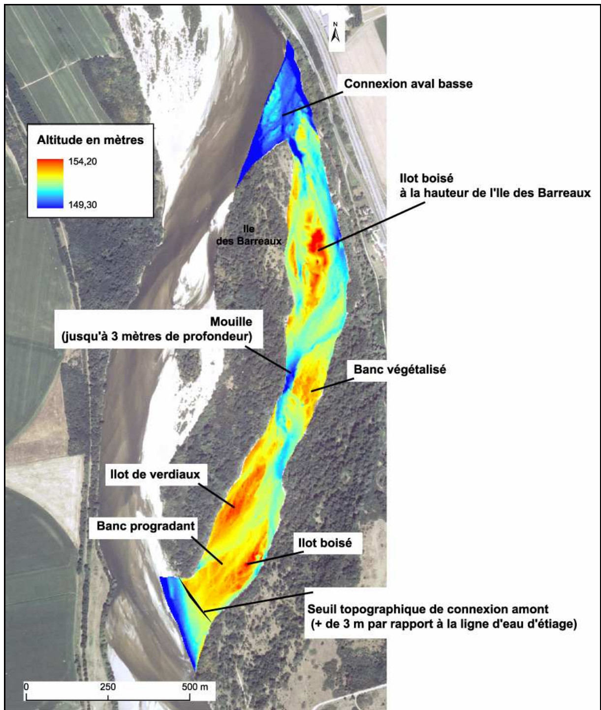
Figure 182 – Description géomorphologique de la modélisation du bras des Barreaux. Modélisation de la topographie à partir du LIDAR (DIREN-Centre).
