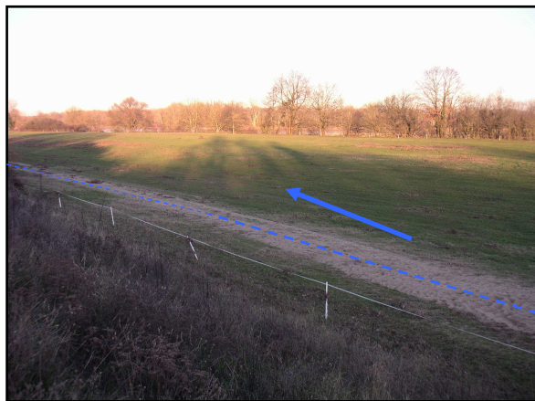
Photographie 32 – Ecoulements sur les francs-bords. Les écoulements les plus forts dans les francs-bords se sont localisés dans les anciens chenaux, aujourd'hui les parties basses : la sédimentation y est de l'ordre de 5 cm.
