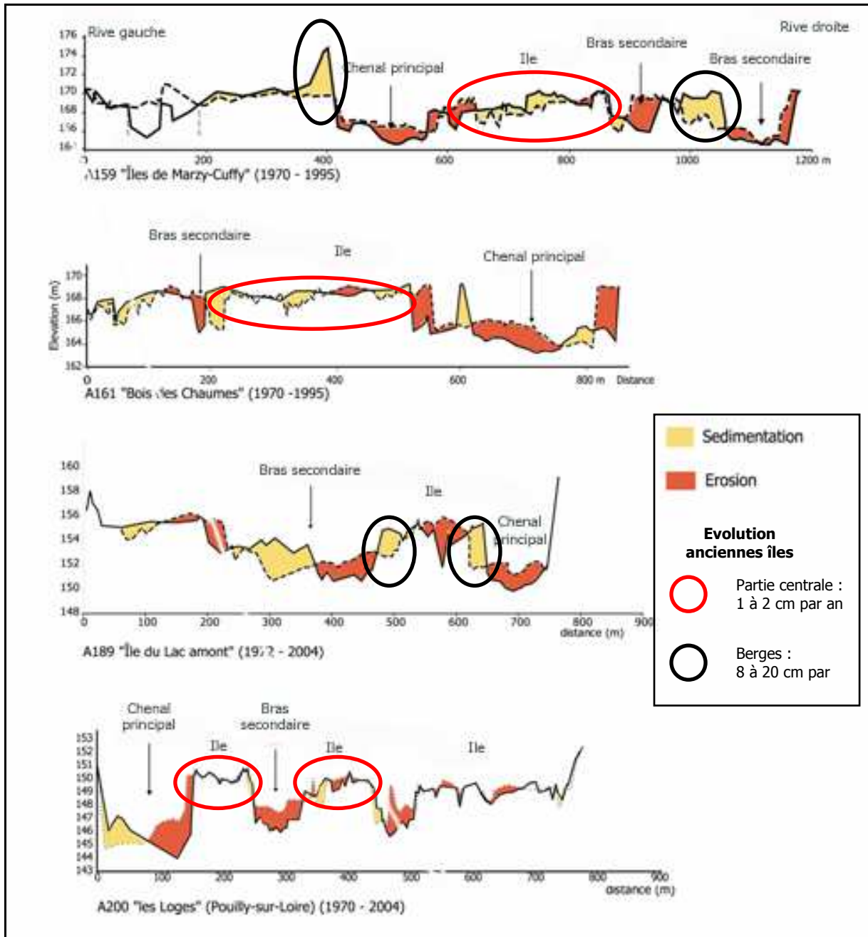
Figure 134 – Profils comparatifs des Sites Ateliers 1 et 3.
