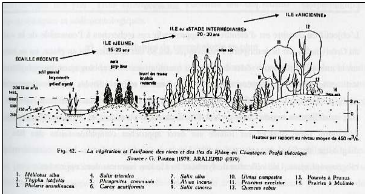
Figure 26 – Relation formes fluviales – végétation dans la vallée du Rhône.
