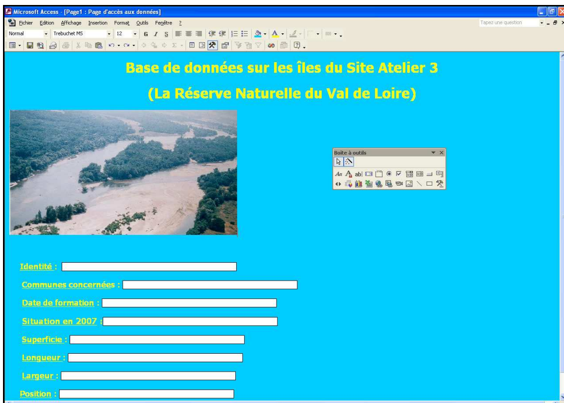
Figure 242 – Création d'une base de données « îles ».
