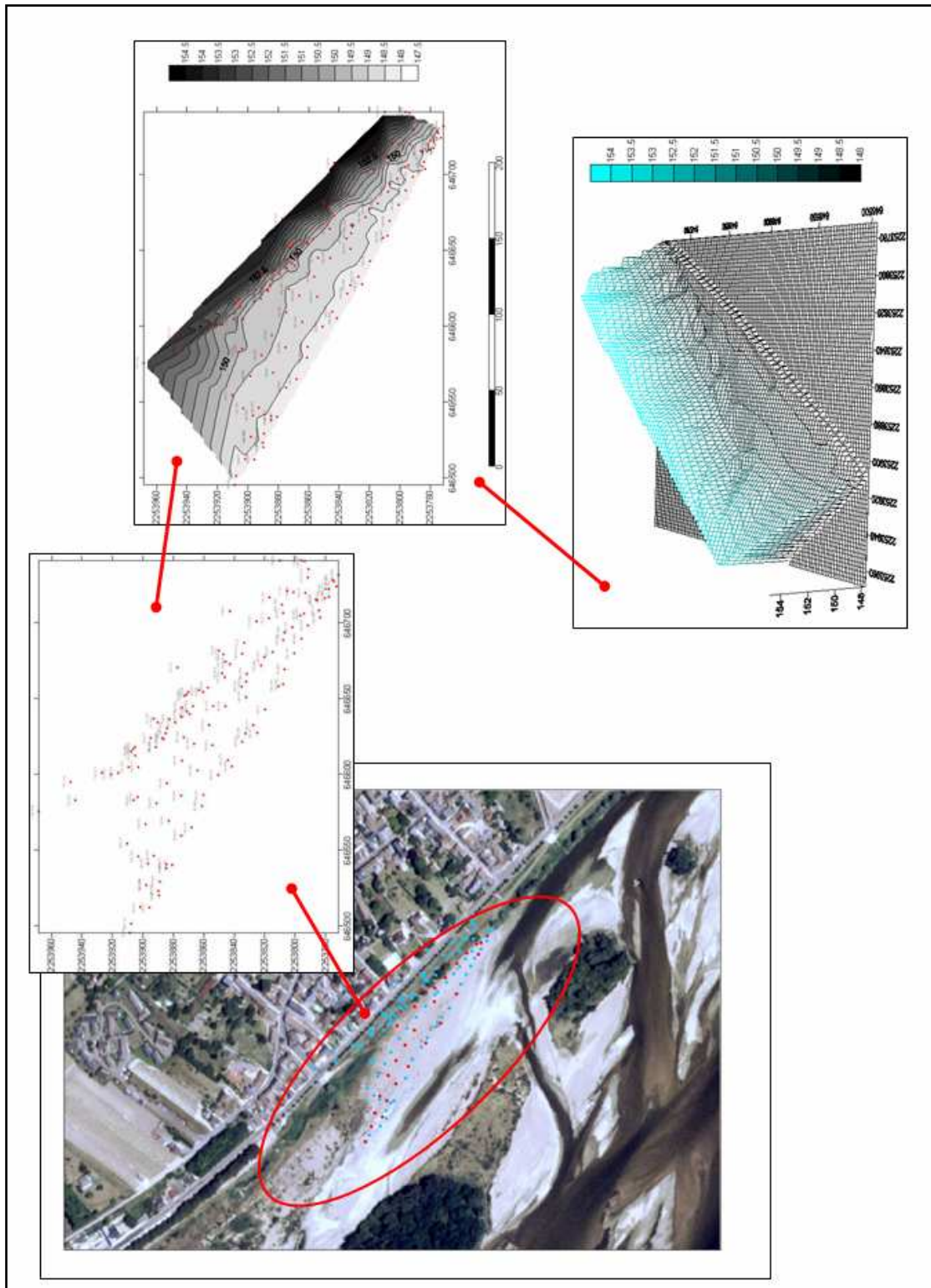
Figure 57 – Les grandes étapes des mesures topographiques depuis les levés de terrain jusqu'à la création des MNT.
