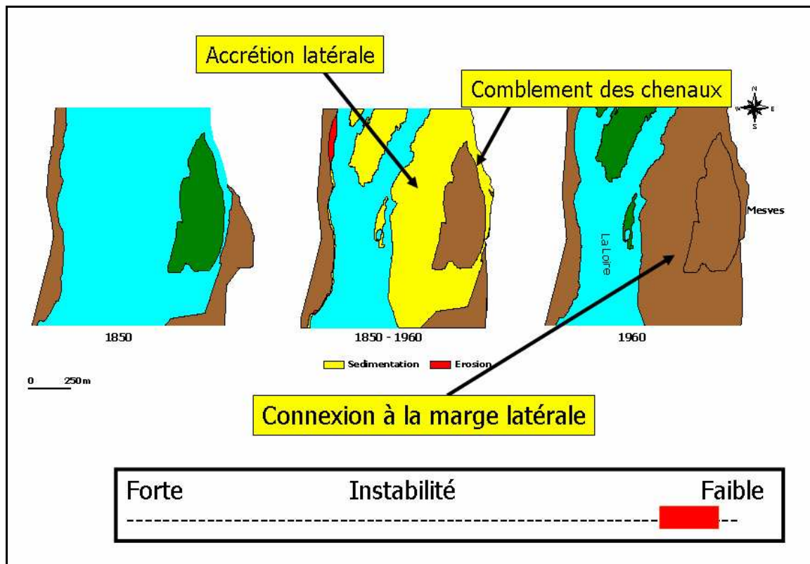
Figure 115 – Le rattachement d'une île à un franc-bord représente le stade définitif de la stabilisation. Ces îles quittent alors le monde des formes insulaires pour rejoindre celui des franc-bords, beaucoup plus stables dans un système en anabranché comme la Loire des îles.
