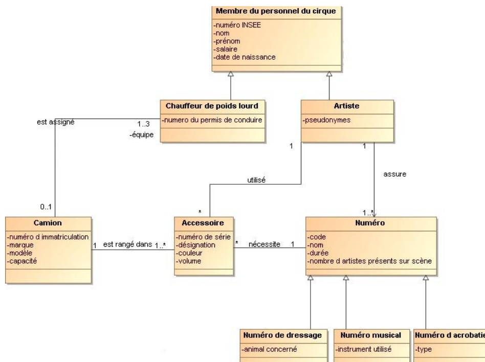
Figure 66 : Enoncé et diagramme de référence de l'exercice « Cirque » (avec MagicDraw UML)
