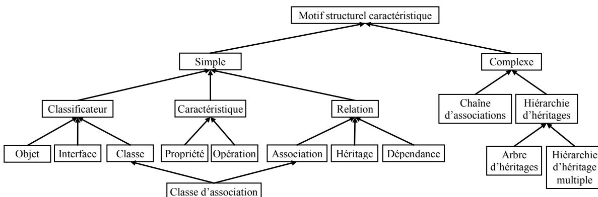
Figure 37 : Motifs structurels caractéristiques des diagrammes de classes UML 2
