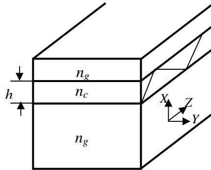
Figure 3. 2 - Guide plan à saut d'indice
