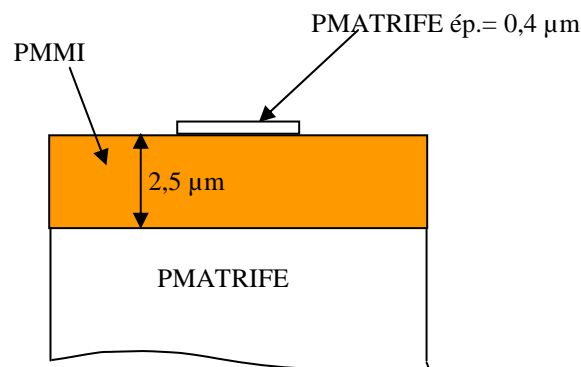
Figure 4. 73 - Architecture du SLWG réalisé en polymères classiques
