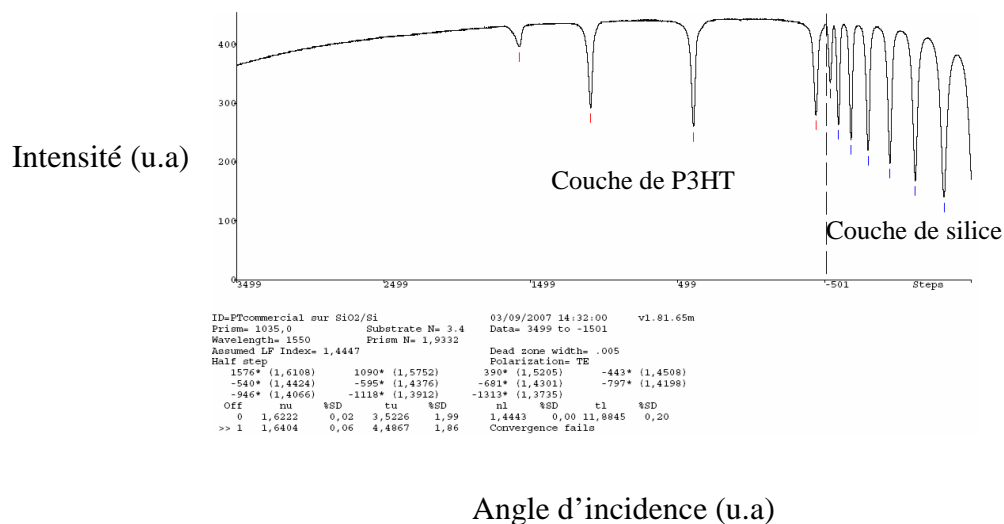
Figure 4. 54 - Spectre m-lines d'un film P3HT ( 100\text{g.l}^{-1} ) déposé sur un substrat de silice
