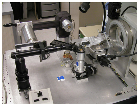
Figure B.2 - Photo du banc expérimental de la mesure en champ lointain
