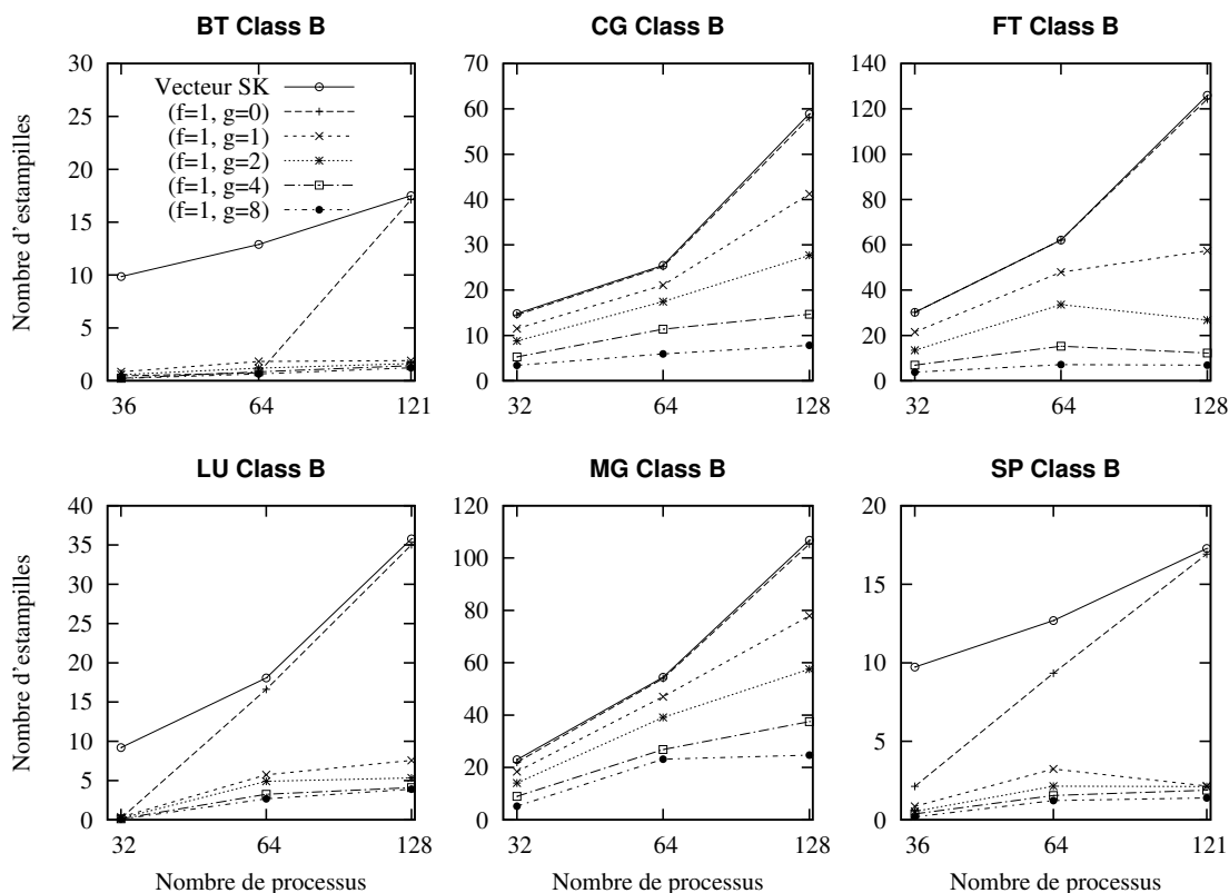
FIG. 5.30 – Influence du degré de diffusion sur la quantité de données attachées sur les messages de l'application avec un enregistreur d'événements distribué
