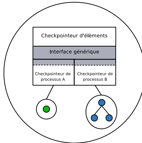
FIG. 3.3 – Utilisation de plusieurs checkpointeurs de processus par XtremGCP
