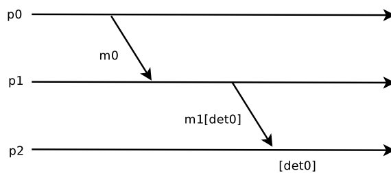
FIG. 5.6 – Protocole à enregistrement de messages causal
