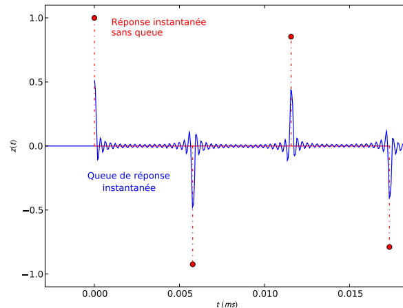
Figure 2.13 – Réponse impulsionnelle d'un cylindre (modèle de Raman, marqueurs \circ et pointillés) et son approximation modale (20 modes pris en compte, trait plein).
