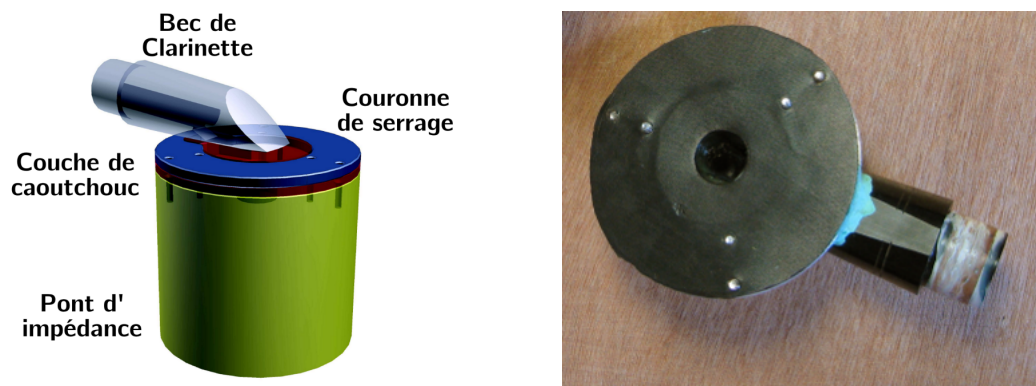
Figure 5.5 – Schéma et photo de l'interface bec-captur d'impédance.
