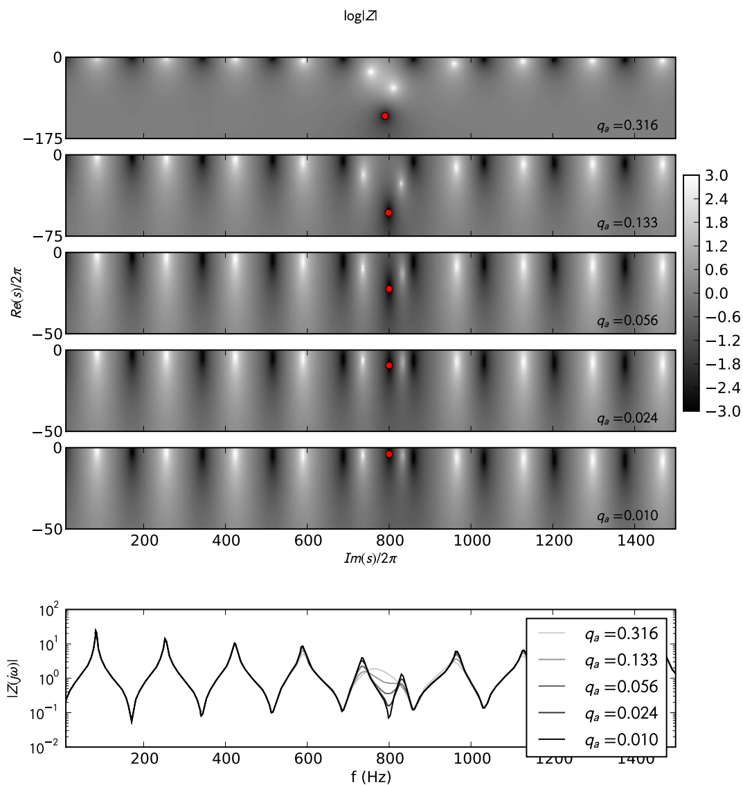
Figure 2.8 – Effet du débit d'anche sur la position des pôles de l'impédance. Variation de l'amortissement d'anche. Cylindre de 1m, anche ( f_a = 800 Hz, \Delta l_a = 10 mm). Le marqueur représente la position du pôle de la dynamique d'anche.
