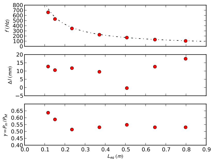
Figure 5.12 – Seuils estimés avec la lèvre de glycérine pour une ouverture au repos de 5.2 \text{ mm}^2 , une raideur à basses pressions de 6.1 \text{ kPa/mm}^2 .
