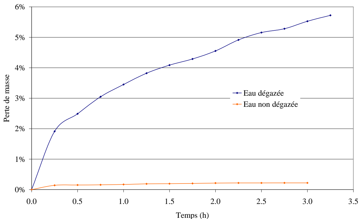
Figure 50 : Comparaison de l'érosion de compacts 10 % avec de l'eau du robinet dégazée, ou non ( T = (28 \pm 4)^\circ\text{C} )
