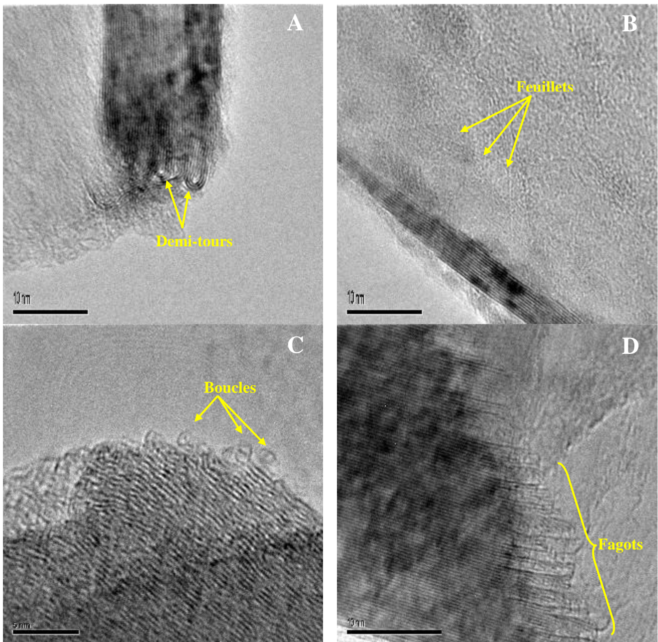
Figure 66 : Mise en évidence de structures exotiques. A et B : échantillon traité à 20 W/cm 2 ; C et D : échantillon traité à 30 W/cm 2 .
