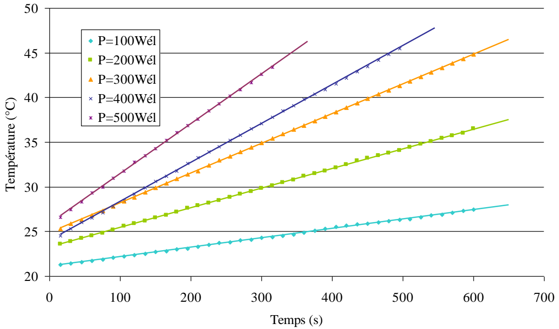
Figure 56 : Échauffement de l'eau ultrapure dégazée pour cinq puissances pour la calibration de la puissance ultrasonore de la sonotrode 10x55 mm
