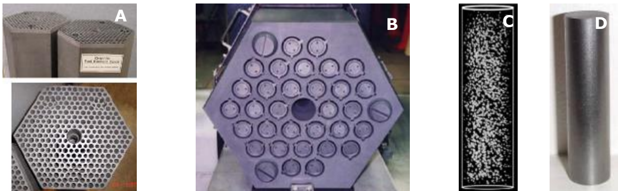
Figure 8 : A : Éléments de combustible en graphite de FSV [24] ; B : Élément de combustible fabriqué par Toyo Tanso [29] ; C : Reconstitution 3D d'un compact avec les particules TRISO [46] ; D : Photo d'un compact fourni par CERCA.
