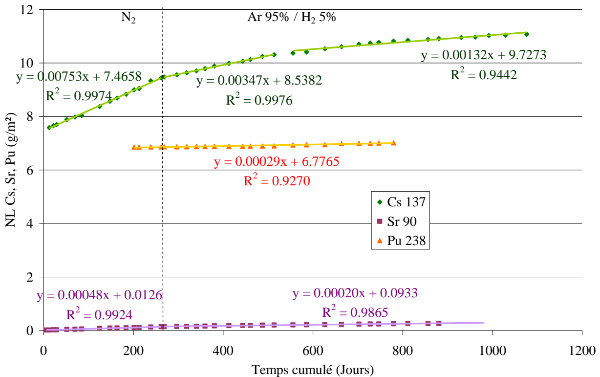
Figure 115 : Pertes de masses normalisées de ^{137}\text{Cs} , ^{90}\text{Sr} et ^{238}\text{Pu}
