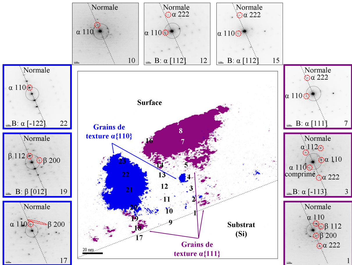
FIG. III.14 – Superposition des champs sombres associés aux plans \alpha -W \{110\} et \alpha -W \{111\} de texture, localisation des nanodiffraction et clichés caractéristiques (négatifs des originaux) associés.
