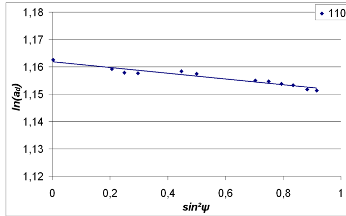
(b) W/Cu 3/1
