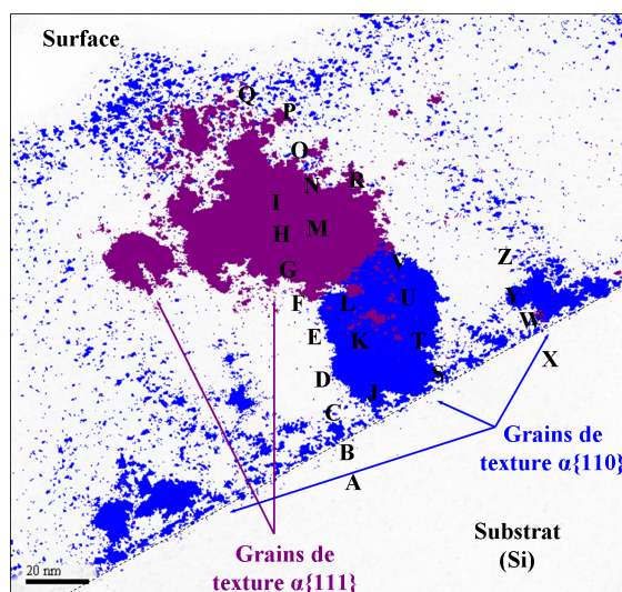
(b) Superposition des champs sombres associés aux plans \alpha\text{-W}\{110\} et \alpha\text{-W}\{111\} de texture
