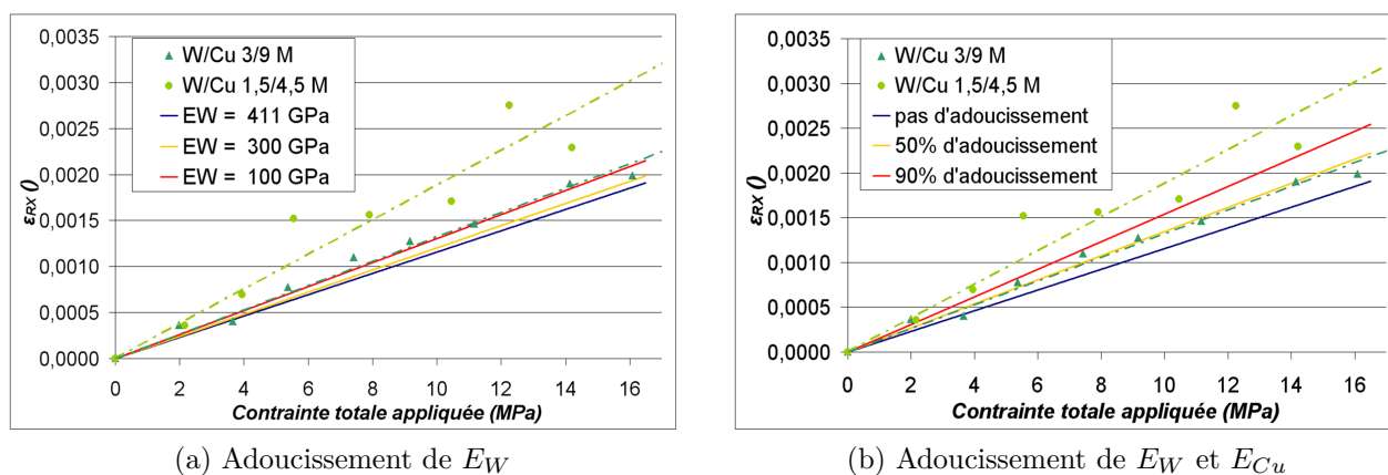
FIG. IV.22 – Évolution de la déformation élastique des sous-couches de tungstène au sein des deux multicouches W/Cu 3/9 M et W/Cu 1,5/4,5 M ( \phi=0^\circ , \psi=58,5^\circ ) en fonction de la contrainte appliquée à l'ensemble film-substrat. Les lignes en pointillé représentent la régression linéaire des déformations et les lignes pleines, les déformations calculées par homogénéisation ( \phi=0^\circ , \psi=60^\circ ) en considérant un adoucissement du module d'Young du tungstène seul (a) ou de chacune des phases (b).
