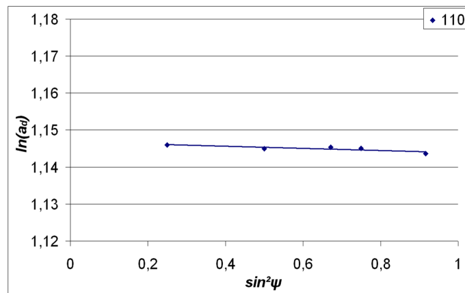
(c) W/Cu 1,5/1
