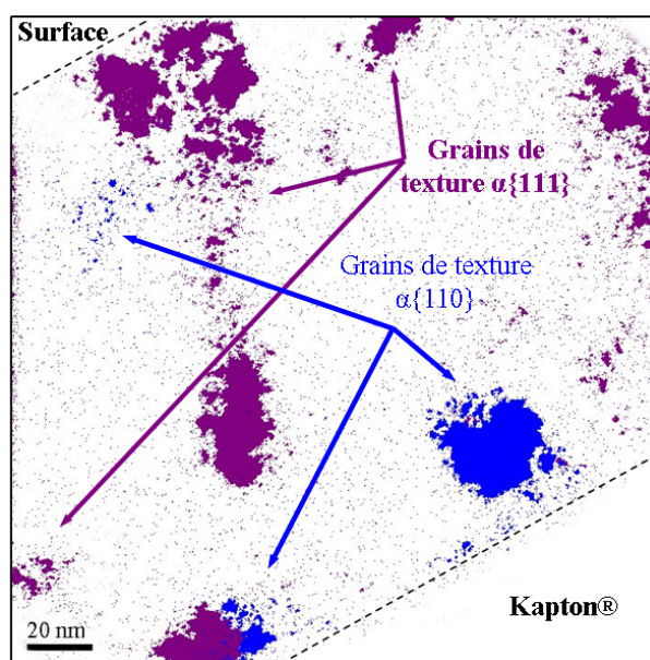
FIG. III.17 – Superposition des champs sombres sur les taches de diffraction \alpha\text{-W}\{110\} et \alpha\text{-W}\{222\} de l'échantillon W/W 2/2 sur substrat de Kapton®.
