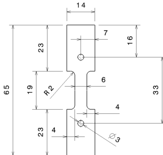
FIG. II.5 – Géométrie des éprouvettes de traction utilisées (unités exprimées en mm).
