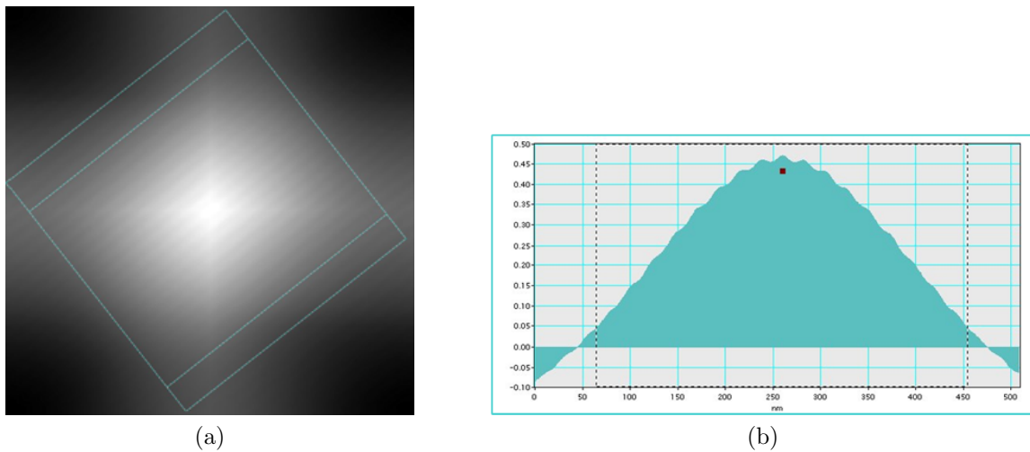
FIG. IV.4 – (a) Auto-corrélation de l'image en champ clair de la figure IV.3 et (b) profil d'intensité associé.
