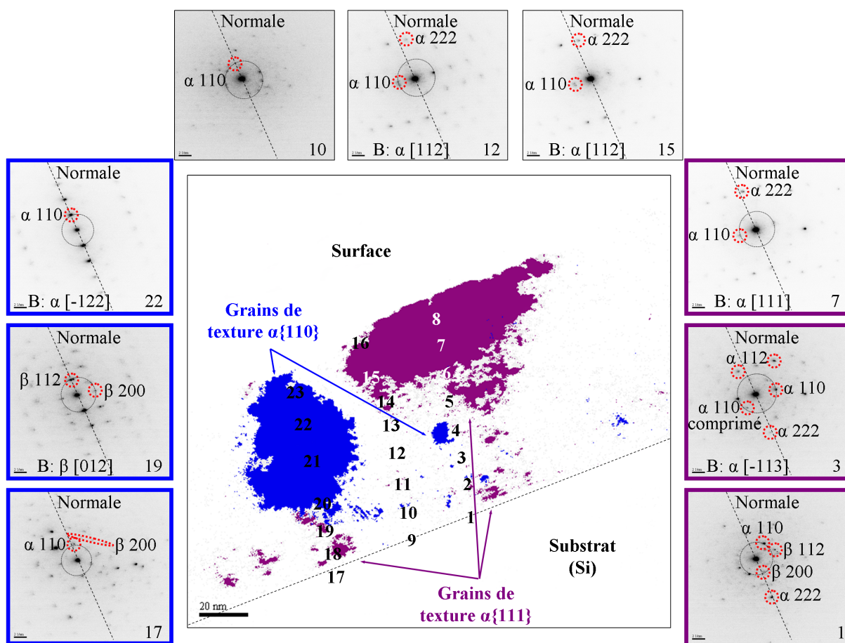
FIG. III.14 – Superposition des champs sombres associés aux plans \alpha -W \{110\} et \alpha -W \{111\} de texture, localisation des nanodiffraction et clichés caractéristiques (négatifs des originaux) associés.
