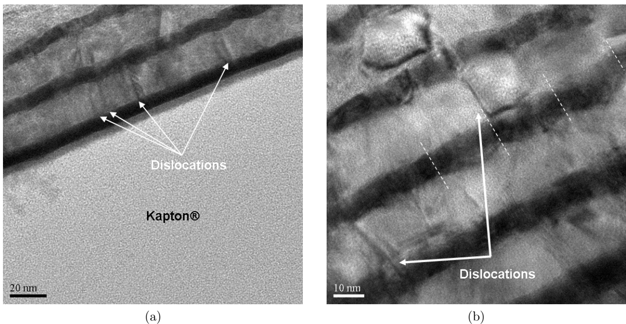
FIG. IV.39 – Images haute-résolution de l'interface film-substrat de l'échantillon W/Cu 6/18 MP en deux zones différentes.
