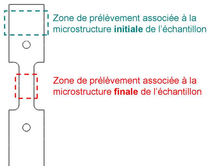
FIG. IV.26 – Zones de prélèvement des spécimens utilisés lors de la préparation des lamelles de microscopie électronique en transmission témoignant de la microstructure de l'échantillon avant et après traction au delà de la limite d'élasticité.
