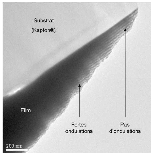
FIG. IV.29 – Image en champ clair de l'échantillon W/Cu 6/18 avant traction au delà de la limite d'élasticité.
