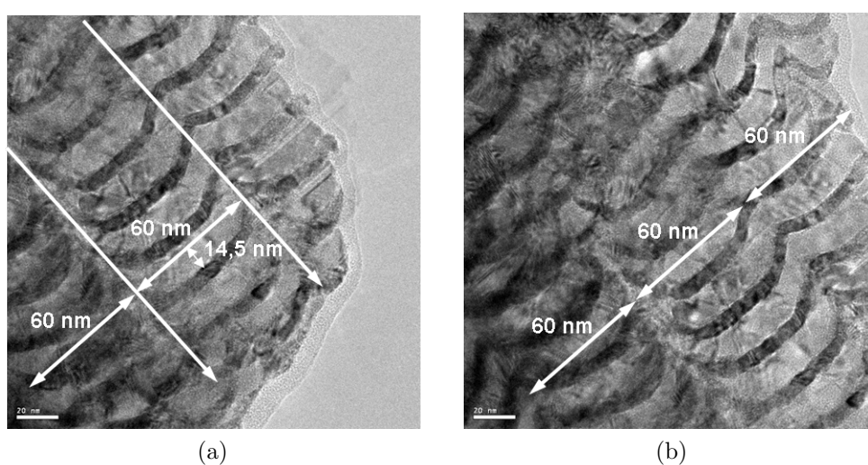
FIG. E.3 – Images en champs clair de deux zones ((a) et (b)) de l'échantillon W/Cu 6/18 M sur silicium où l'amplitude de l'oscillation des couches est maximale.
