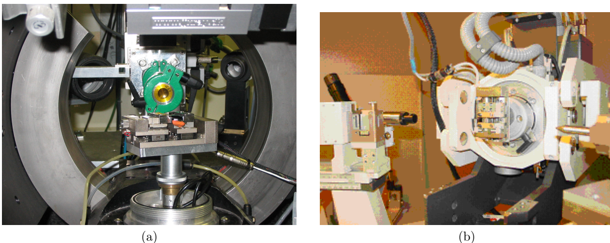
FIG. II.11 – Machine de traction disposée sur (a) le diffractomètre 7-cercles de l'ESRF et (b) le diffractomètre 4-cercles du laboratoire PhyMat.
