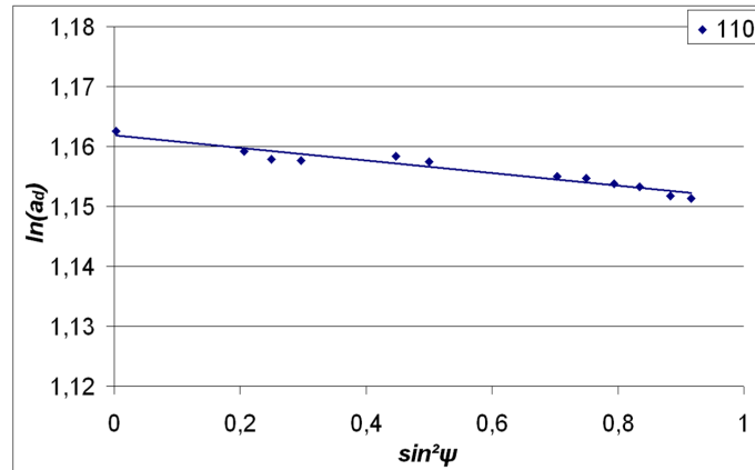
(b) W/Cu 3/1
