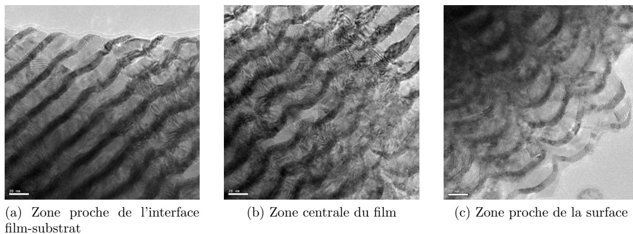
FIG. E.2 – Pointés d'images haute-résolution de l'interface film-substrat vers la surface sur l'échantillon W/Cu 6/18 M sur silicium.
