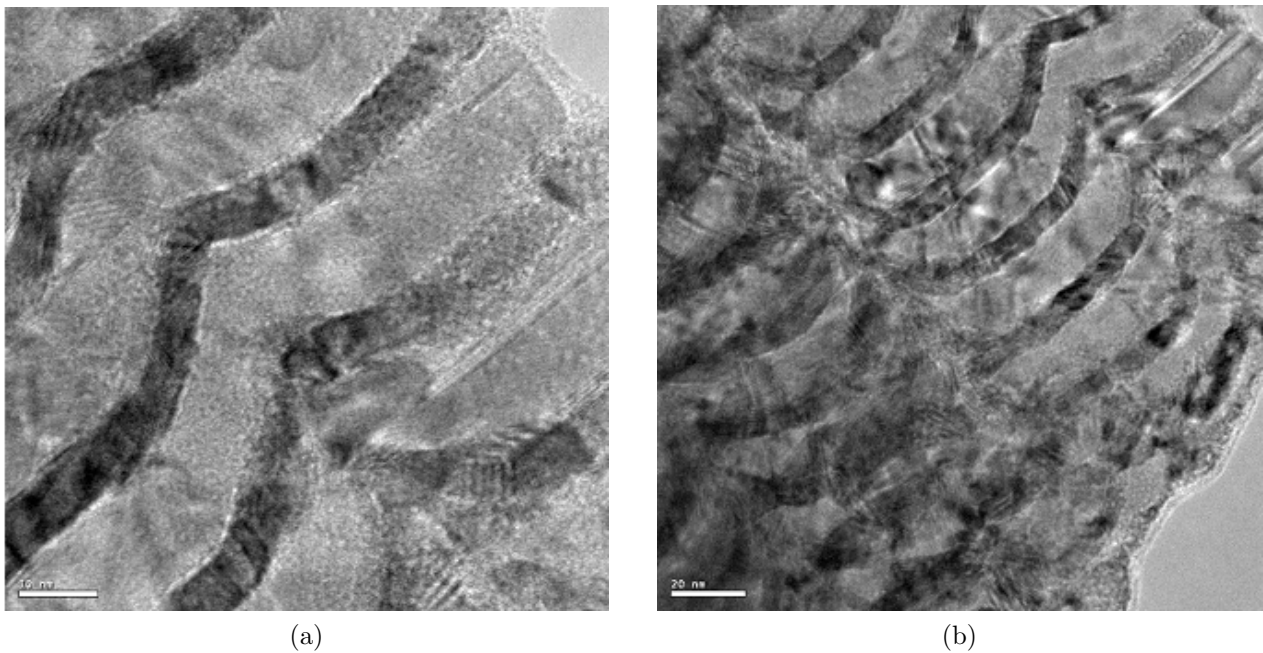
FIG. E.4 – Images haute-résolution des zones de forte courbure des couches sur l'échantillon W/Cu 6/18 M sur silicium.
