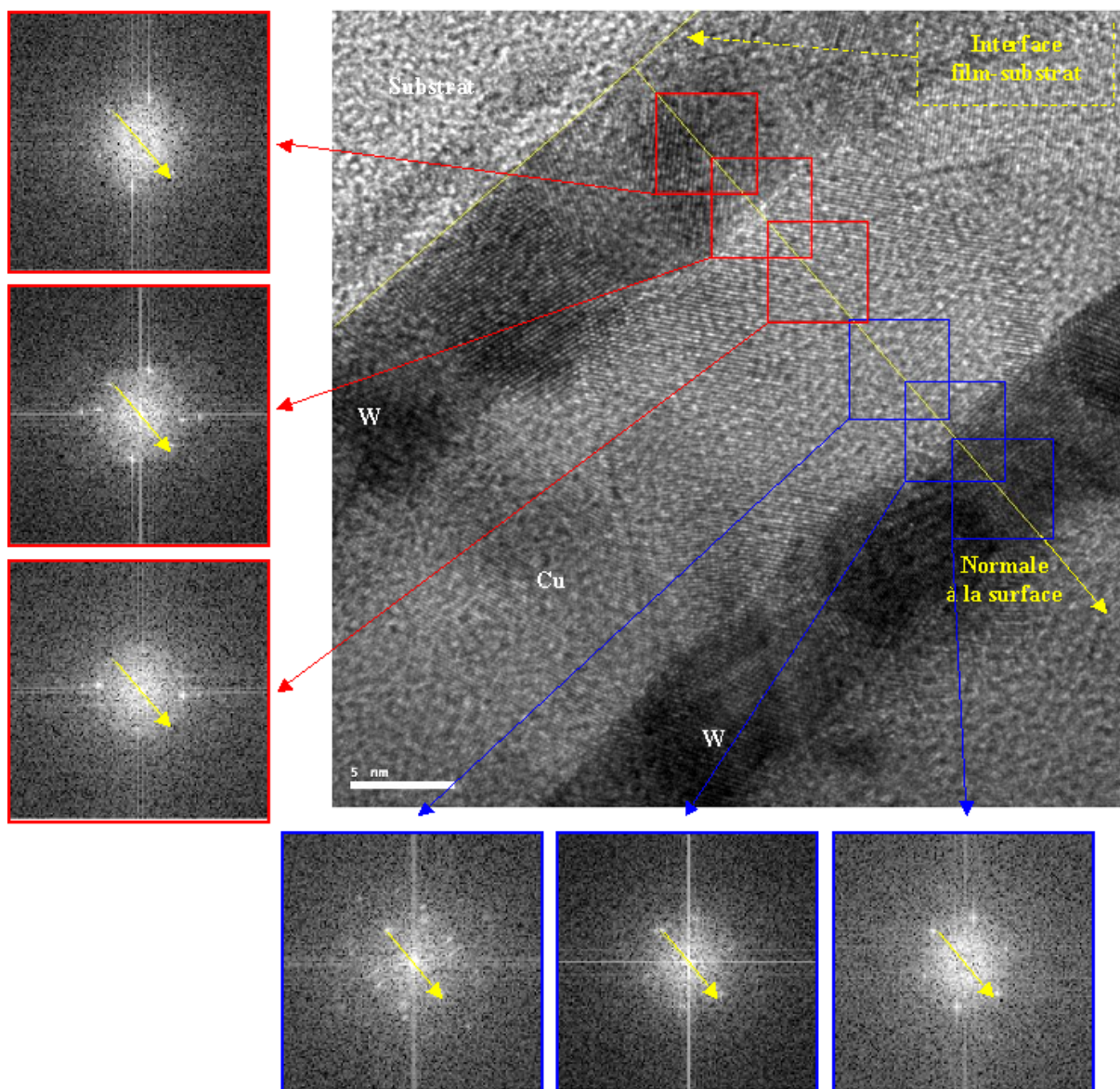
FIG. IV.5 – Analyse de l'orientation cristalline selon la direction de croissance des couches ou normale à l'interface film-substrat (indiquée par les flèches jaunes) par transformées de Fourier réduites d'une image haute-résolution réalisée dans une zone proche de l'interface film-substrat.
