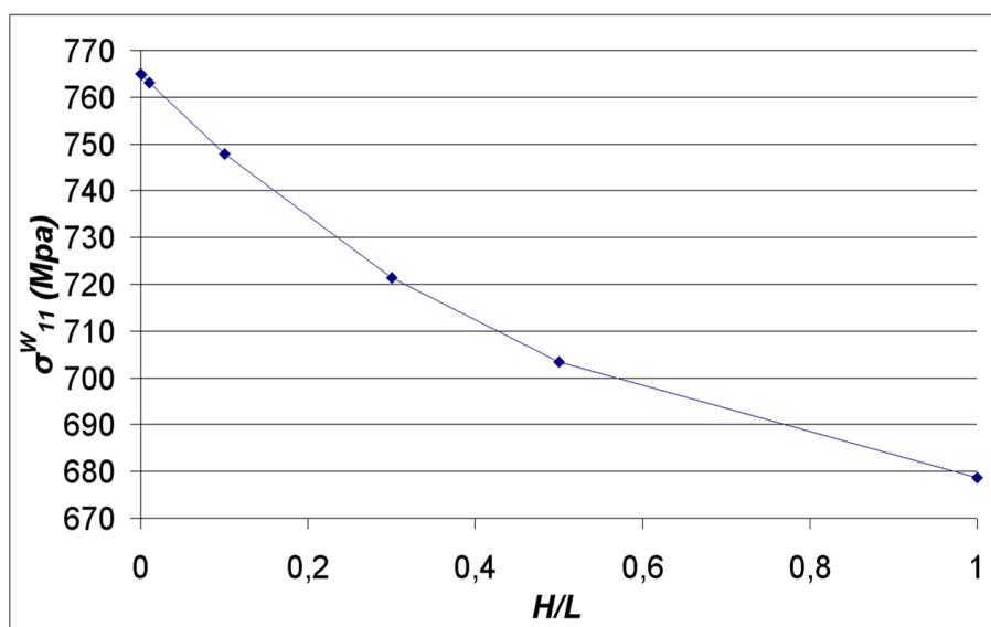
FIG. III.24 – Influence du rapport H/L des inclusions de cuivre sur la contrainte transmise dans la matrice de tungstène.
