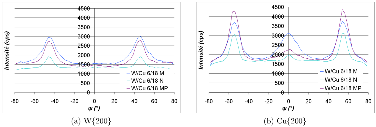
FIG. IV.24 – Superposition des (a) \psi -scan W{200} et (b) Cu{200} des échantillons W/Cu 6/18 M, W/Cu 6/18 MP et W/Cu 6/18 I.
