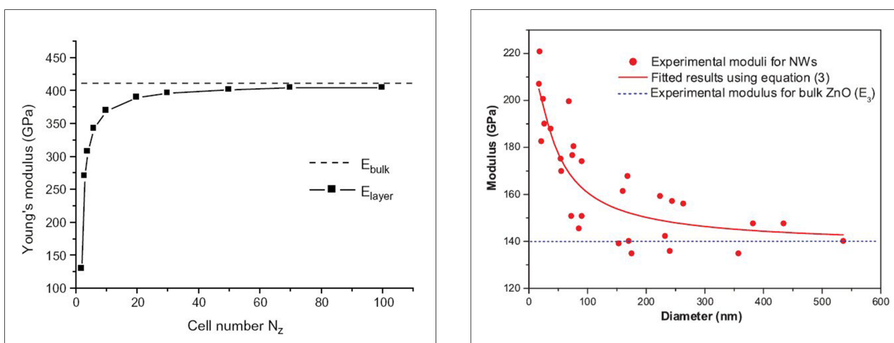
(a) Évolution du module d'Young d'un film de W monocristallin en fonction du nombre de mailles cristallines (épaisseur du film) [27].
