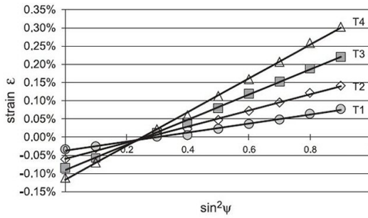
(a) Déformation d'un film polycristallin de W en fonction de \sin^2\psi pour la famille de plans 211. La charge appliquée est croissante de T1 à T4 [72].
