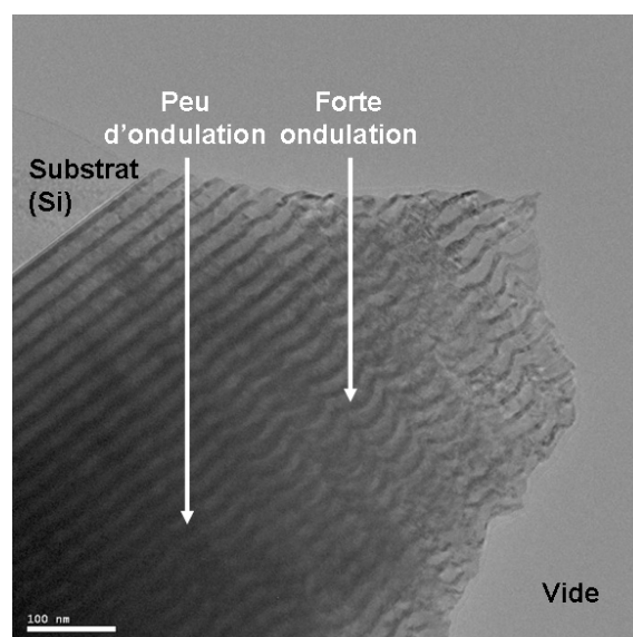
FIG. E.1 – Vue d'ensemble du film W/Cu 6/18 M sur substrat de silicium en champ clair.
