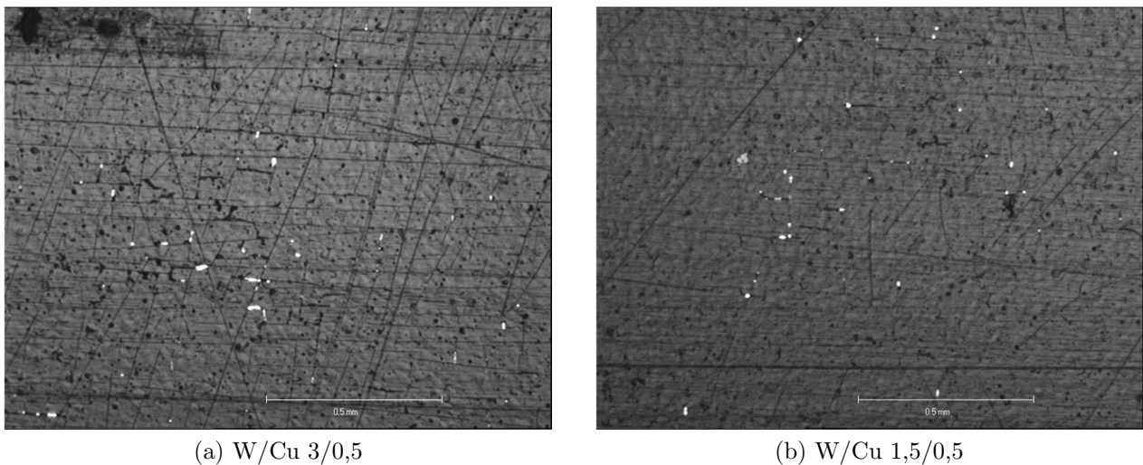
FIG. III.27 – Observation par microscopie optique de la zone d'interaction avec le faisceau X sur les films (a) W/Cu 3/0,5 et (b) W/Cu 1,5/0,5.
