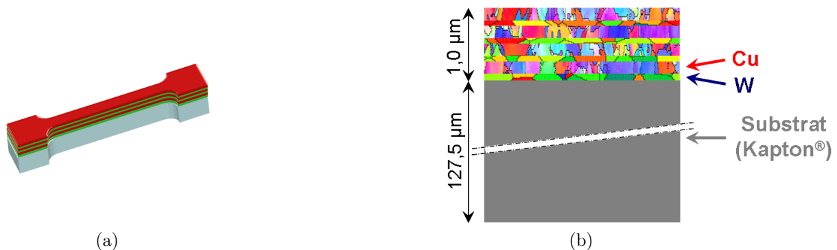
FIG. D.1 – (a) Éprouvette de traction et (b) vue en coupe de sa modélisation
