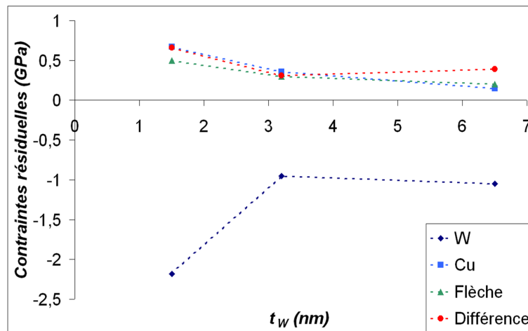
FIG. C.6 – Évolution des contraintes résiduelles dans les couches de tungstène \alpha et de cuivre des composites lamellaires, en fonction de l'épaisseur de la couche de tungstène.
