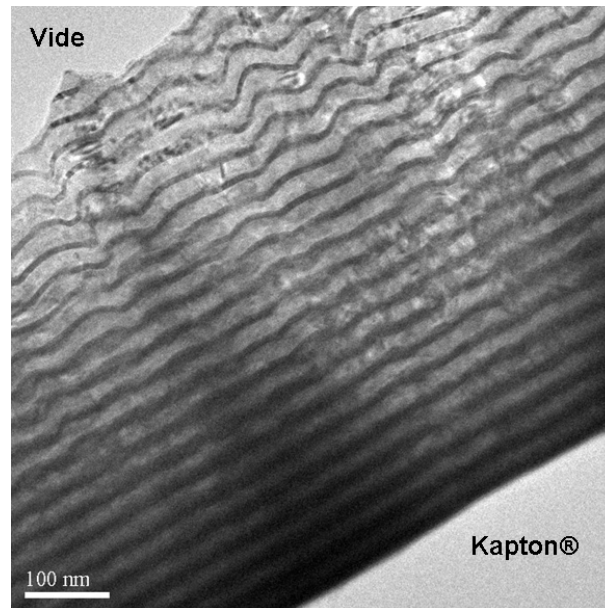
FIG. IV.41 – Image en champ clair d'une zone de l'échantillon W/Cu 6/18 MP présentant le film mince dans sa totalité.
