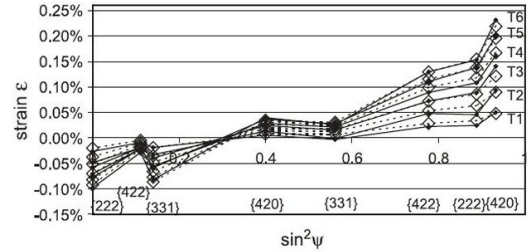
(b) Déformation d'un film polycristallin d'Au texturé 111 en fonction de \sin^2\psi . La charge appliquée est croissante de T1 à T5 [59].
