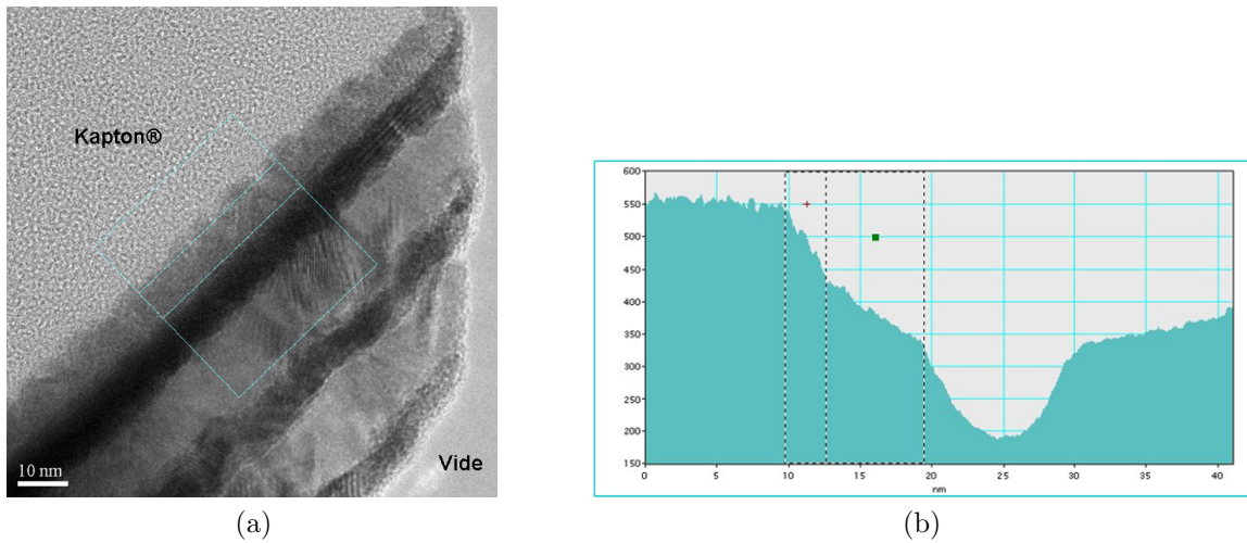
FIG. IV.11 – (a) Image en champ clair de l'interface film-Kapton ® et (b) profil d'intensité associé.
