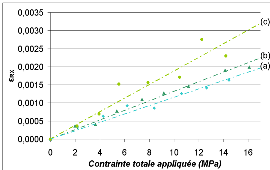
FIG. IV.18 – Évolution de la déformation élastique des sous-couches de tungstène au sein des trois composites lamellaires selon la direction longitudinale ( \phi=0^\circ ) en \psi=58,5^\circ en fonction de la contrainte appliquée à l'ensemble film-substrat : (a) W/Cu 6/18 M, (b) W/Cu 3/9 M et (c) W/Cu 1,5/4,5 M.
