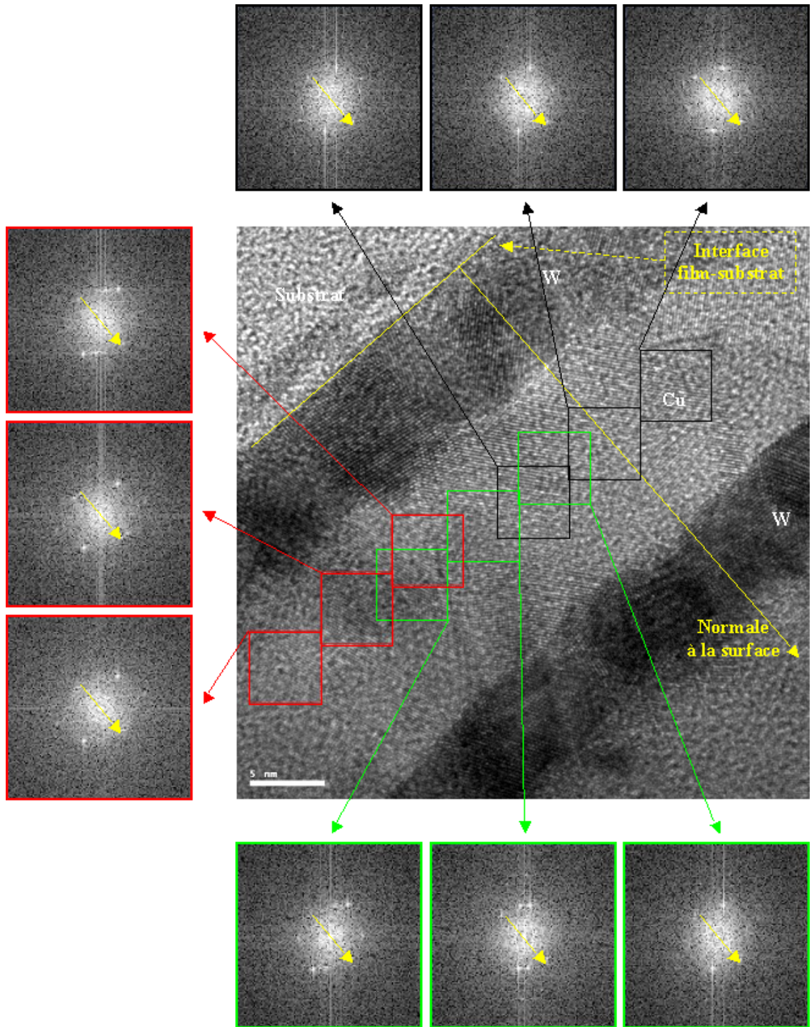
FIG. IV.7 – Analyse de l'orientation cristalline dans le plan des couches de cuivre par transformées de Fourier réduites d'une image haute-résolution réalisée dans une zone proche de l'interface film-substrat. Les flèches jaunes indiquent la normale à l'interface film-substrat.
