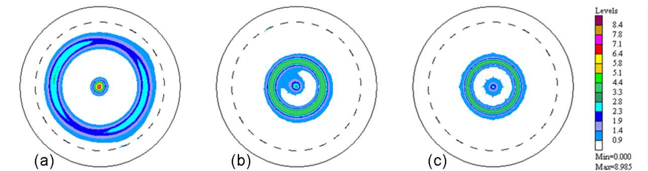
FIG. III.9 – Figures de pôles réalisées sur le pic \alpha -W{110} de chacun des échantillons : (a) W/Cu 3/1, (b) W/Cu 3/0,5 et (c) W/W 3/3.
