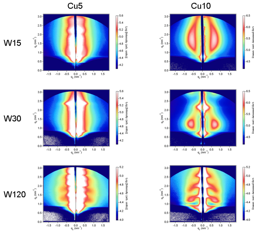
FIG. A.2 – Diagrammes 2D de diffusion centrale en incidence rasante. Les épaisseurs nominales e dans W_e et Cu_e sont données en Angström.
