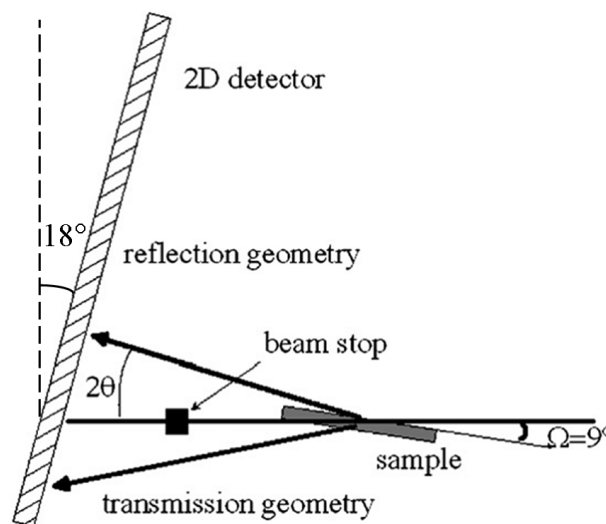
FIG. IV.16 – Configuration géométrique des expériences de diffraction de l'ALS.
