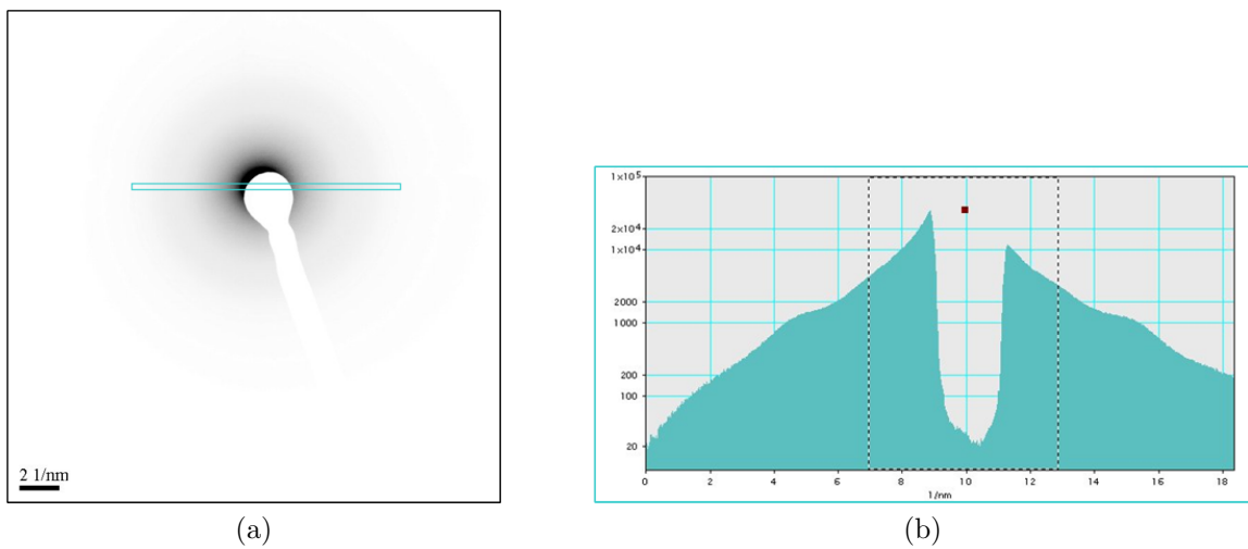
FIG. IV.12 – (a) Cliché de diffraction électronique réalisé sur Kapton ® (négatif) et (b) profil d'intensité radial associé.
