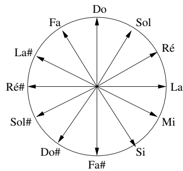
FIG. 2.3 – Le cercle des quintes, avec les vecteurs unité de chacune des clés.
