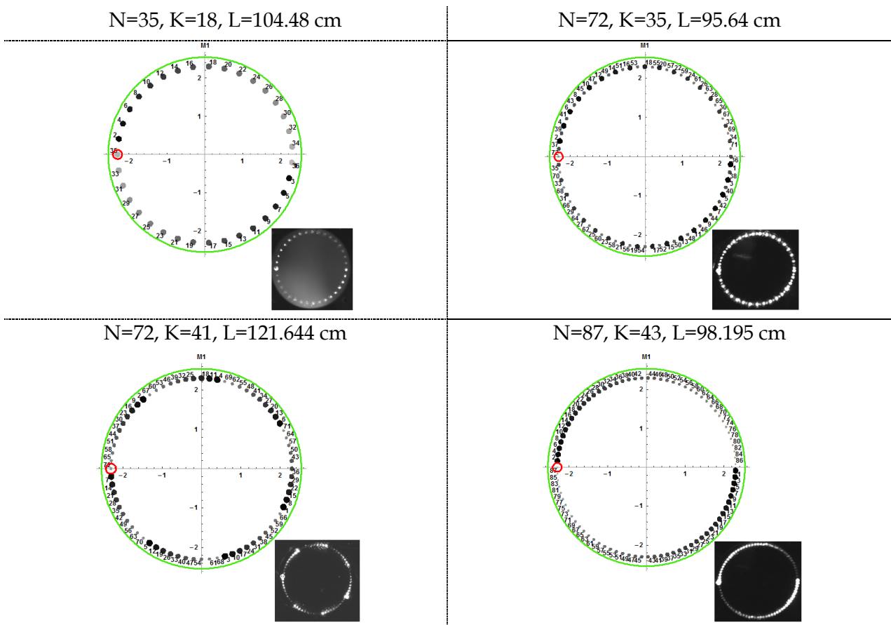
Figure 6.5 : Exemple de quelques trajectoires circulaires typiques calculées et observées pour différents couples de valeurs réentrantés (N, K) . Les intensités des taches d'impacts simulées, aussi bien que leur taille, sont proportionnelles à l'ordre de la réflexion. La première égale les propriétés d'un faisceau mode matché sur le mode fondamental de la cavité où le critère de 99% de son intensité transverse est pris en compte.
