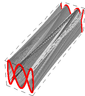
Figure 5.17 : Simulation de profils 3D de trajectoires de faisceau mettant en évidence la symétrie de révolution autour du profil dit en « X et en O » caractérisé par un couple de valeurs réentrantes (N,K_x,K_y)=(1002,250,251) et les injections initiales ad hoc pour garantir respectivement le cercle sur M_1 et la croix sur M_2 (cf. section 5.1.1.3.2).
