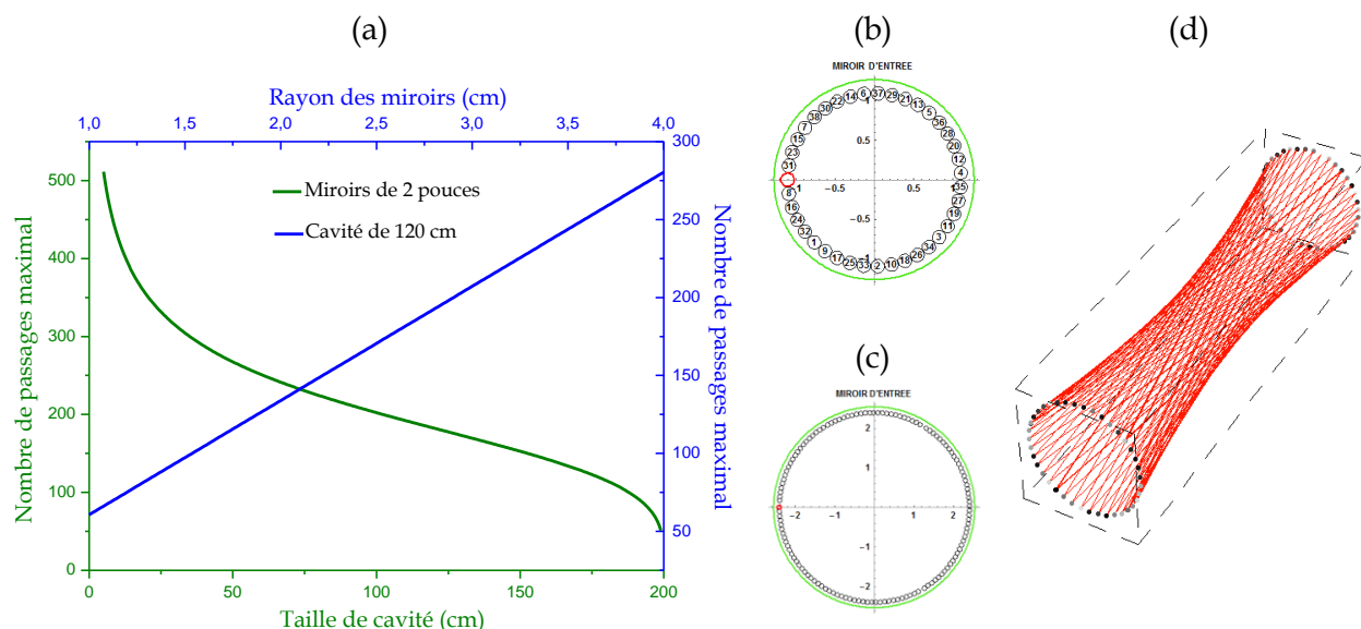
Figure 6.4 : Illustration de la limitation du nombre de passages dans une cellule de Herriott sphérique. Le graphique (a) présente simultanément le nombre maximal de passage de cavité pour (en vert) une taille de miroir donnée dépendamment de la taille de la cavité (donc de la taille des impacts pour \lambda=760 nm et R_{1,2}=1 m) et (en bleu) ce même nombre maximal pour une taille de cavité donnée dépendamment de la taille transverse des miroirs. En (b) et (c) sont représentés des exemples de simulations de nombre maximal de passages pour une cellule de 120 cm avec des miroirs de 1 pouce ( n_{Max}=72 \times 2 ) et des miroirs de 2 pouces pour une cavité de 50,34 cm ( n_{Max}=260 \times 2 ),
