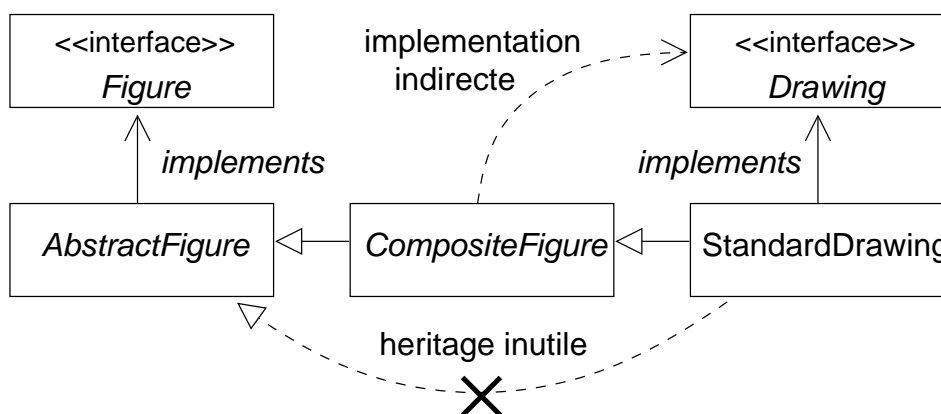
Illustration 7.1 – Hiérarchie de StandardDrawing et réutilisation du motif COMPOSITE dans JHotDraw.
