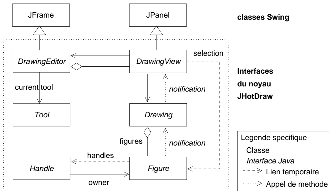
Illustration 4.1 – Schéma synthétique des entités et relations du noyau JHotDraw
