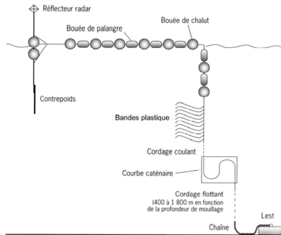
Figure 2-3 : Schéma d'un DCP mi-lourd selon le modèle "océan Indien" (d'après Tessier et al. 2000).
