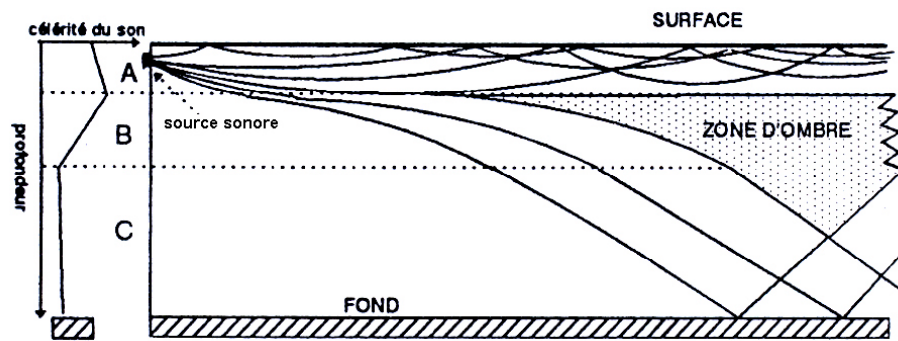
Figure 1-5 : Propagation de rayons sonores dans un milieu présentant une variation de célérité marquée. Une thermocline provoque une forte diminution de la célérité, ce qui a pour effet de créer une zone d'ombre dans laquelle aucune énergie sonore ne pénètre (d'après Diner & Marchand 1995).
