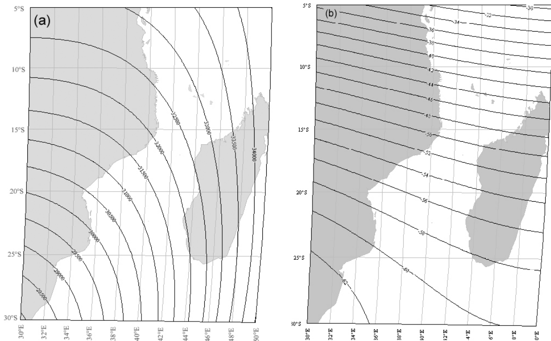
Figure 3-6 : Modélisation du champ magnétique terrestre dans le canal du Mozambique pour l'année 2003. (a) Intensité géomagnétique (par intervalle de 500 nT). (b) Inclinaison géomagnétique (par intervalle de 2°) (source : http://www.ava.fmi.fi/MAGN/igrf/applet.html ).
