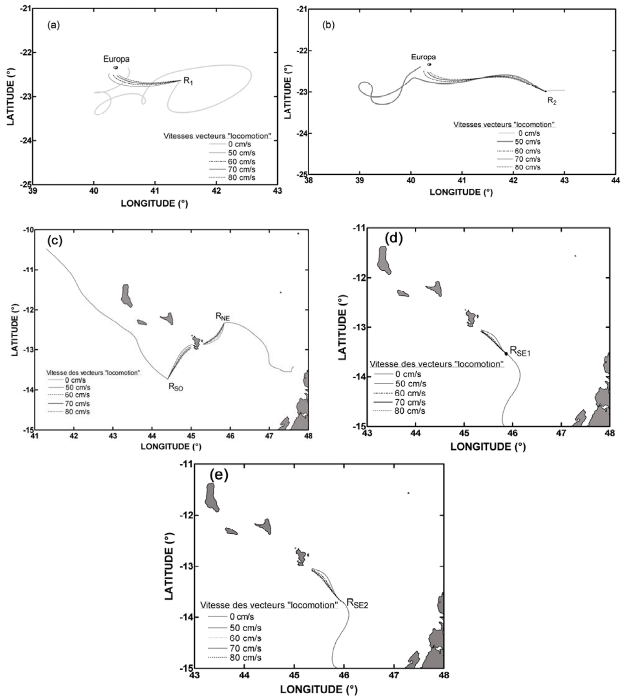
Figure 3-15 : Simulation de trajets de tortues virtuelles, relâchées aux mêmes emplacements et aux mêmes dates que les vraies tortues. Ces tortues virtuelles estiment toutes les heures la direction de leur plage de ponte avec précision mais elles ne sont pas capables de compenser la dérive due au courant. Chaque trajet correspond à une séquence de vecteurs "trajets" calculés en sommant toutes les heures un vecteur "courant" local (estimé à partir des champs de vélocité de surface) et un vecteur "locomotion de vitesse égale à 0, 50, 60, 70 ou 80 cm/s selon la simulation. Les trajets simulés correspondant au troisième lâcher de 2005 (au même site que le second lâcher mais un jour après) sont extrêmement similaires à ceux du second lâcher (fig. e). Ils ne sont, de ce fait, pas représentés.
