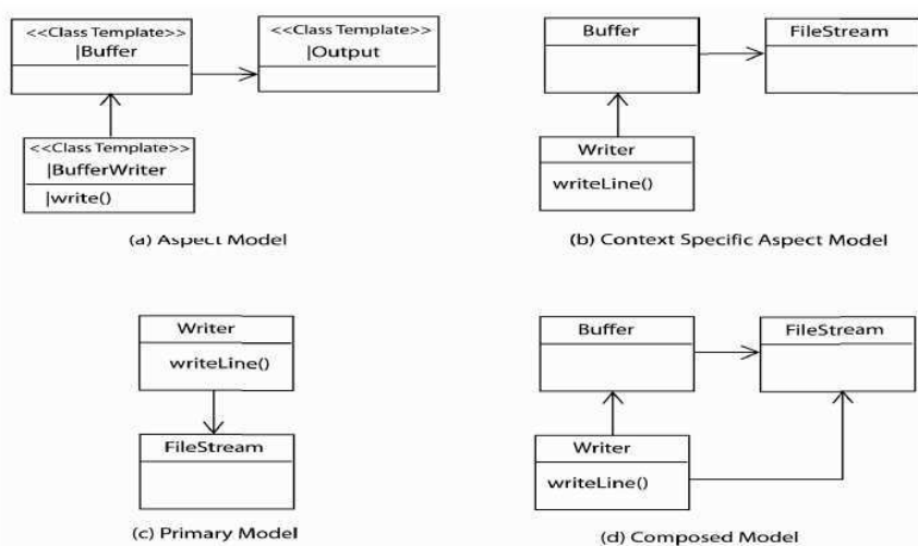
FIG. 3.9 – Exemple de composition [SGS + 04]
