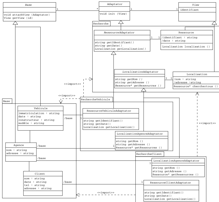
FIG. 11.6 – Introduction du patron Adaptateur
