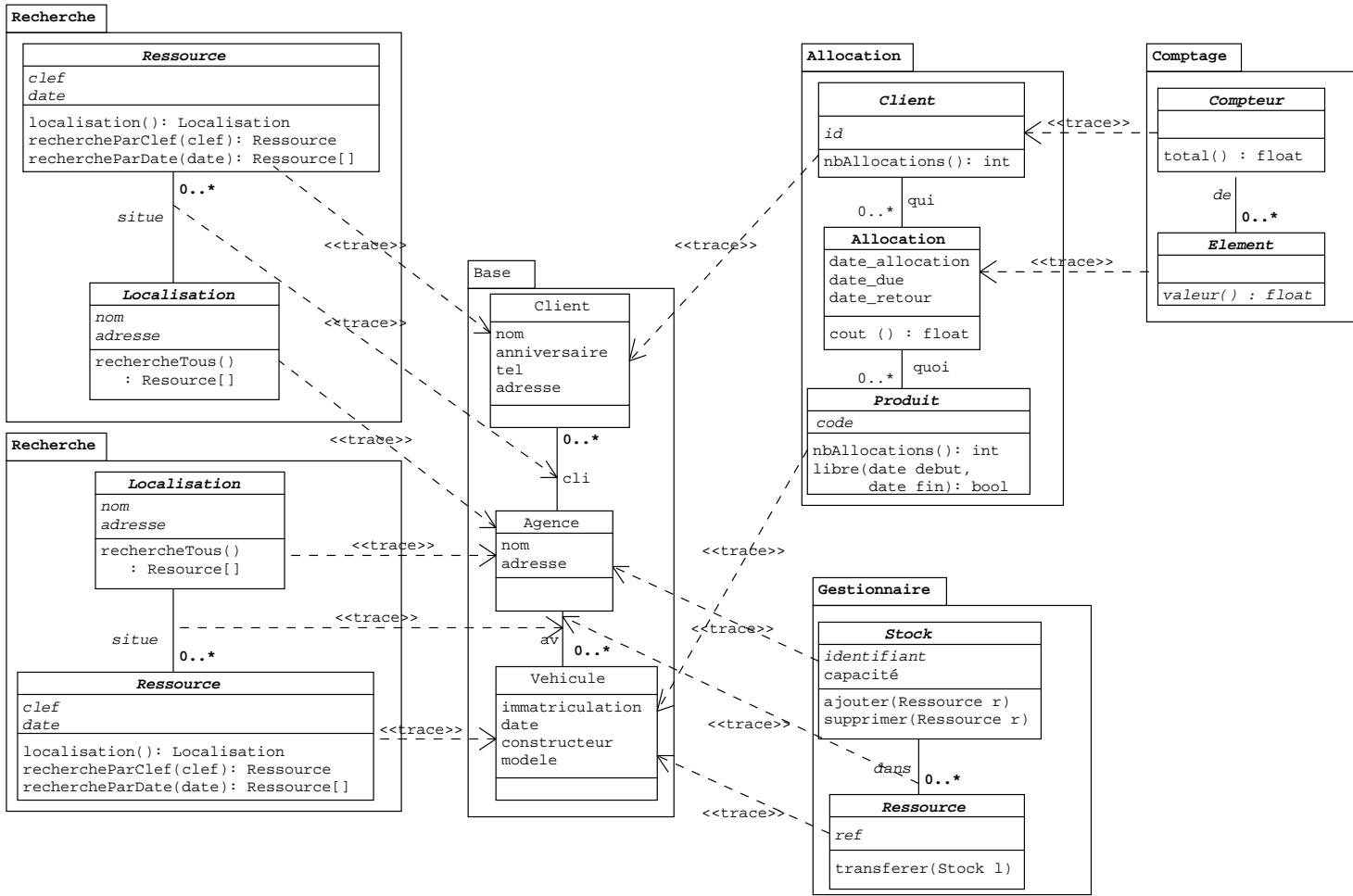
Fig. C.2 – Modèle résultat du système de location de véhicules
