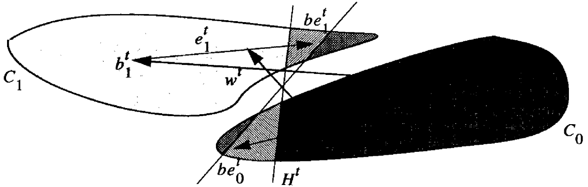
FIG. 5.1: Illustration de la convergence du BCP
