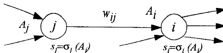
FIG. 3.10: Notations pour la rétropropagation
