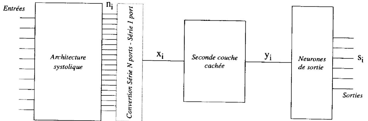
FIG. 5.28: Schéma général
