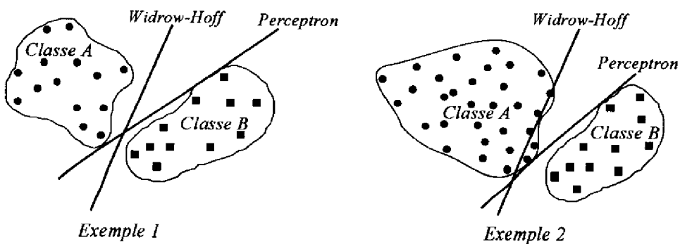
FIG. 3.7: Comparaison des solutions fournies par la règle du Perceptron et la règle de Widrow-Hoff
