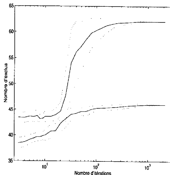
FIG. 5.12: Nombre d'exemples exclus par BCP Max en fonction du nombre d'itérations pour des distributions gaussiennes qui se chevauchent en dimension 2.
