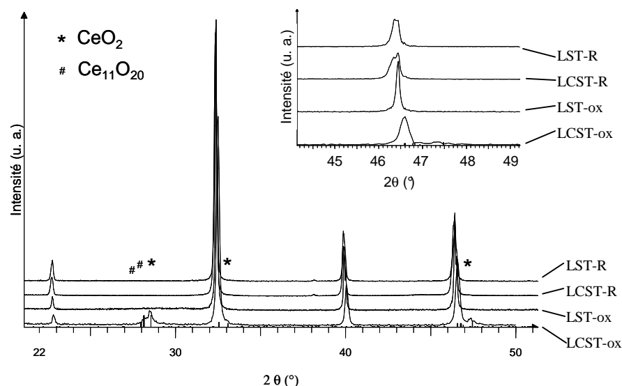
Figure II.21 : diagrammes de DRX sur poudre des composés LCST-ox, LST-ox, LCST-R, LST-R (de bas en haut). Le zoom a été réalisé en soustrayant la contribution de la raie K\alpha_2 de Cu. Le zoom témoigne du dédoublement des pics lié à l'abaissement de la symétrie cubique de la pérovskite idéale des composés LCST-R et LST-R.
