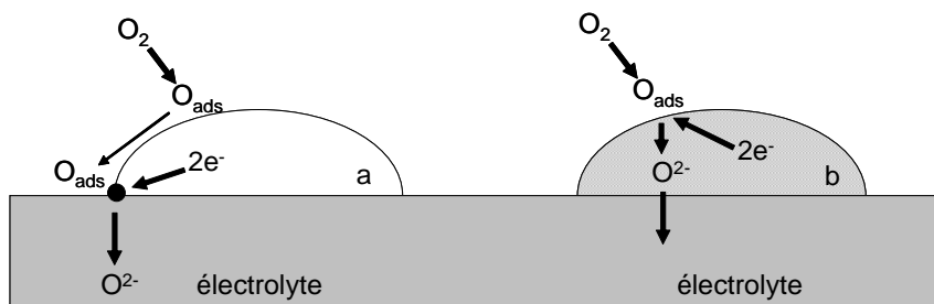
Figure I.4 : illustration des mécanismes de diffusion de l'oxygène en surface (a) ou en volume (b) du matériau d'électrode. Dans le cas d'un conducteur électronique, seul le cas a) pourra être envisagé, tandis que dans le cas d'un conducteur mixte, les deux cas seront potentiellement réalisables.
