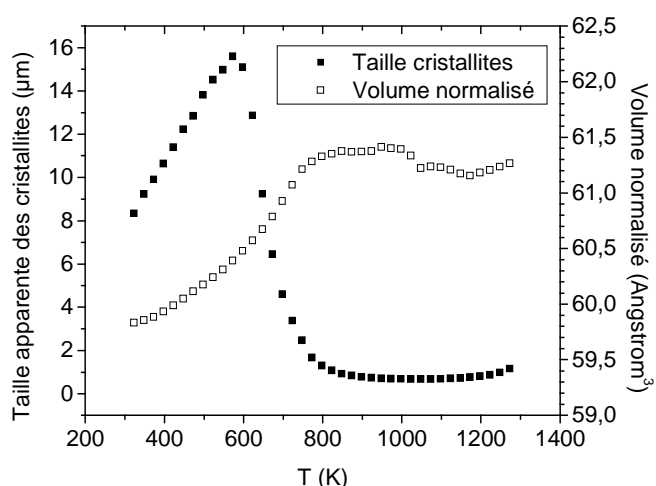
Figure II.28 : évolution combinée en fonction de la température de la taille apparente des cristallites (taille du domaine diffractant) et du volume normalisé de la maille orthorhombique Immm 5.8x5.8x7.8 de LCST-R lors de la réoxydation sous air. Ce résultat a été obtenu par affinement cyclique des données de DRX-HT enregistrés lors de la montée en température sous air de l'ambiante à 1273K par pas de 25K.
