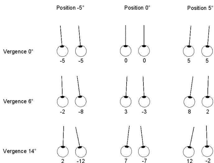
Figure 6.9. Schématisation des positions horizontales des yeux ; calcul de la position moyenne des yeux et de l'angle de la vergence. Sous chaque œil est inscrite sa position horizontale en degré. Une même colonne correspond à une même position moyenne, cyclopéenne, une même ligne à un même angle de vergence.
