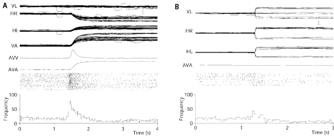
Figure 5.2. Réponse d'un neurone de vergence dans le cortex préarcuate. Les décharges pour plusieurs essais ( raster plots ) sont alignées sur le début du mouvement oculaire. Les histogrammes temporels péri-stimulus représentent la moyenne. A : réponse neurale pendant une vergence. B : réponse neurale pendant une saccade. AVA, angle de vergence moyen. AVV, vitesse de vergence moyenne. HL, position horizontale de l'œil gauche. HR, position horizontale de l'œil droit. TARG, position de la cible. VA, angle de vergence. VL, position verticale de l'œil gauche. Source : Gamlin et Yoon (2000).
