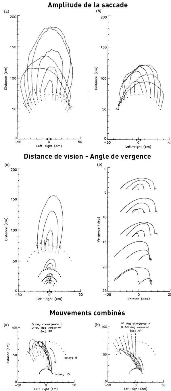
Figure 3.4. Trajectoires des saccades et des mouvements combinés saccade-vergence, projetées dans le plan horizontal. En haut : trajectoires de saccades vers la droite (a) ou vers la gauche (b) sur un cercle d'isovergence 5°. Au milieu : trajectoires de saccades vers la droite en coordonnées métriques sur différents cercles d'isovergence (a) ; les mêmes saccades sont ensuite représentées en coordonnées angulaires (b). En bas : trajectoires de saccades vers la droite associées à une convergence de 10° (a) et de saccades vers la gauche associées à une divergence de 10° (b). Adapté de Collewyn et al. (1997).
