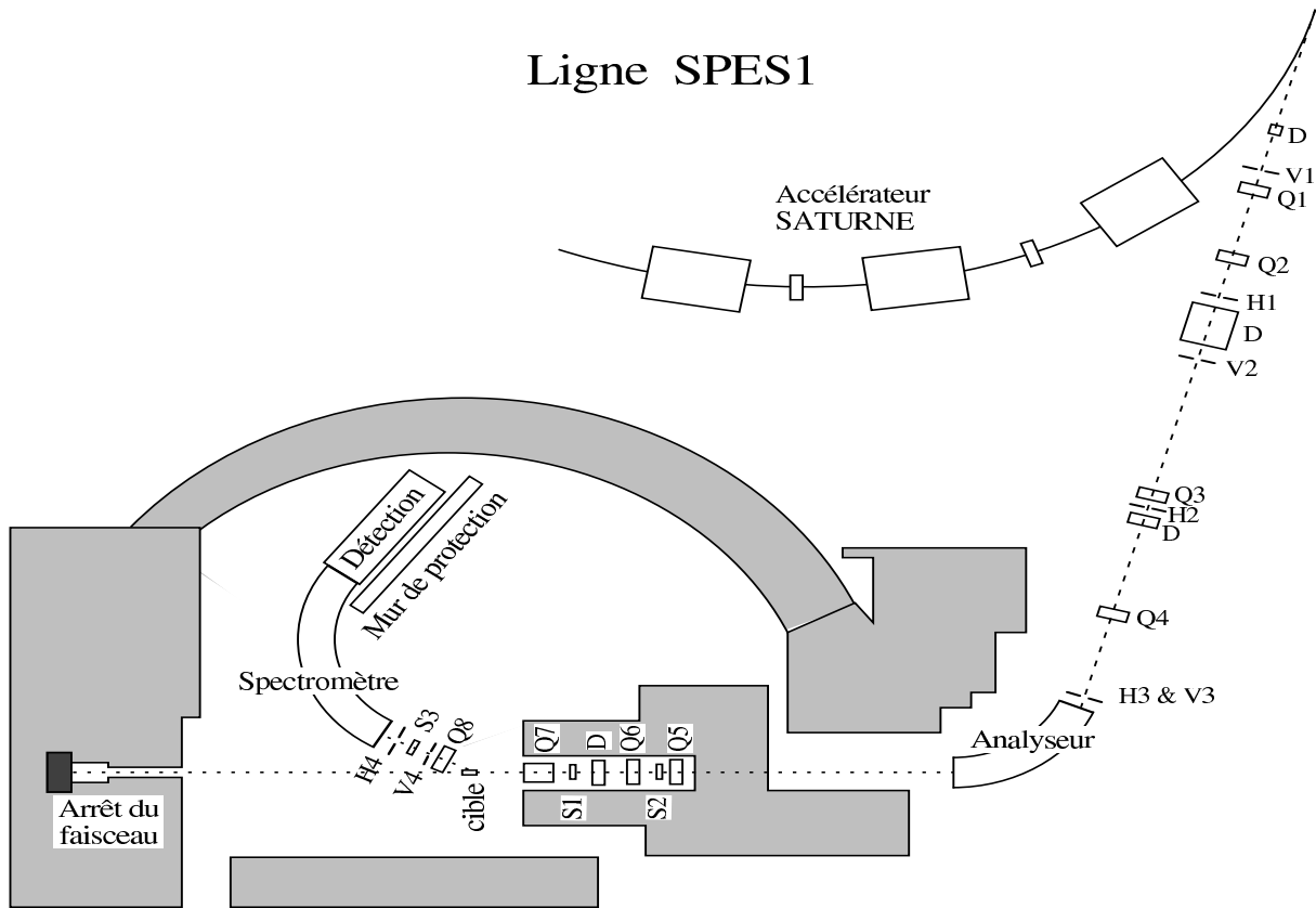
FIG. 3.3 – Spectromètre SPES1.
