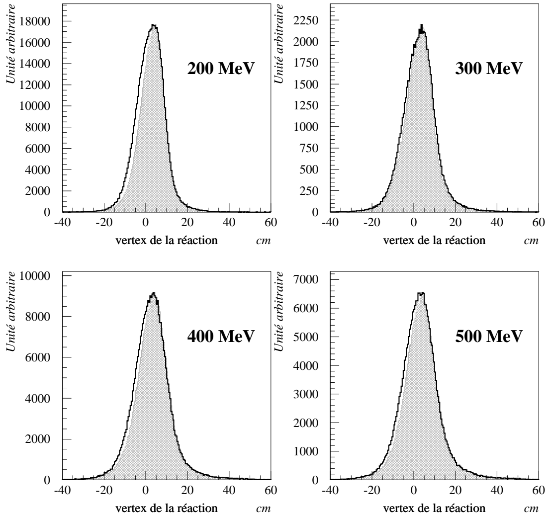
FIG. 3.19 – Vertex de la réaction {}^1\text{H}(\vec{d}, 2\text{p})\text{n} calculé avec les données expérimentales (grisé) et simulées (ligne sombre) à quatre énergies deuton.
