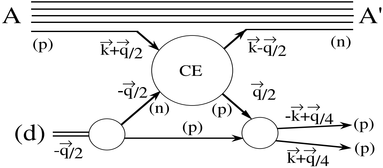
FIG. 2.1 – Diagramme de l'approximation d'impulsion pour dA \rightarrow (pp)A' , montrant les états initial et final dans le repère de Breit du deuteron.
