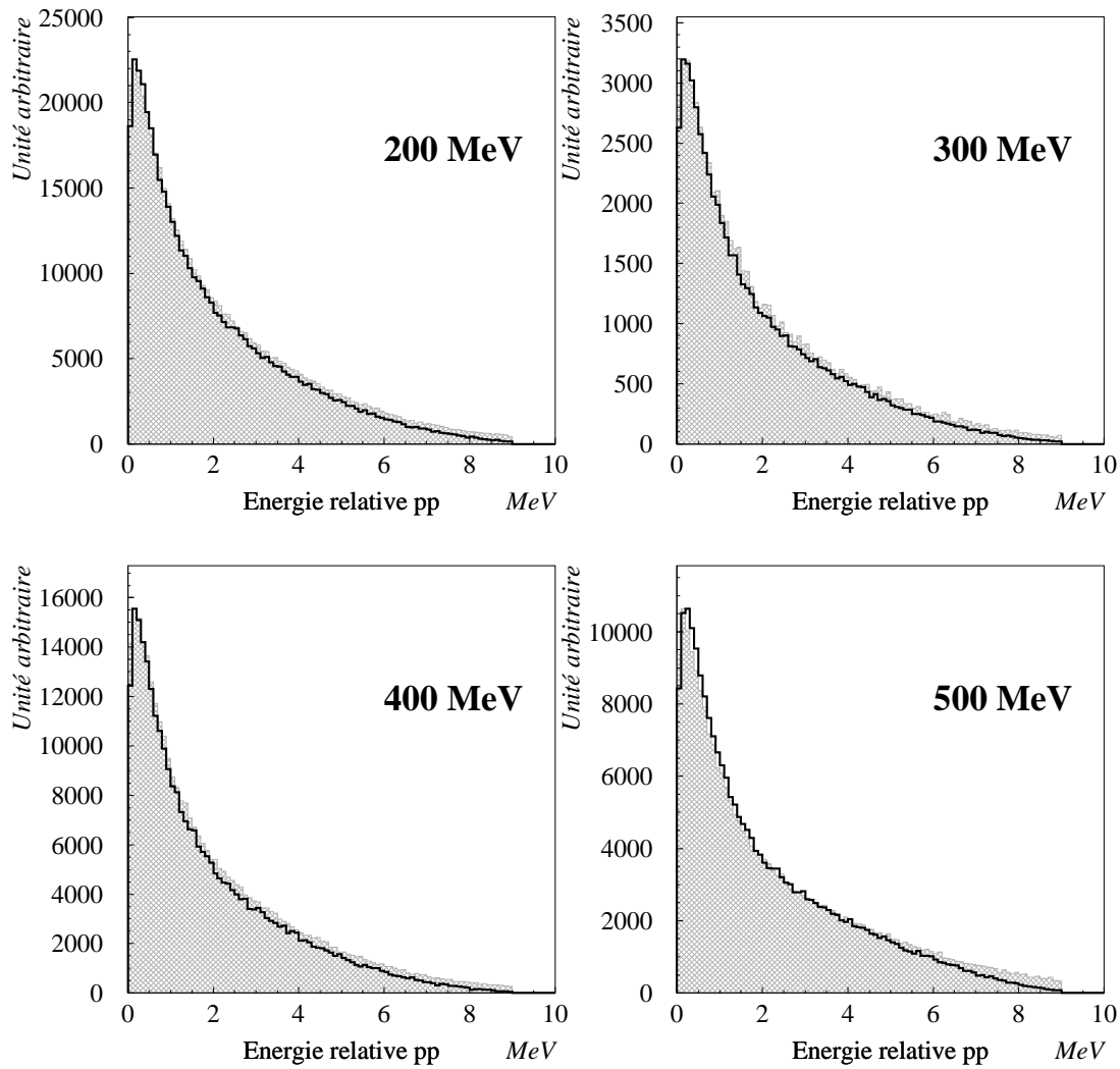
FIG. 3.24 – Energie relative de la réaction {}^1\text{H}(\vec{d},2\text{p})\text{n} calculée avec les données expérimentales (grisé) et simulées (ligne sombre) à quatre énergies deuton.
