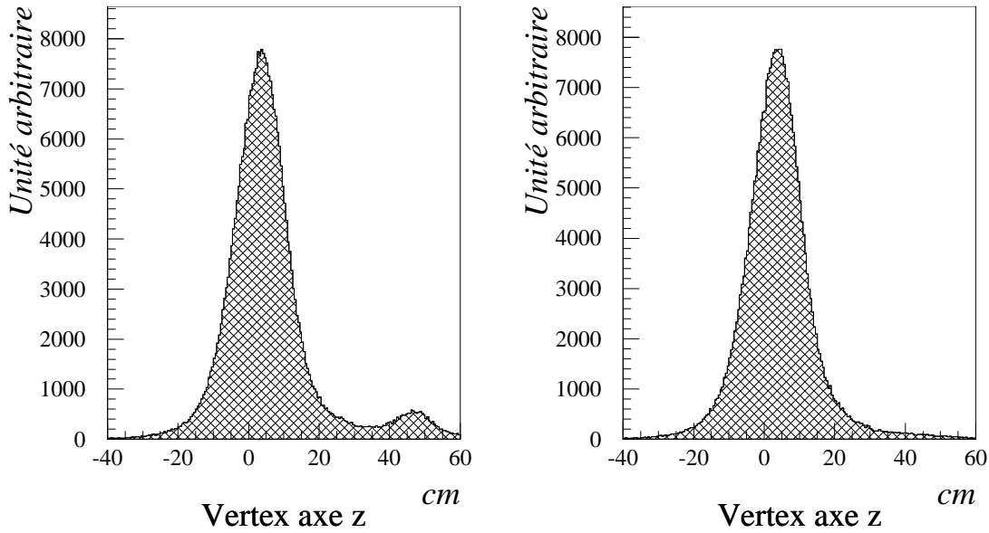
FIG. 3.18 – Vertex de la réaction {}^1\text{H}(\vec{d},2\text{p})\text{n} reconstitué avant (figure de gauche) et après (figure de droite) les coupures dues à la levée de l’ambiguïté pour une énergie cinétique deuton de 400 MeV.
