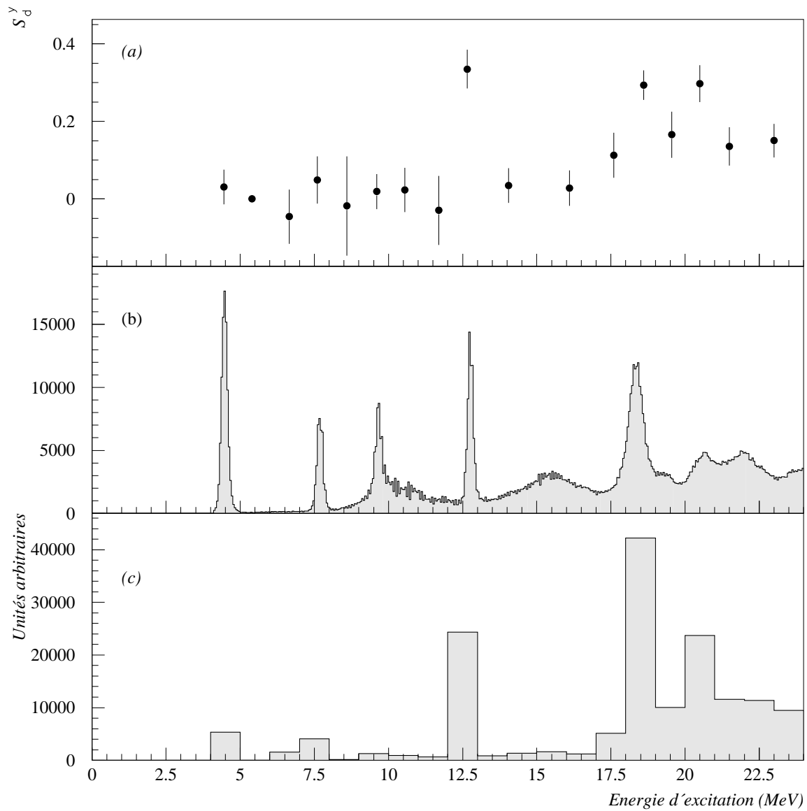
FIG. 4.1 – Résultats de l'expérience sur le ^{12}\text{C} à 4^\circ dans le laboratoire en fonction de l'énergie d'excitation. Les taux de comptage sont représentés pour des intervalles de 100 KeV (b). En (c) est tracé, pour des intervalles de 500 KeV, le produit de la section efficace et de la signature S_d^y (a).
