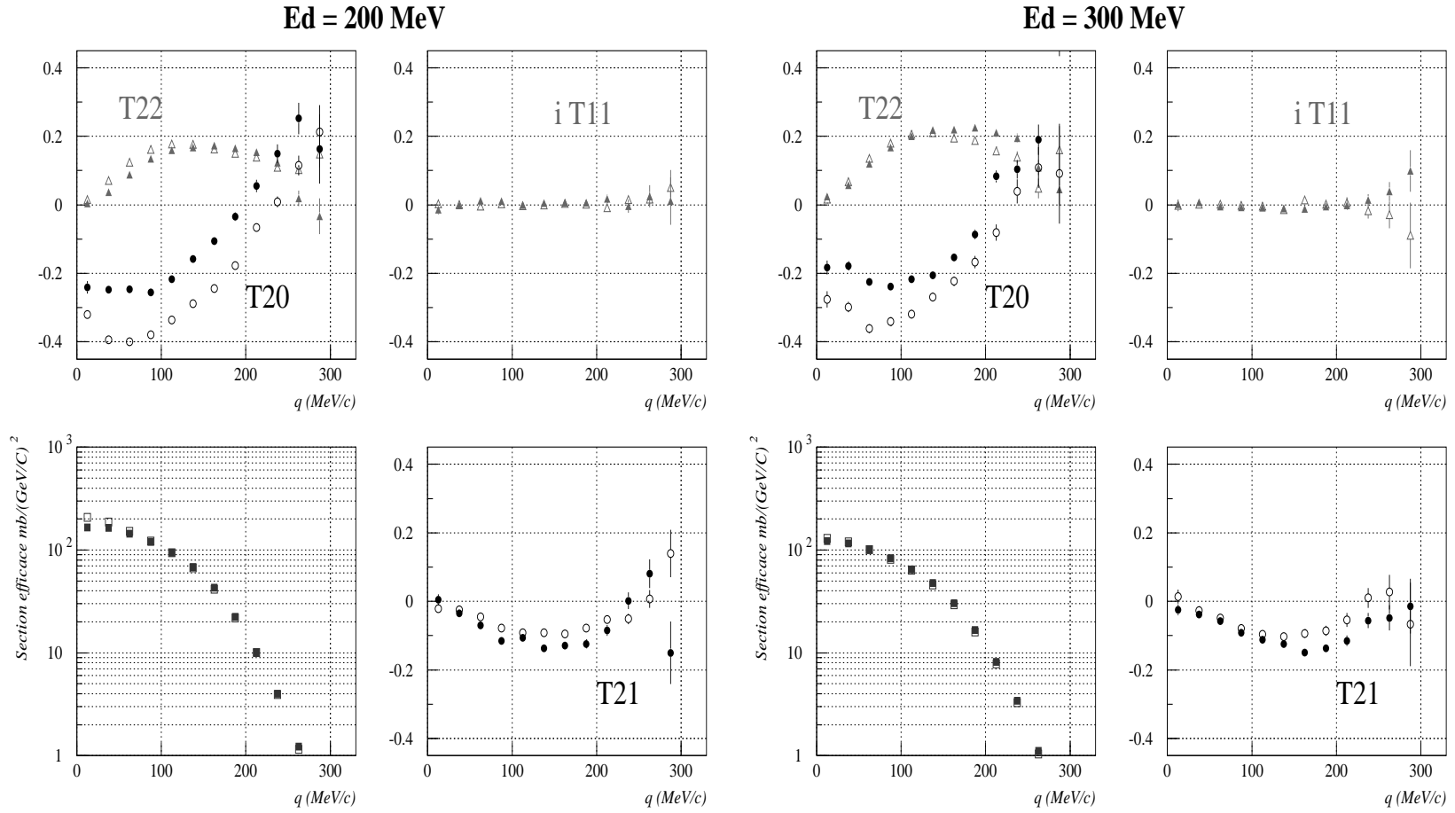
FIG. 3.27 – Pouvoirs d'analyse et section efficace de la réaction {}^1\text{H}(\vec{d}, 2\text{p})\text{n} à 200 et 300 MeV, pour une coupure en énergie relative de 5 MeV.
