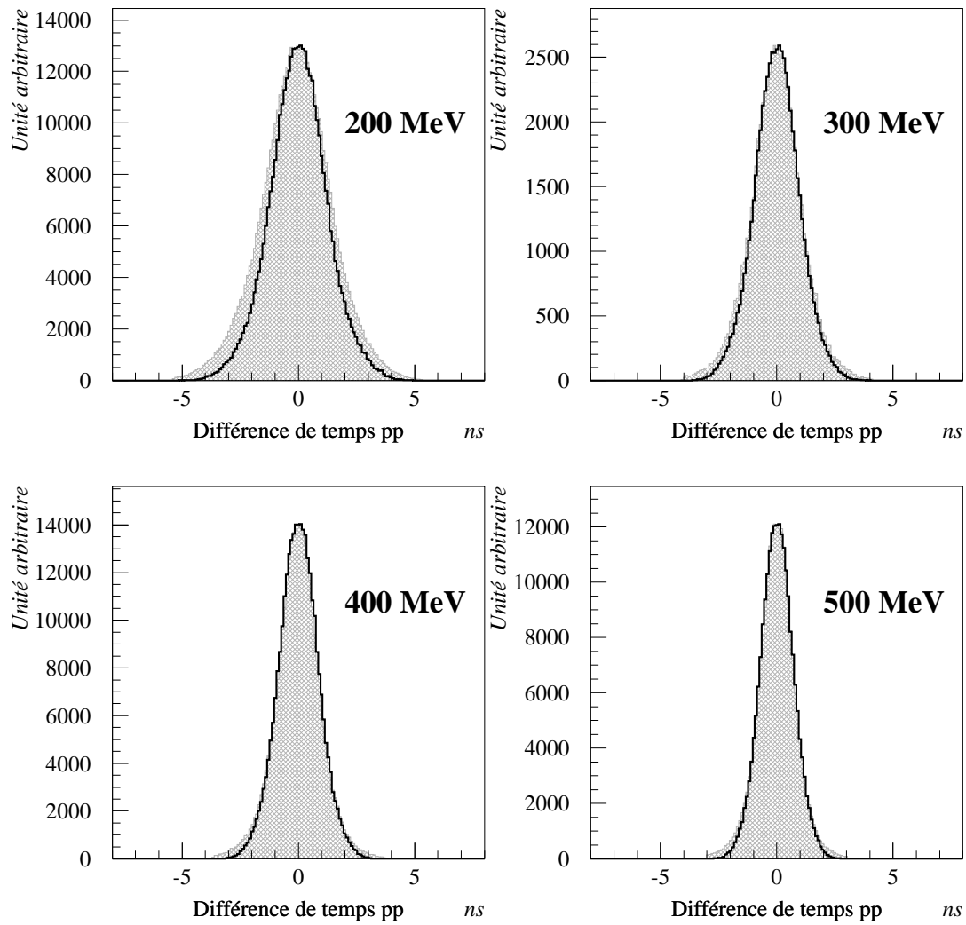
FIG. 3.16 – Différence de temps de vol dans le grand hodoscope entre les deux protons d'échange de charge pour les données expérimentales (grisé) et simulées (ligne sombre) à quatre énergies deuteron.
