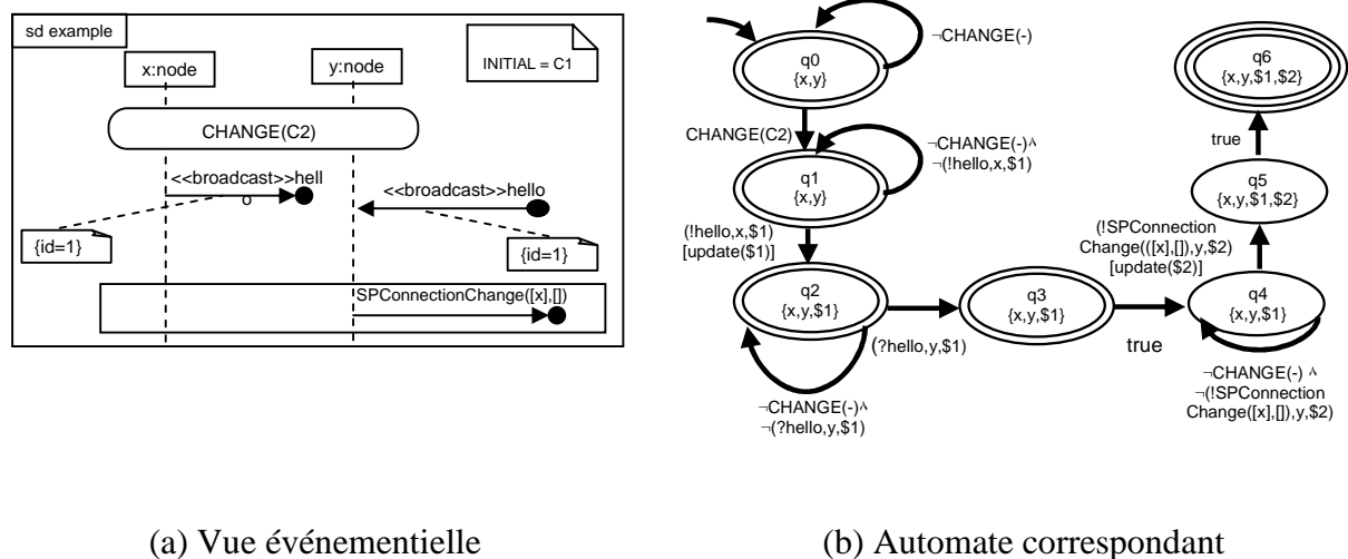
Figure 27. Interprétation de la vue événementielle d'un scénario TERMOS
