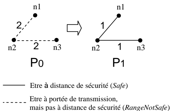
Figure 52. Vue spatiale du scénario de fusions concurrentes
