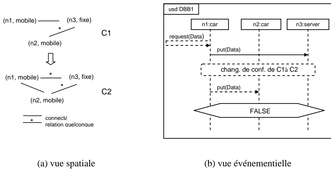
Figure 23. Exemple de scénario d'exigence de la boîte noire
